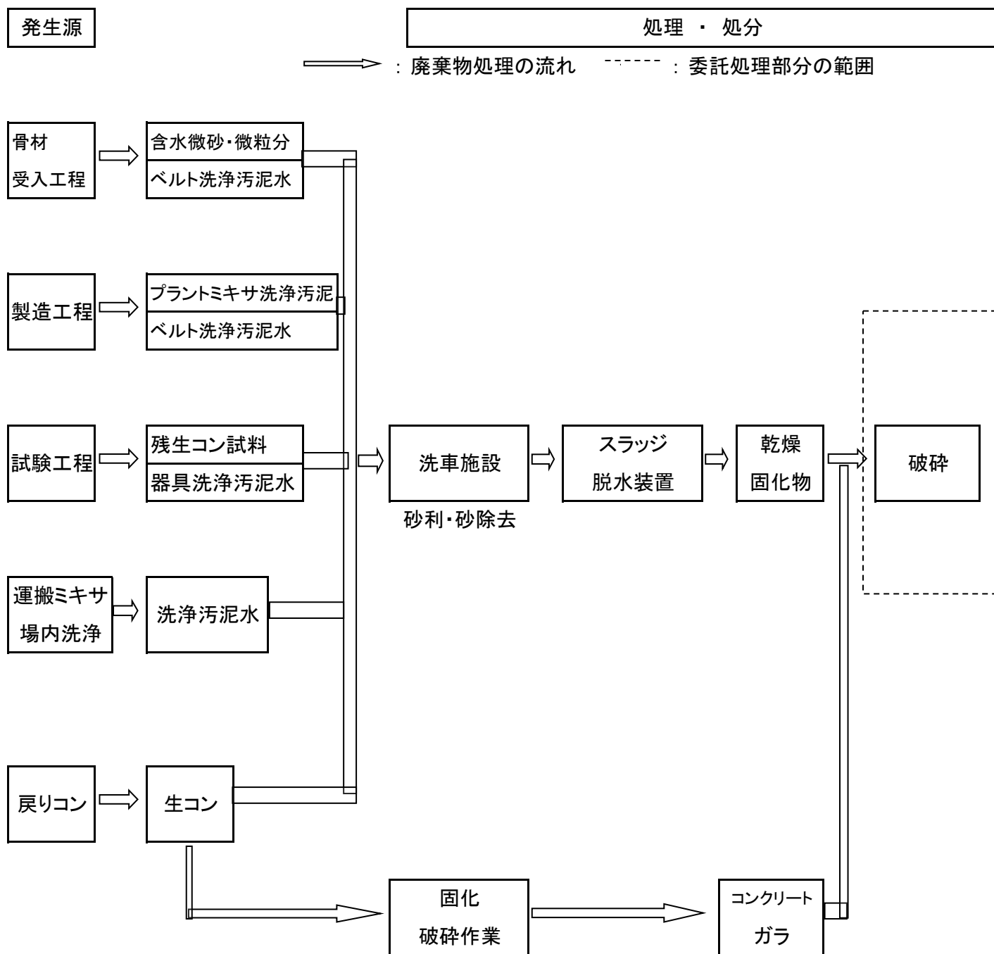
別紙1 廃棄物処理フロー図
