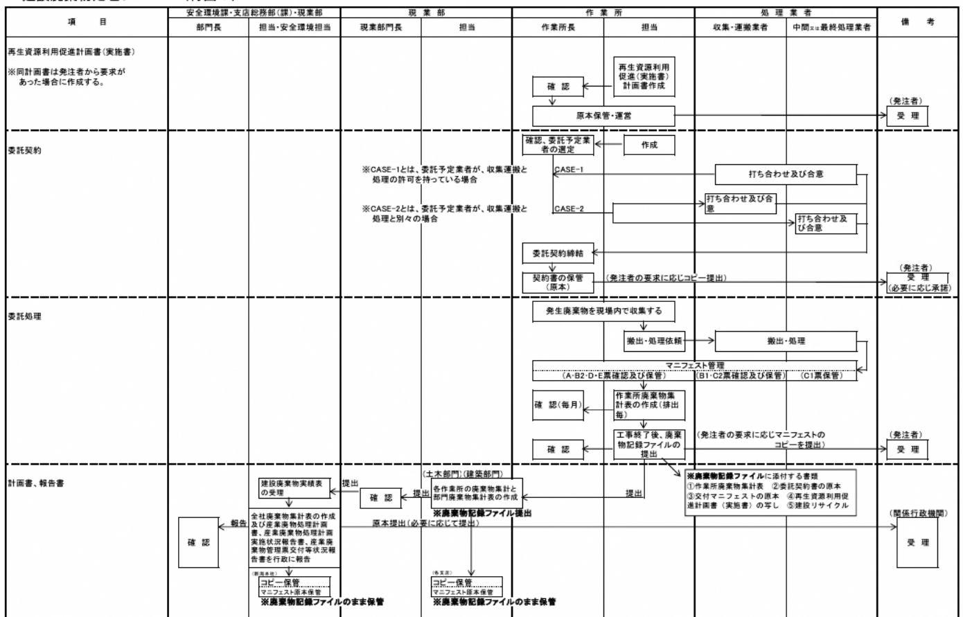
建設廃棄物処理フロー (付図1)
