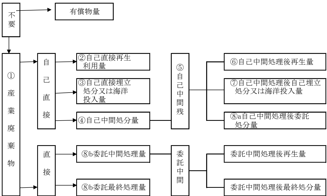
(産業廃棄物処理フロー図)
