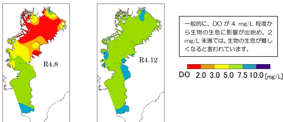
令和4年度における東京湾の下層 DO（溶存酸素量）の平面分布
