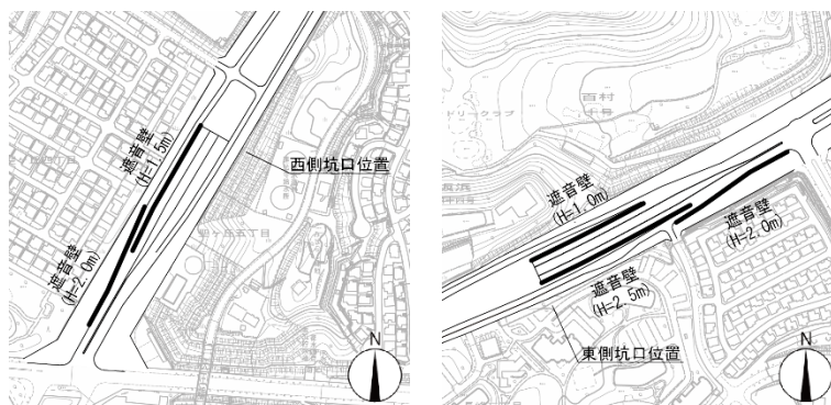
図 5.1.3-3 トンネル取付部の遮音壁設置位置（特例環境配慮書資料編 74 ページ）
