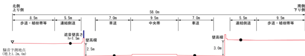
図 5.1.3-1 騒音予測地点断面図（西側坑口部 聖ヶ丘四丁目付近）
