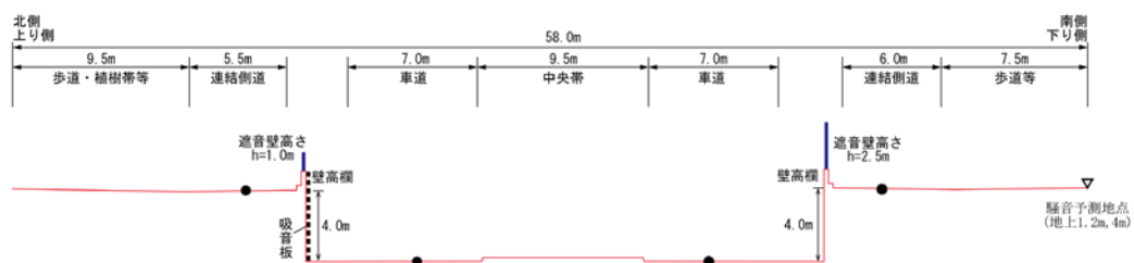
図 5.1.3-2 騒音予測地点断面図（東側坑口部 長峰三丁目付近）
