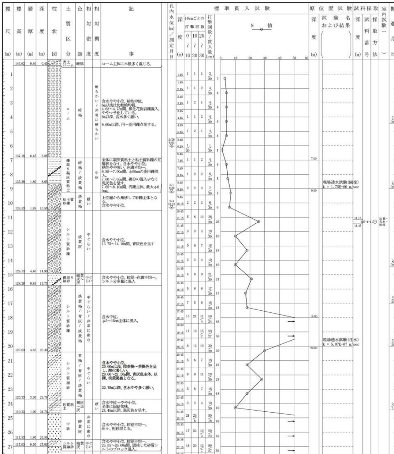
図 5.1-2(1) 柱状図(B-1①)
