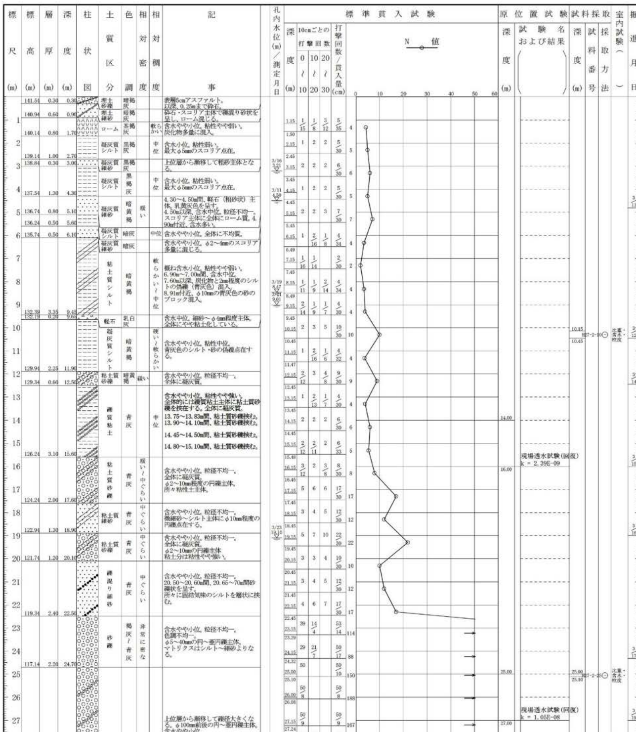
図 5.1-2(3) 柱状図(B-2①)
