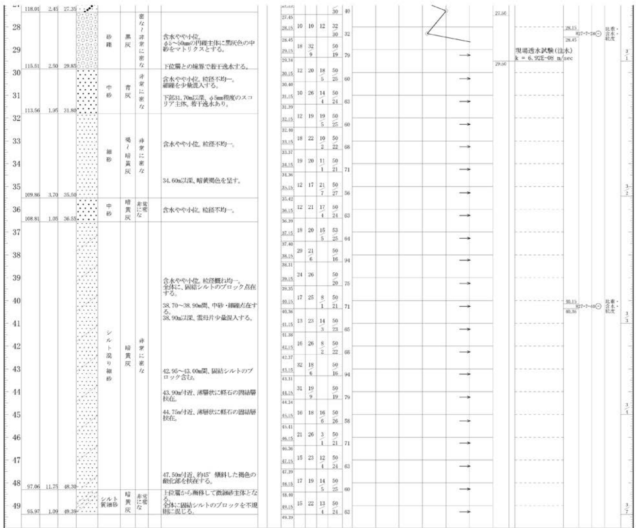
図 5.1-2(14) 柱状図(B-7②)
