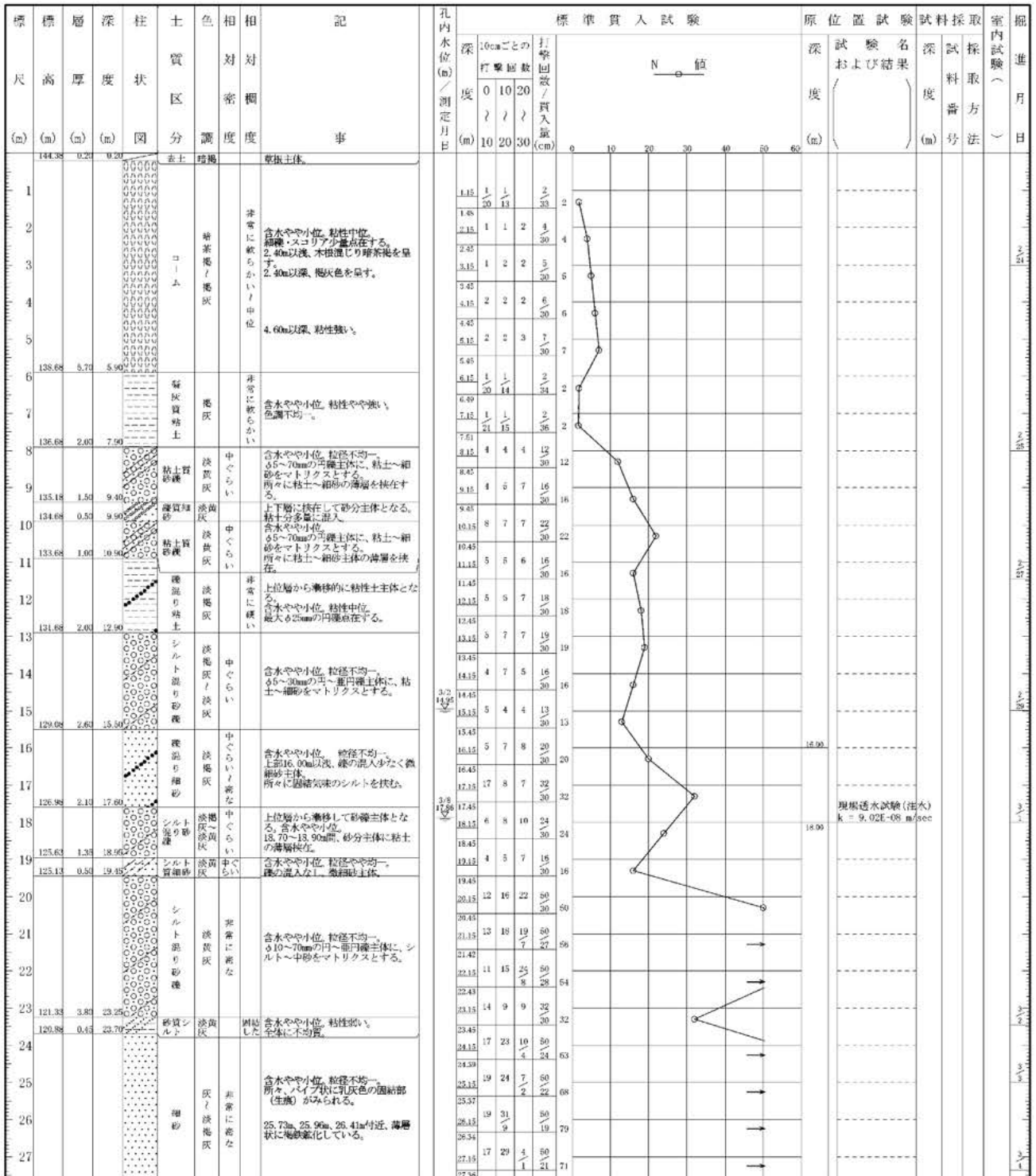
図 5.1-2(5) 柱状図(B-3①)
