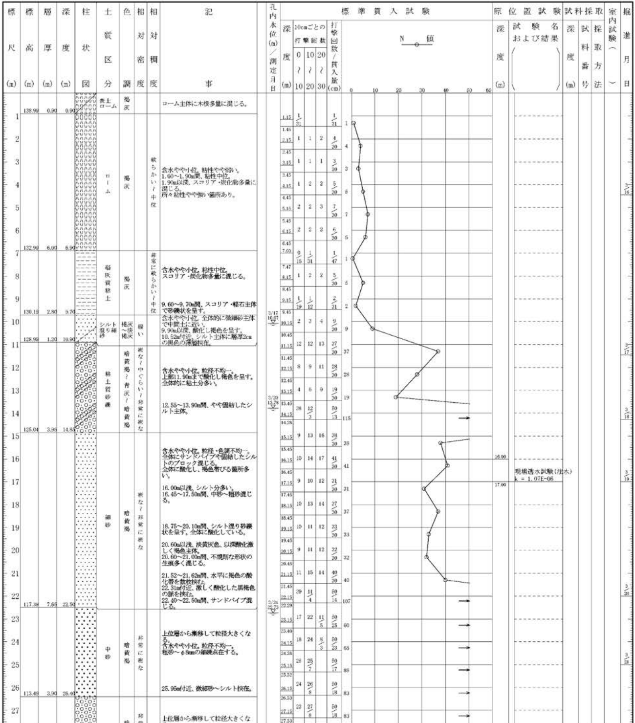
図 5.1-2(7) 柱状図(B-4①)
