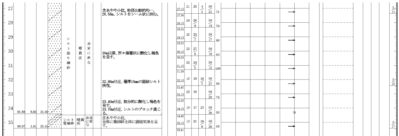
図 5.1-2(10) 柱状図(B-5②)
