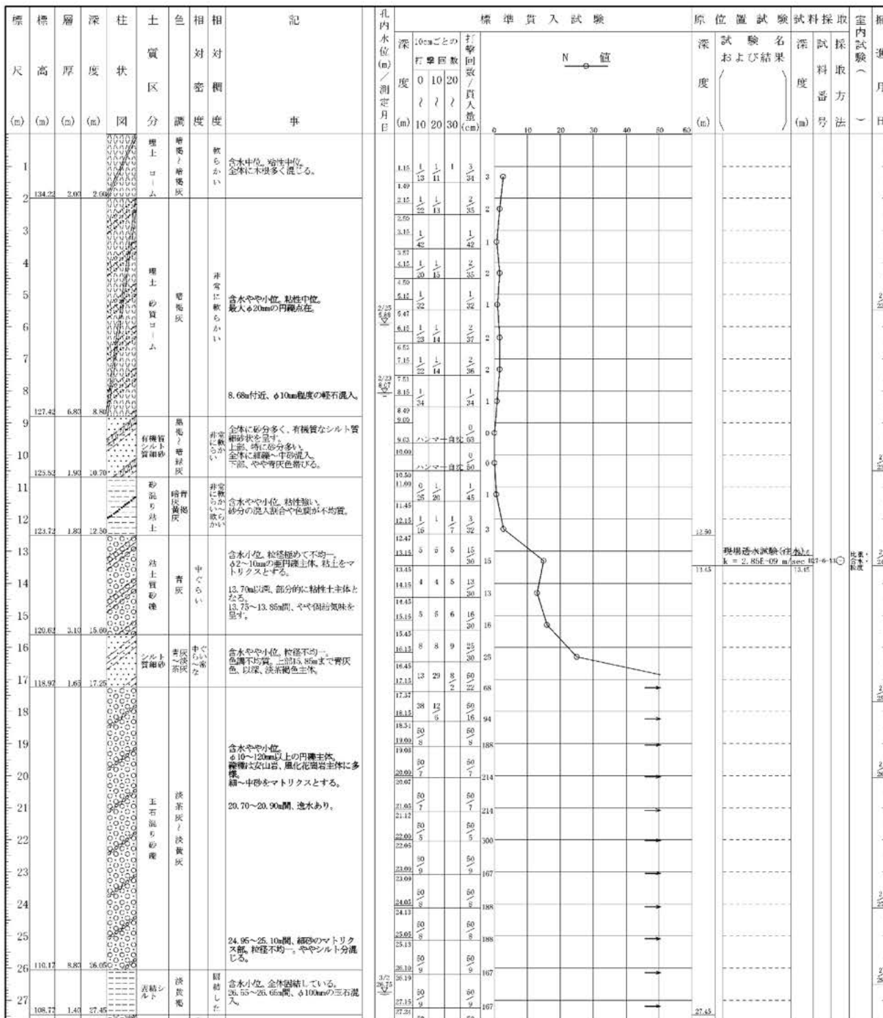
図 5.1-2(11) 柱状図(B-6①)
