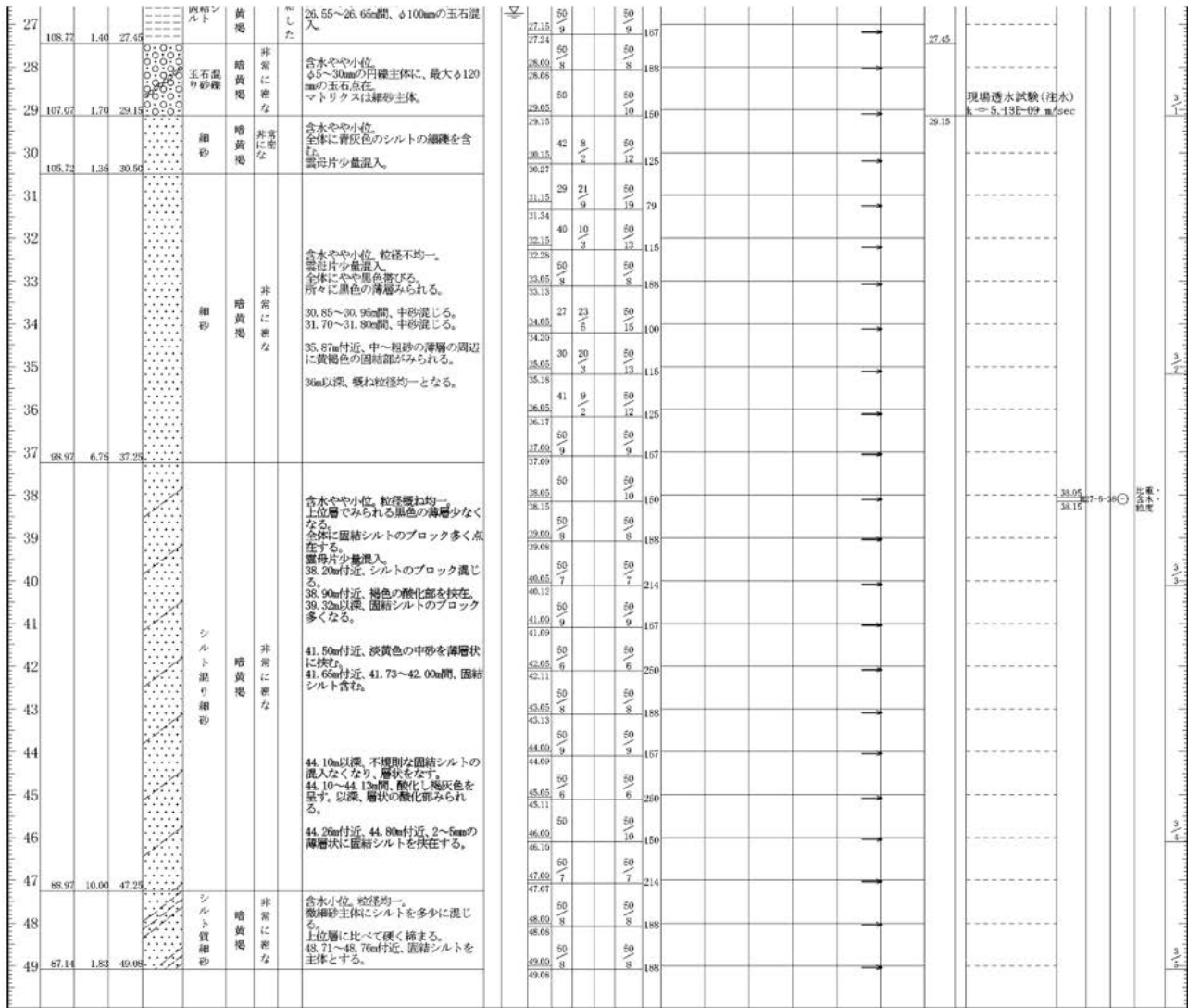
図 5.1-2(12) 柱状図(B-6②)
