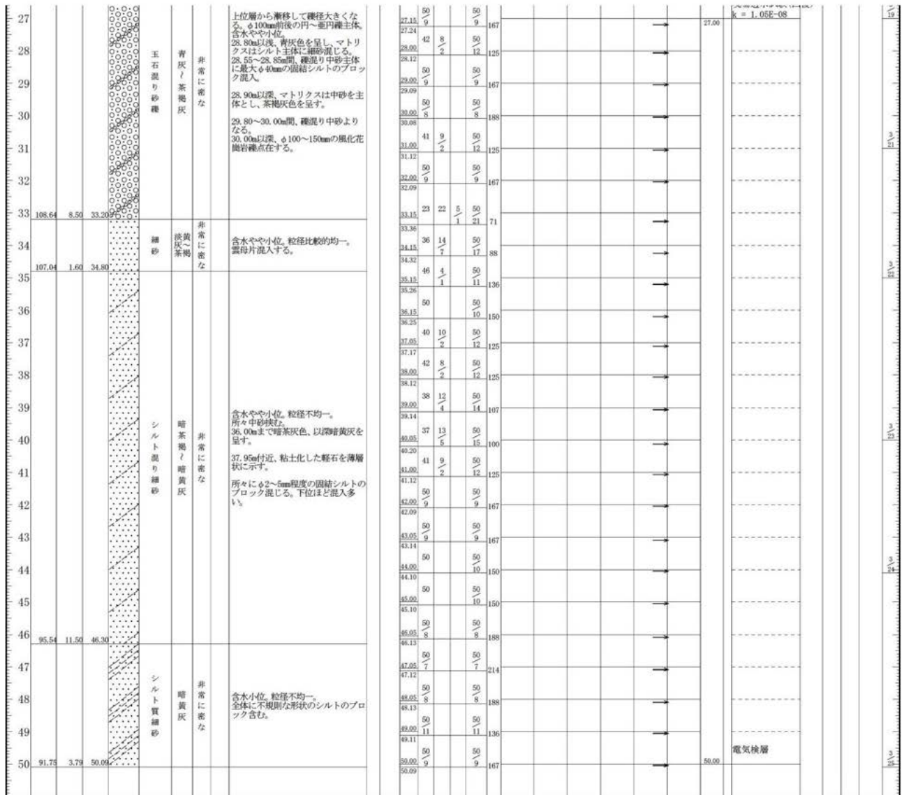
図 5.1-2(4) 柱状図(B-2②)
