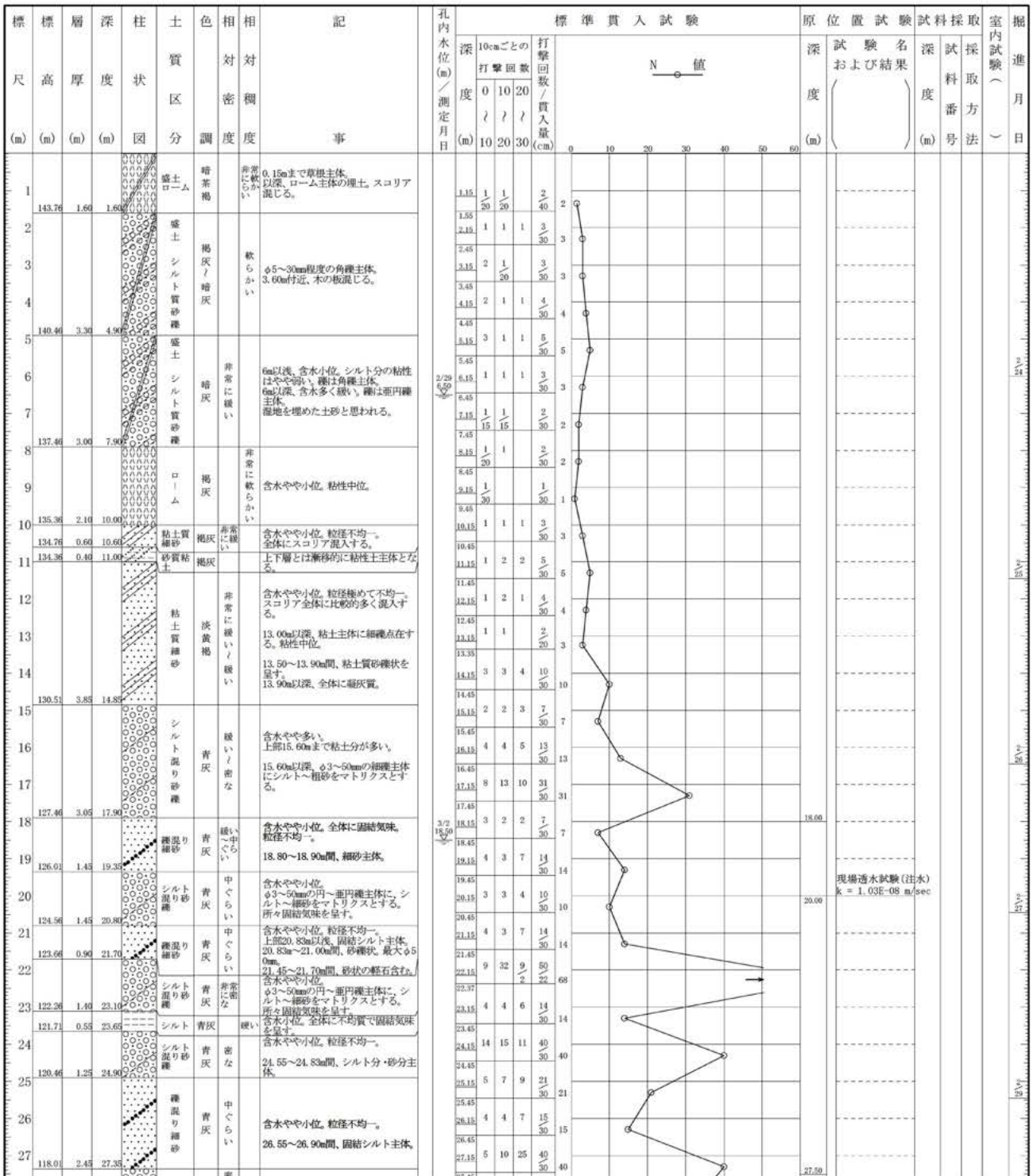
図 5.1-2(13) 柱状図(B-7①)
