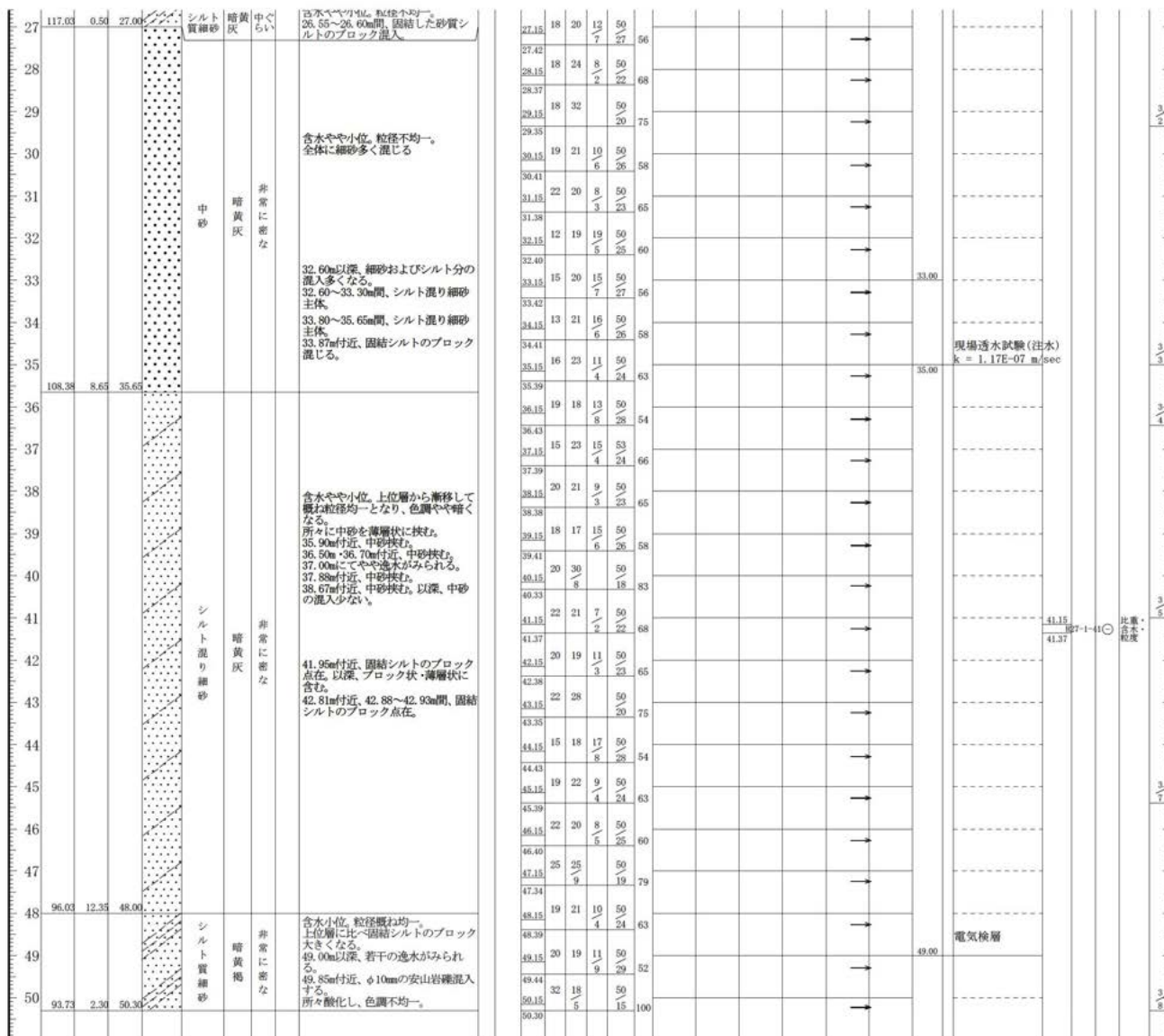
図 5.1-2 (2) 柱状図(B-1②)
