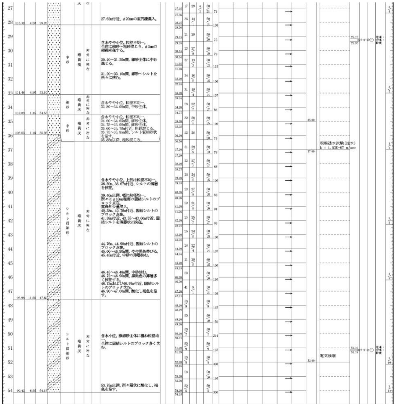
図 5.1-2 (6) 柱状図(B-3②)
