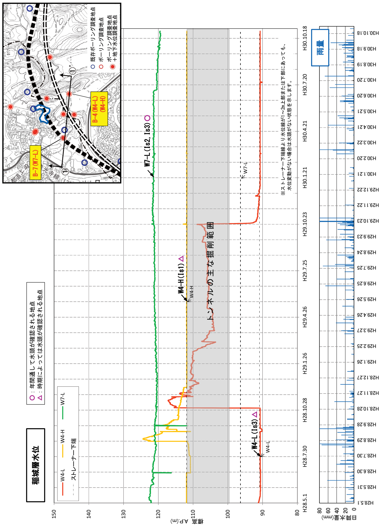
図 6.1-2(2) 地下水位の変動状況（稲城層①）
