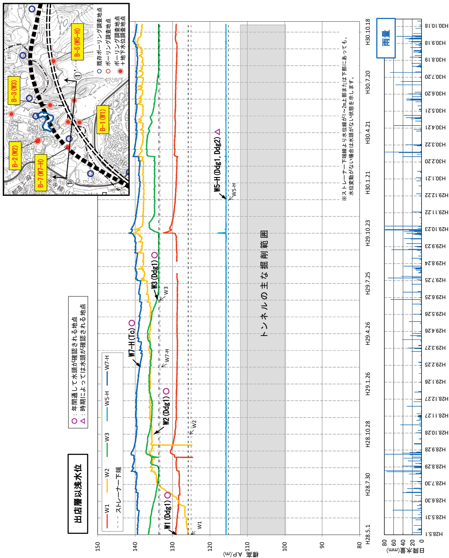
図 6.1-2(1) 地下水位の変動状況（出店層以浅）
