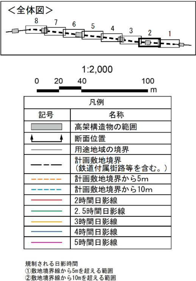
図 8.3.2-2(2) 等時間日影図
