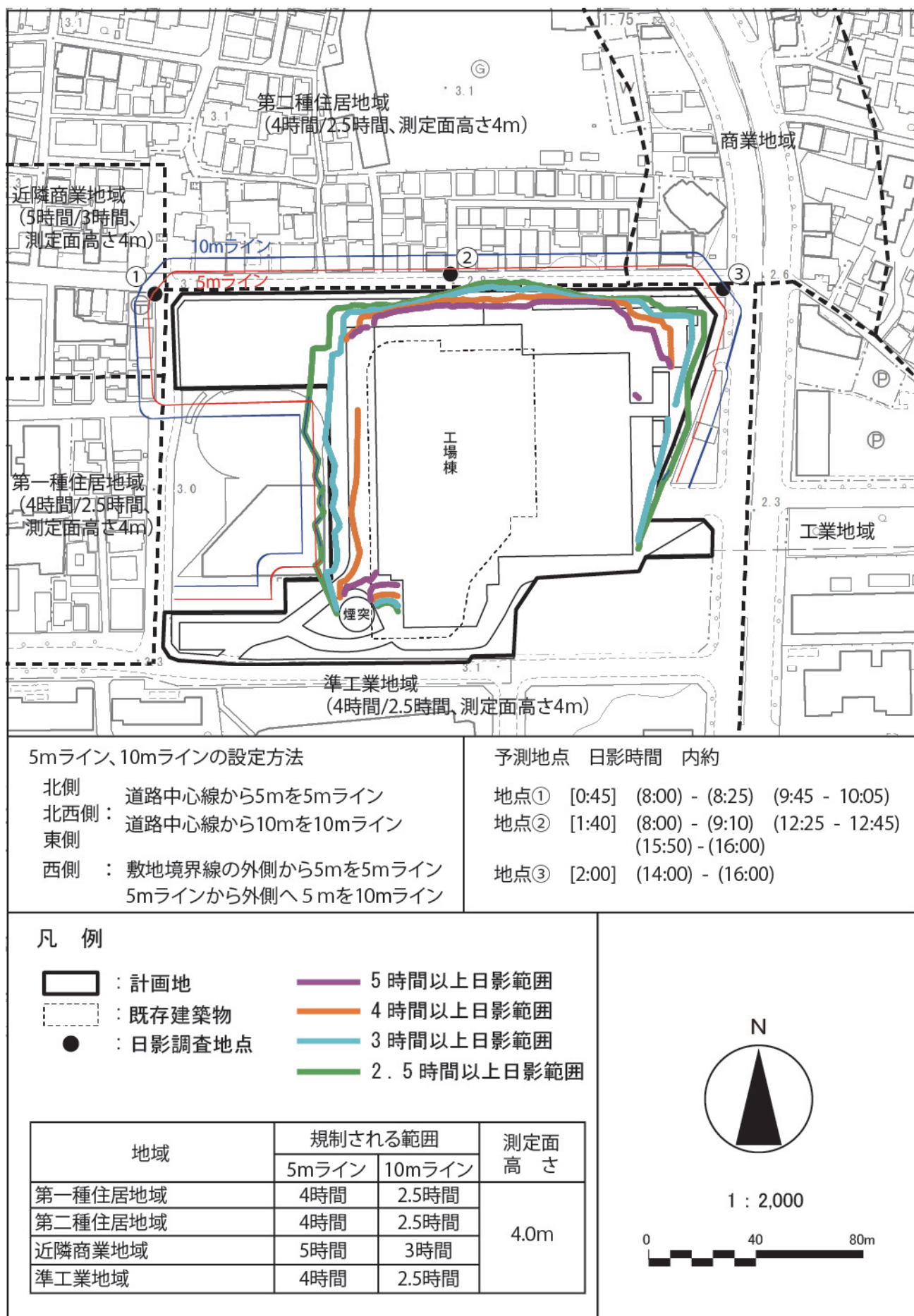
図 8.7-9(2) 計画建築物等（煙突を含む）による等時間日影図
