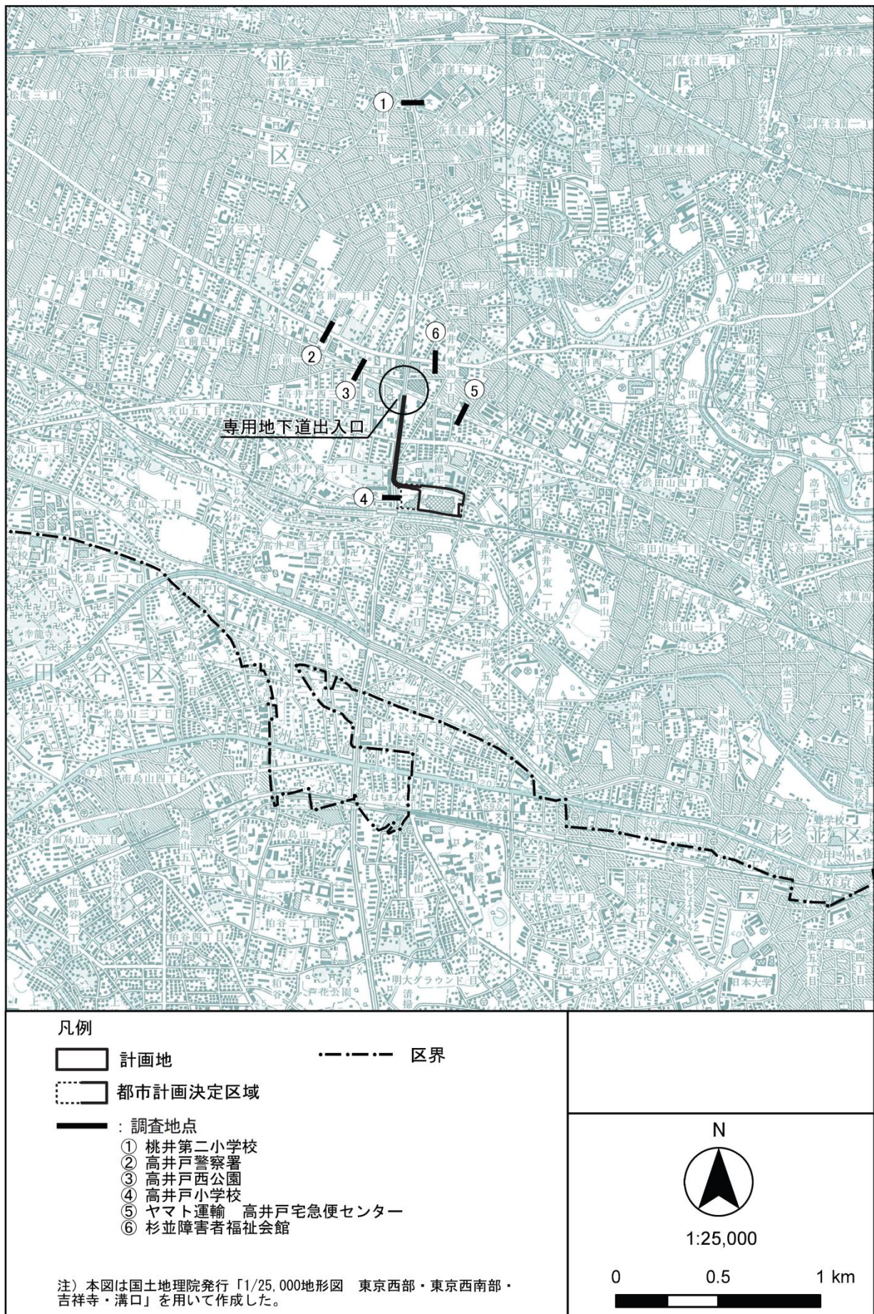
図 7.1-3 清掃車両の台数及び断面交通量の調査地点
