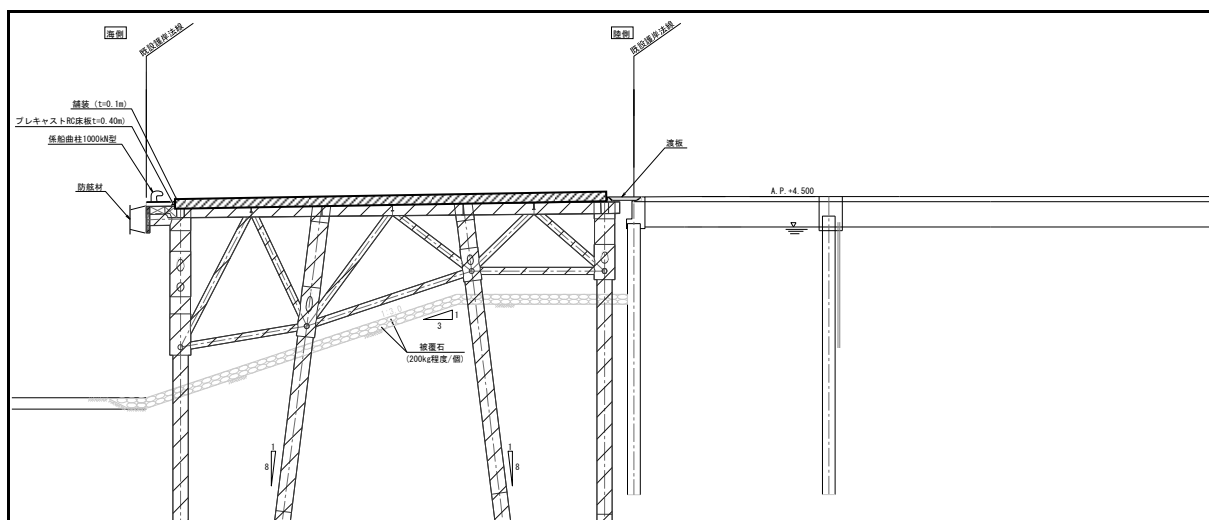
図1-1(1) 工事の実施位置（栈橋式岸壁工）
