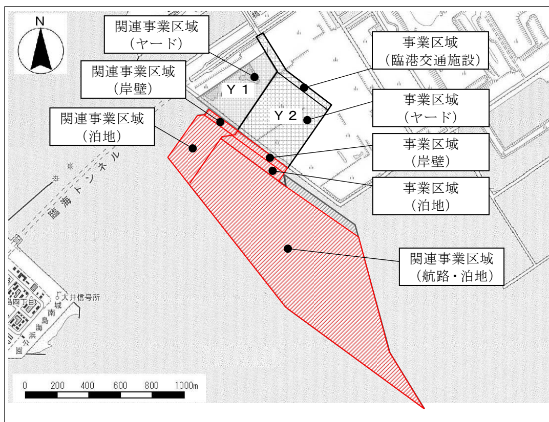
図1-1(3) 工事の実施位置（浚渫工事）
