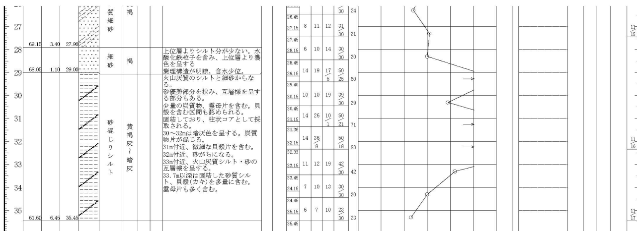
図 8.5-1 (3) ボーリング柱状図 (No. 2) (2)
