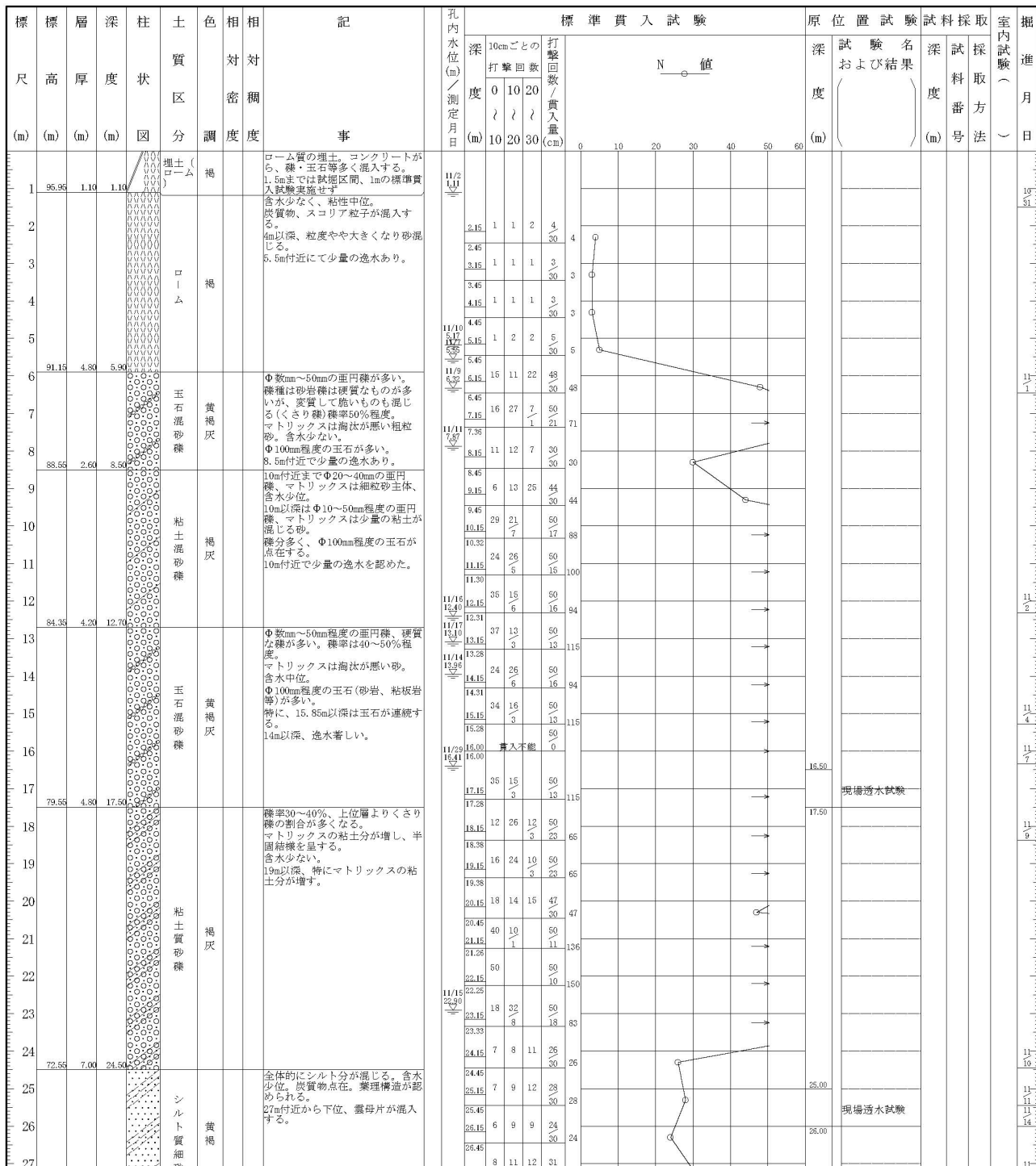
図 8.5-1 (2) ボーリング柱状図 (No. 2) (1)
