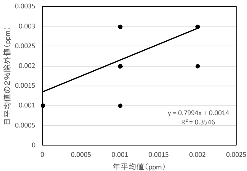
図 8. 1-19 (1) 一般環境大気測定局年平均值・日平均値の2%除外値散布図 (二酸化硫黄)
