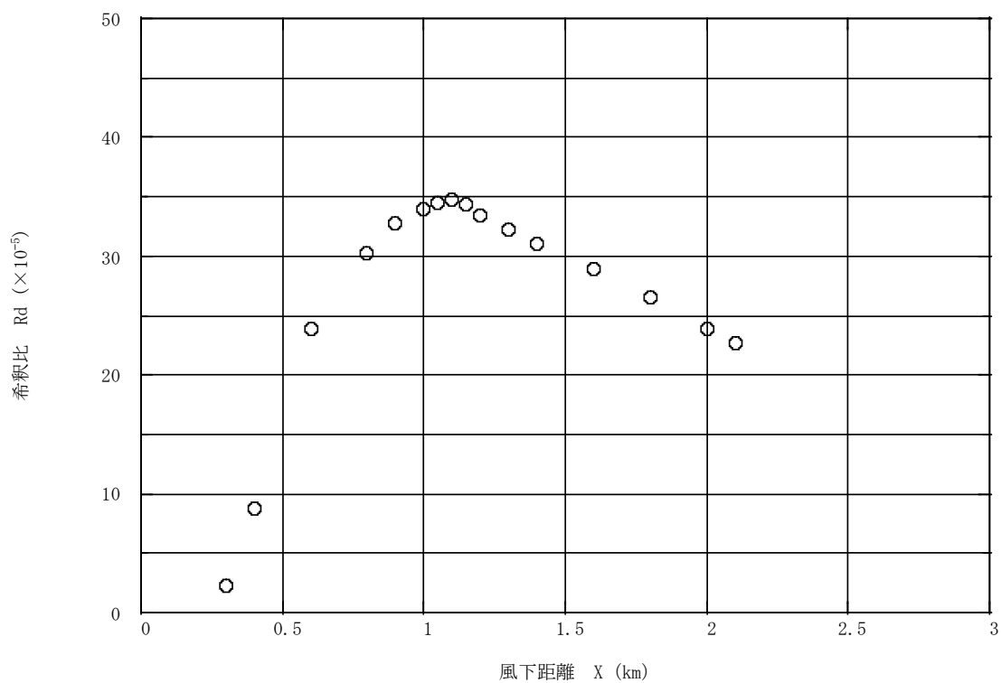
図 8.1-16(4) 地形地表面煙軸濃度分布【風向:東、風速 3.5m/秒】
