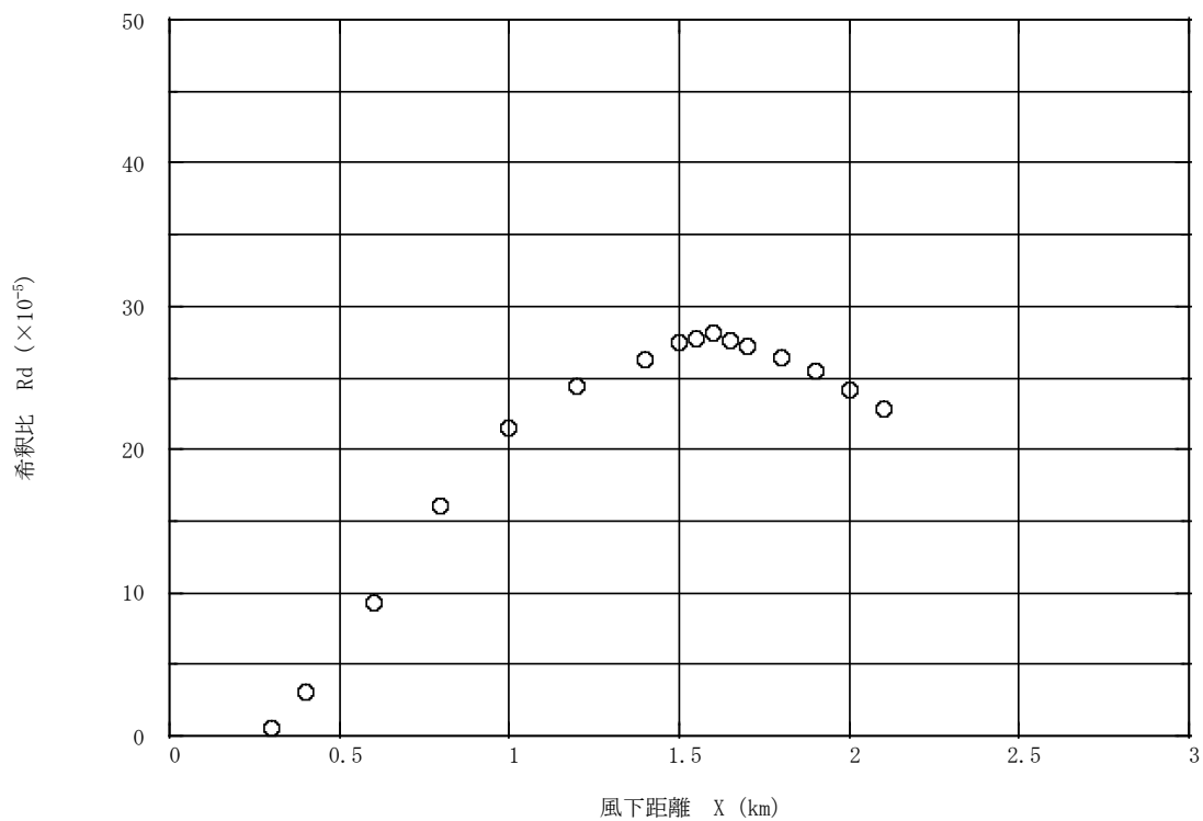
図 8.1-16(3) 地形地表面煙軸濃度分布【風向:東、風速 1.8m/秒】
