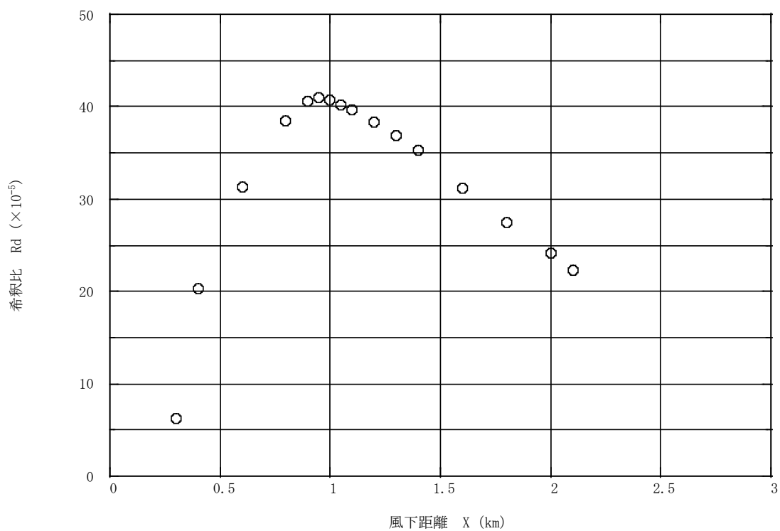
図 8.1-16(2) 地形地表面煙軸濃度分布【風向:北、風速 3.5m/秒】
