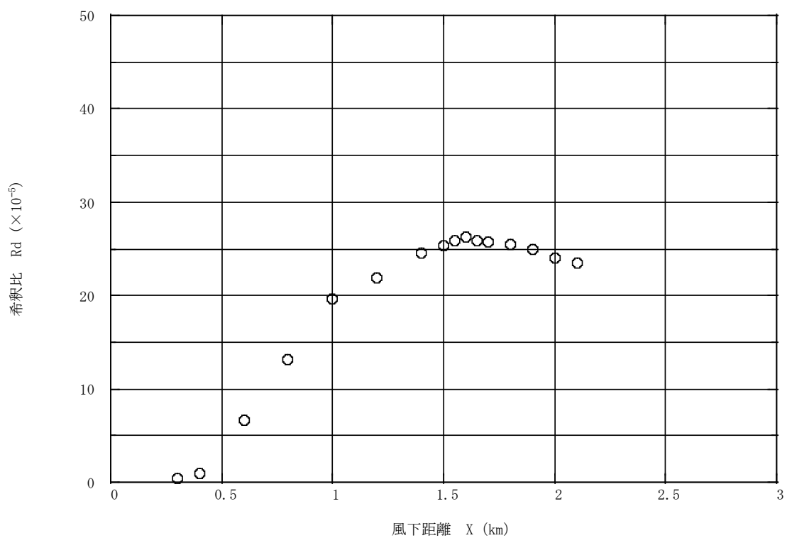
図 8.1-16(5) 地形地表面煙軸濃度分布【風向:西、風速 1.8m/秒】
