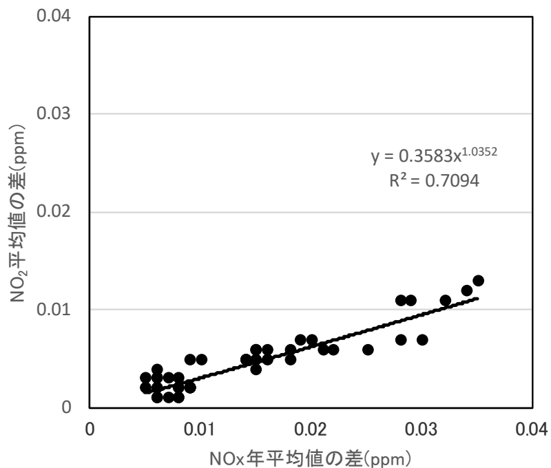
図 8.1-8 自動車の寄与による窒素酸化物と二酸化窒素の散布図 (自動車排出ガス測定局の年平均値と、その測定局から最も近い一般環境大気測定局の平均値の差)
