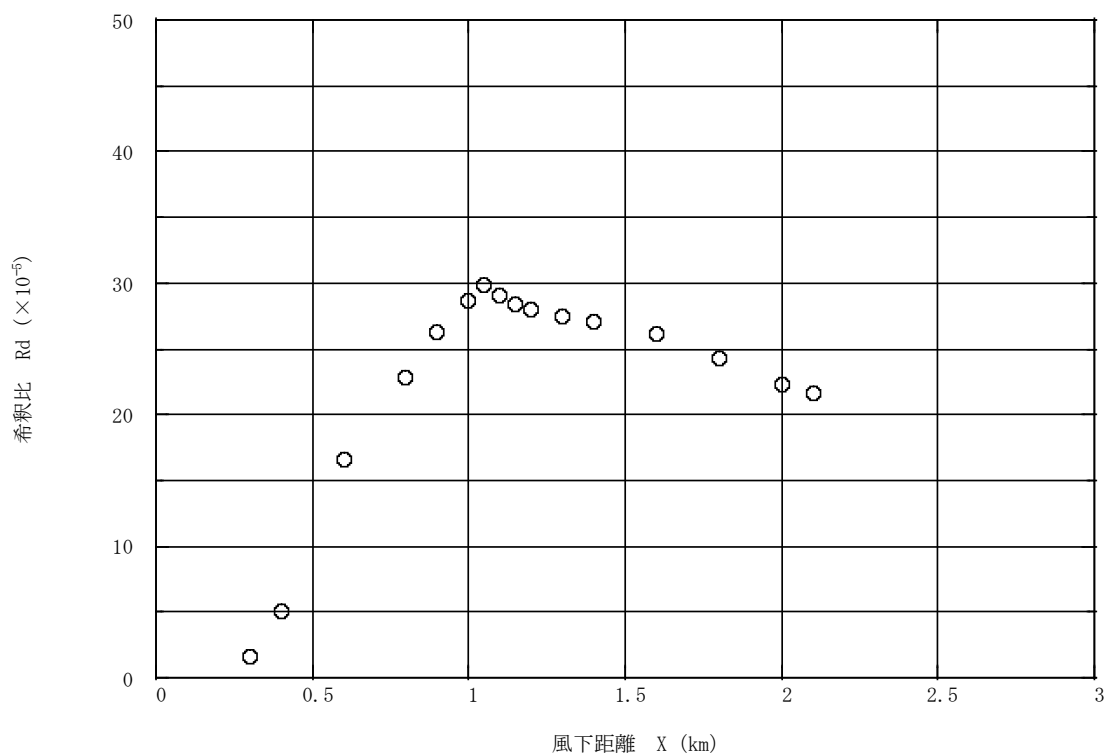
図 8.1-16(6) 地形地表面煙軸濃度分布【風向:西、風速 3.5m/秒】
