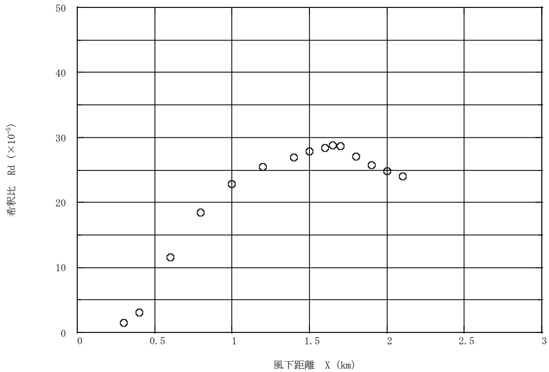
図 8.1-16(7) 地形地表面煙軸濃度分布【風向:南、風速 1.8m/秒】
