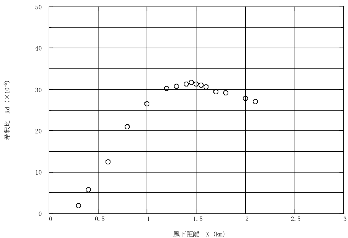
図 8.1-16(1) 地形地表面煙軸濃度分布【風向:北、風速 1.8m/秒】
