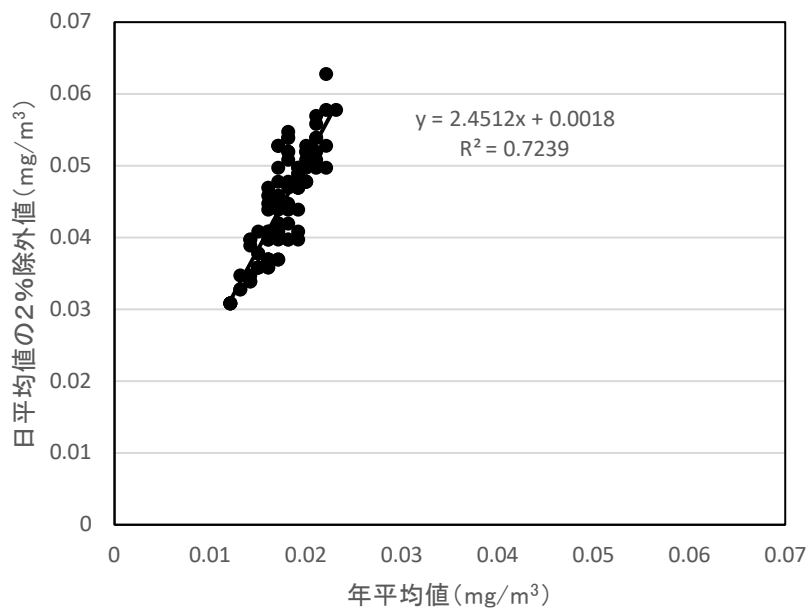
図 8. 1-19 (2) 一般環境大気測定局年平均值・日平均値の2%除外値散布図 (浮遊粒子状物質)
