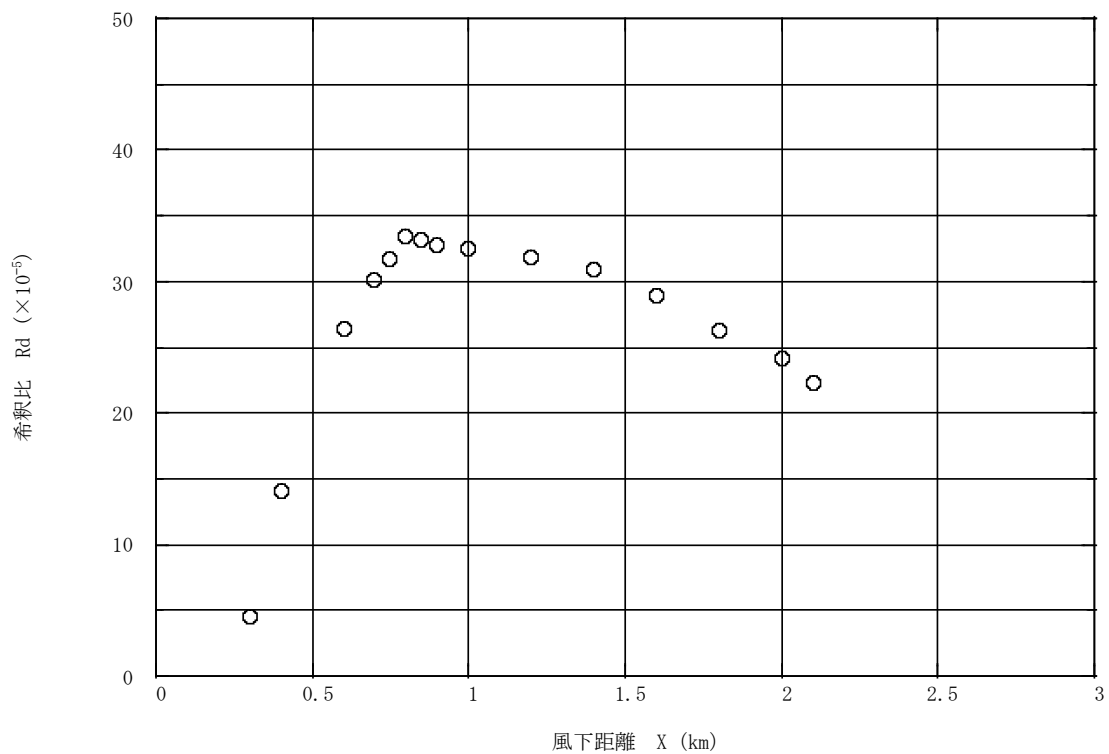
図 8.1-16(8) 地形地表面煙軸濃度分布【風向:南、風速 3.5m/秒】
