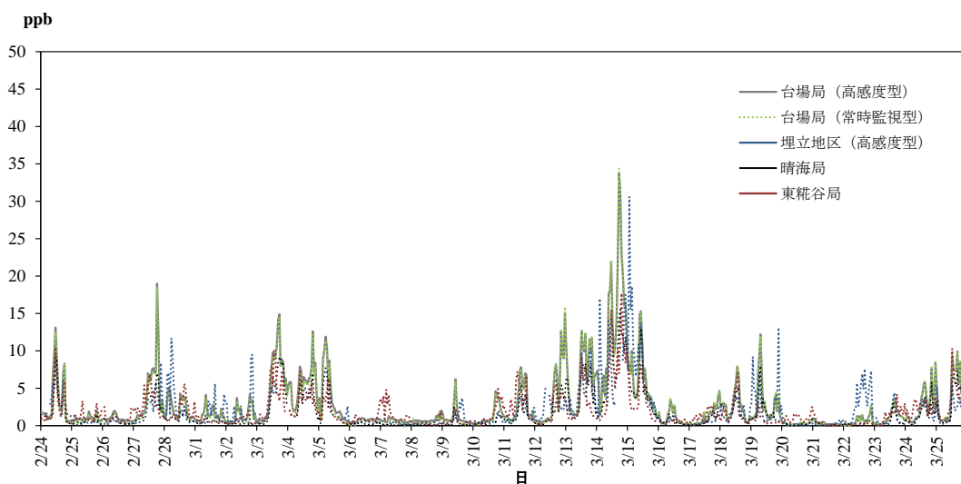
図 3-2 冬季予備調査の SO 2 測定結果
