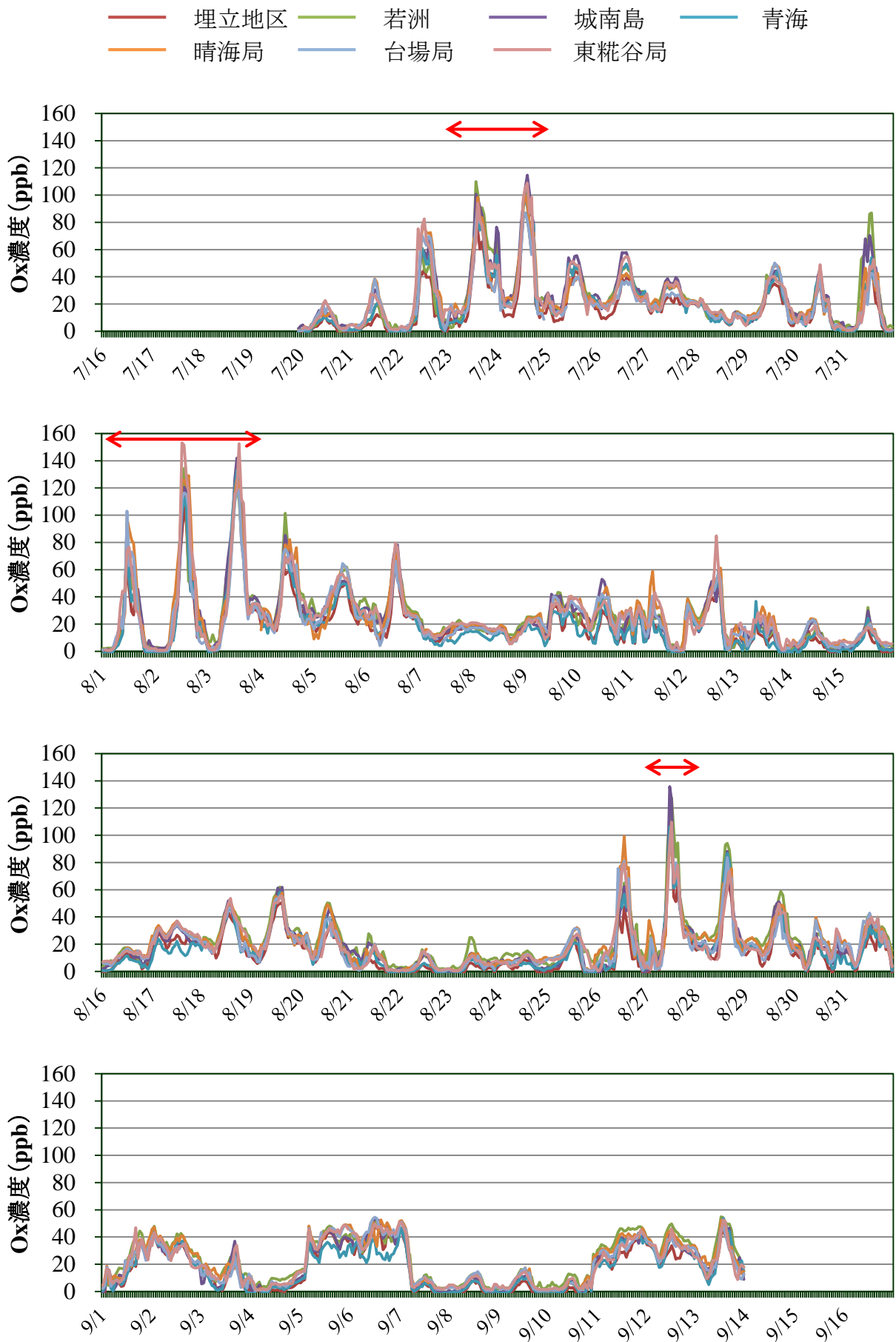
図 4-6 各調査地点における測定結果 (Ox)
