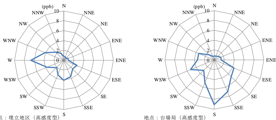
図 3-3 風向別 SO 2 濃度 (左図：埋立地区、右図：台場局)
