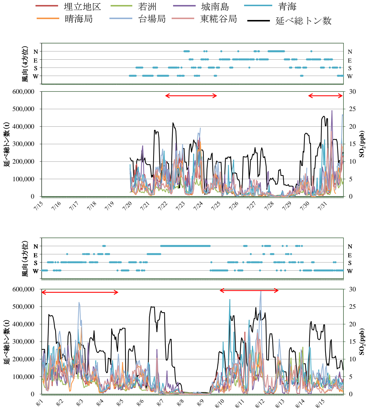
図 4-12 東京港の入出港データ（速報値）を基に求めた「延べ総トン数」と各調査地点の SO 2 濃度（7 月後半～8 月前半）
