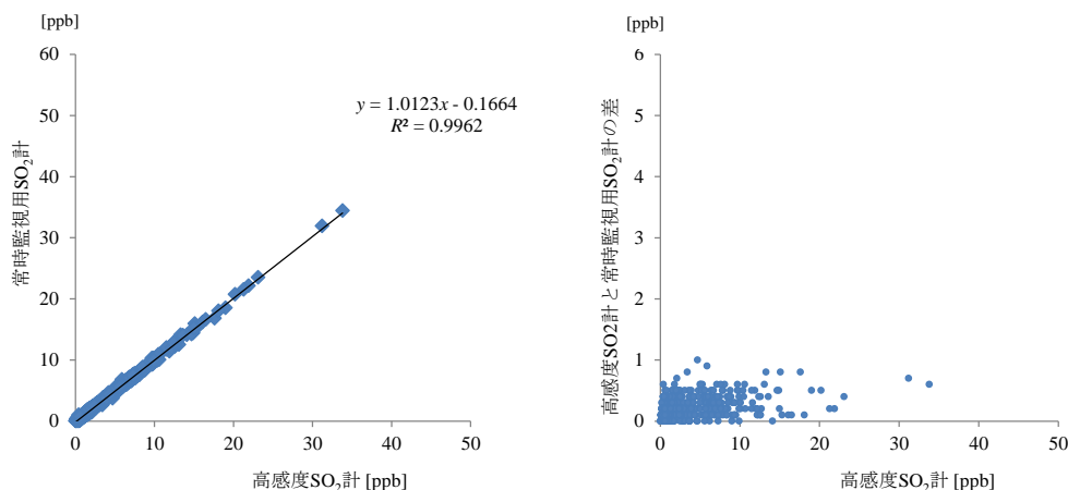
図 3-1 常時監視型 SO 2 計と高感度型 SO 2 計の関係
