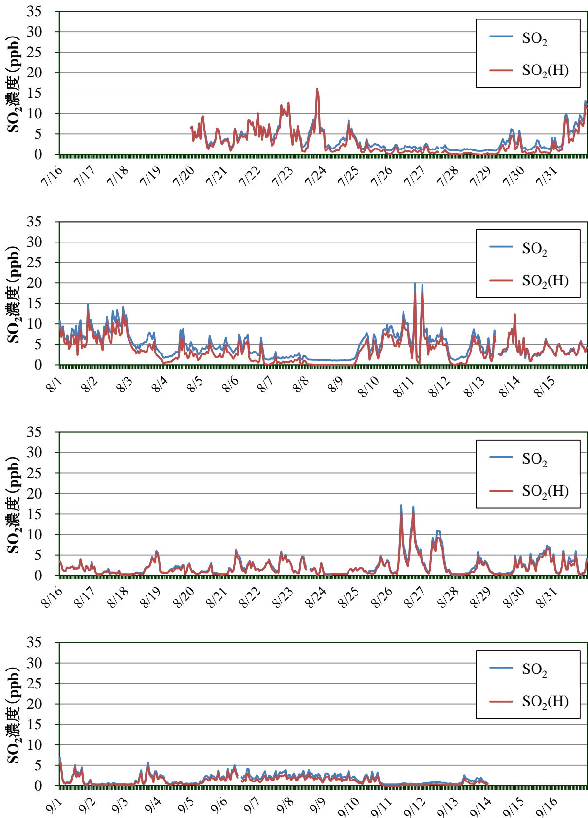
図 4-2 調査期間における埋立地区の SO 2 濃度 (常時監視型、高感度型)
