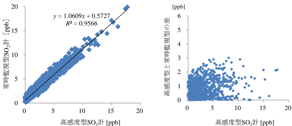
図 4-1 埋立地区における常時監視型 SO 2 計と高感度型 SO 2 計の関係
