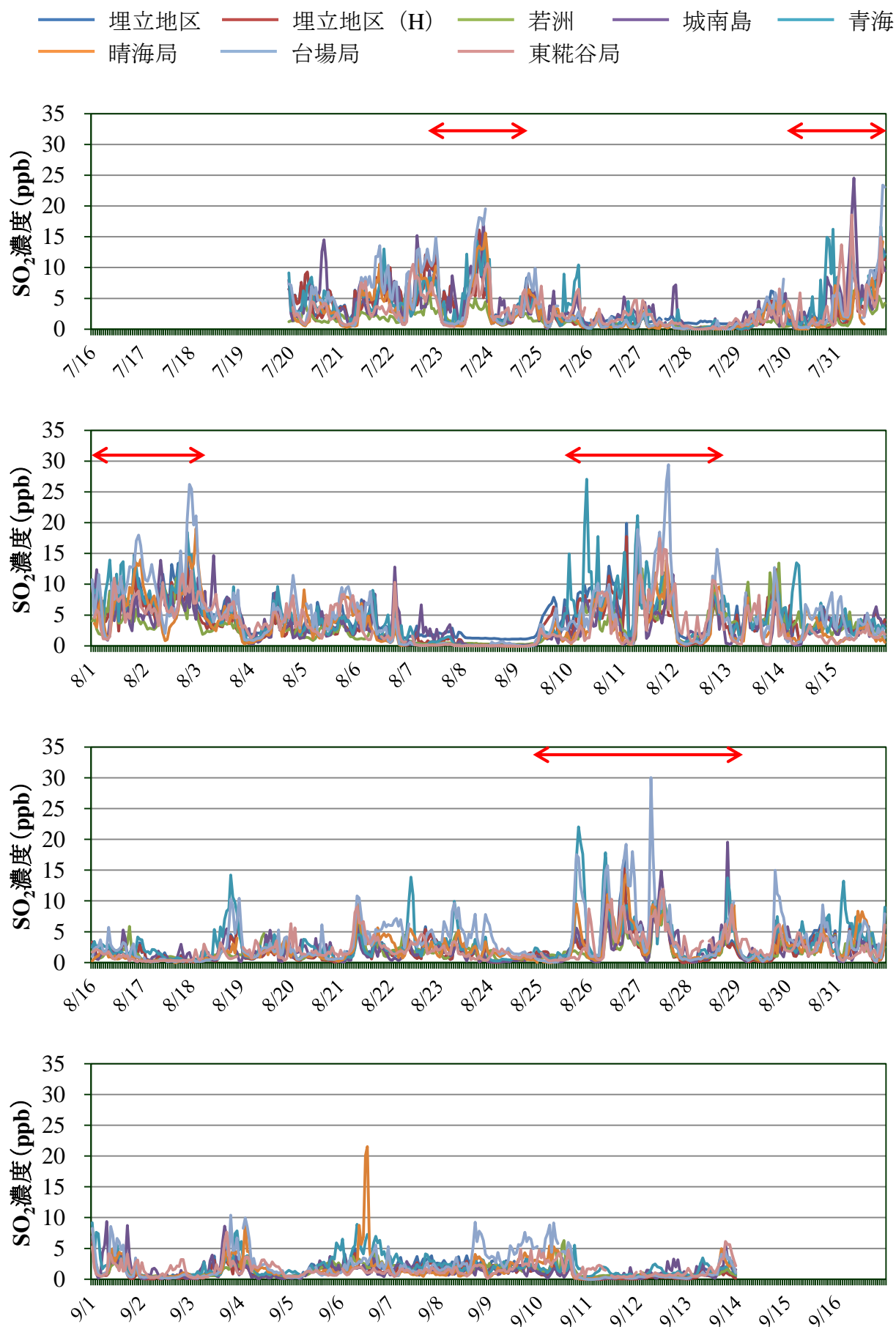
図 4-3 各調査地点における測定結果 (SO 2 )
