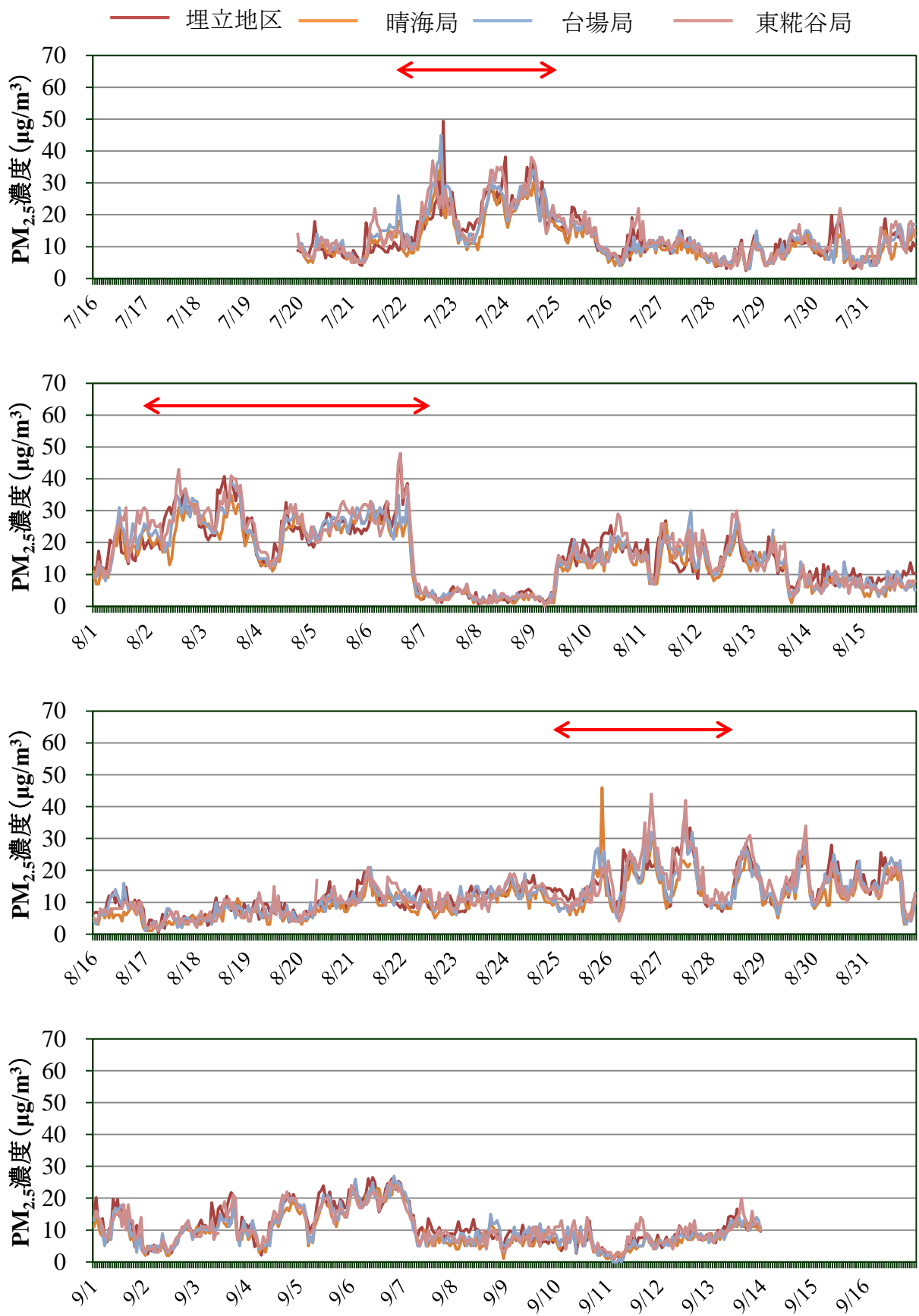
図 4-7 各調査地点における測定結果 (PM 2.5 )
