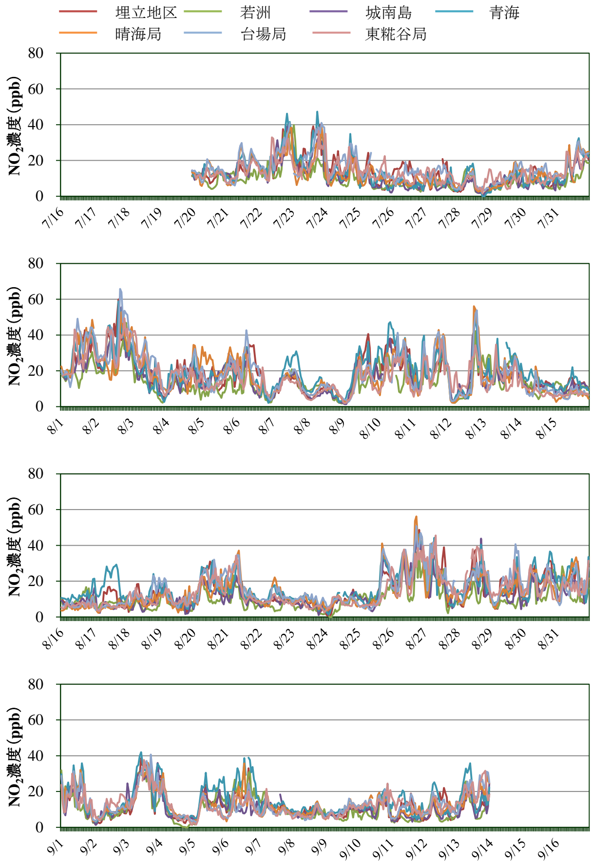
図 4-5 各調査地点における測定結果 (NO 2 )
