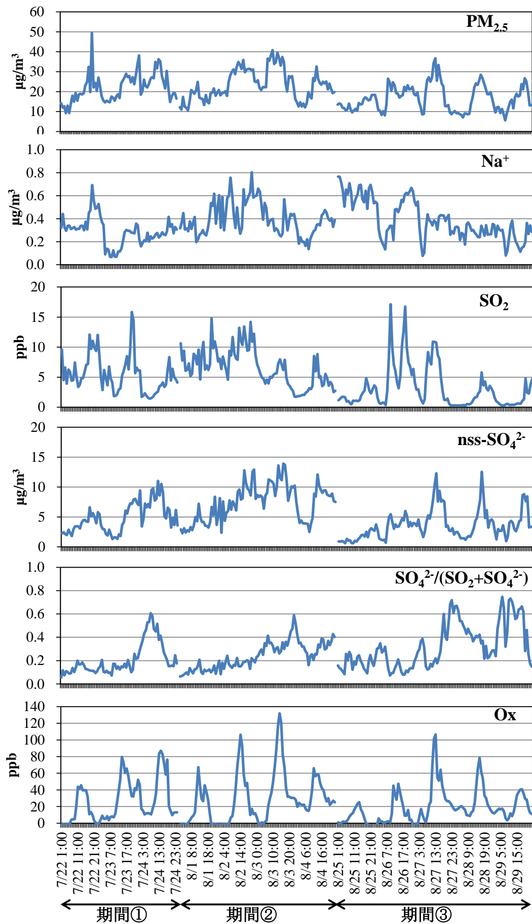
図 4-14 埋立地区における PM_{2.5} 、 Na^+ 、 SO_2 、 nss-SO_4^{2-} 、粒子化率、 Ox 濃度の経時変化
