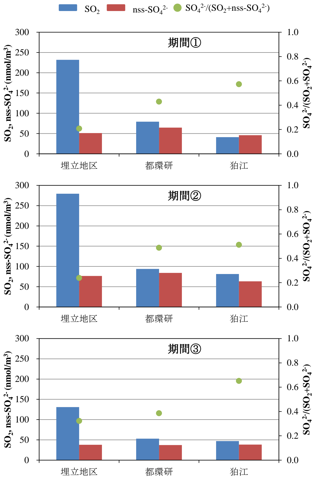
図 4-16 各地点における各高濃度期間の \text{SO}_2 、 \text{nss-SO}_4^{2-} 、粒子化率
