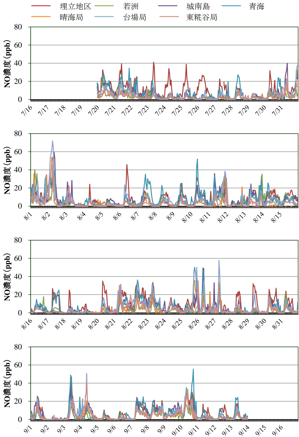
図 4.4 各調査地点における測定結果 (NO)
