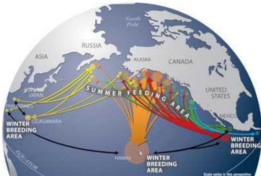
北太平洋におけるザトウクジラの回遊ルート
