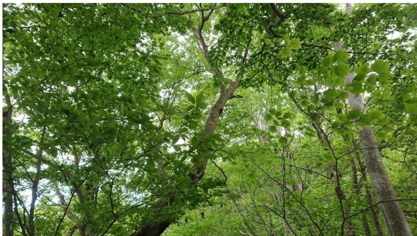
植物の光合成による酸素の生成
