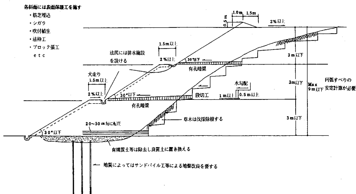
图 盛土工
