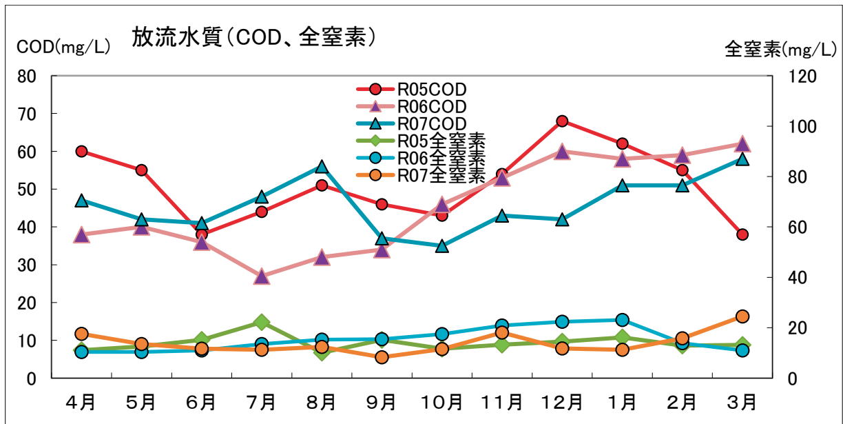
グラフ2 令和5年度～令和7年度処理水の水質（COD、全窒素）
