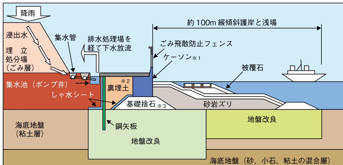
図3 ケーソン式外周護岸
