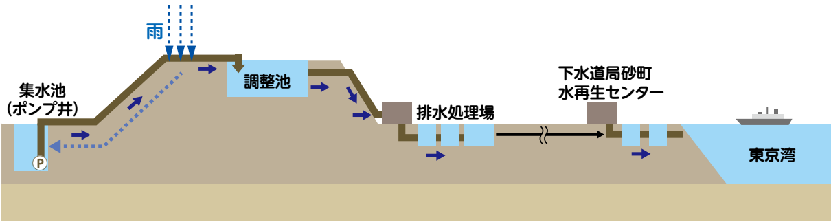
図6 浸出水の流れ
