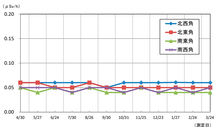
グラフ 3 外側埋立処分場等の空間放射線量率(令和 7 年度)
