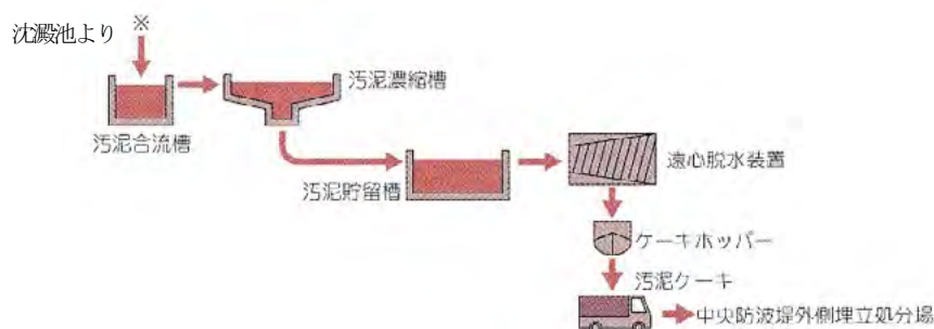
図9 汚泥処理フロー
