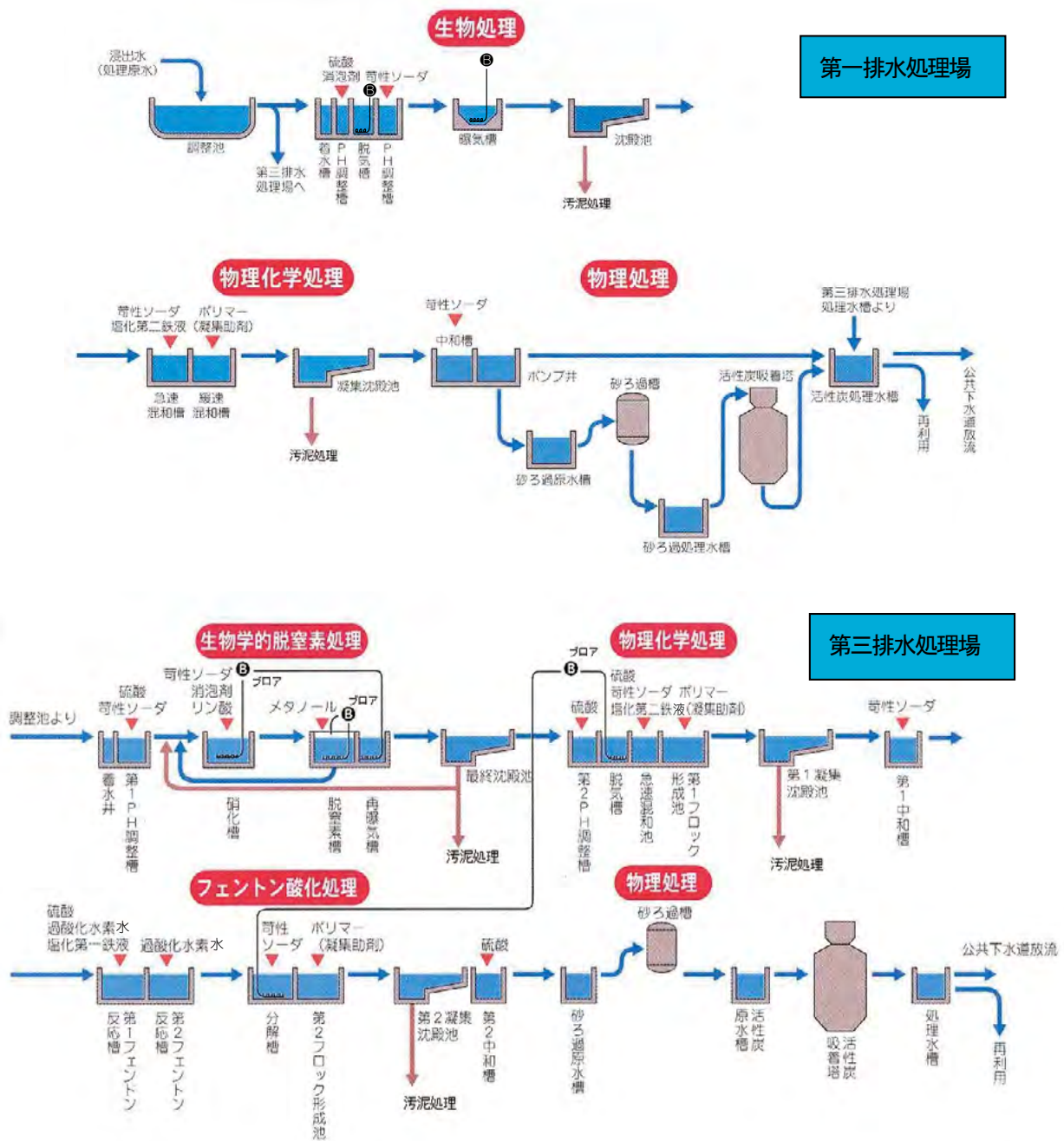
図8 排水（浸出水）処理フロー
