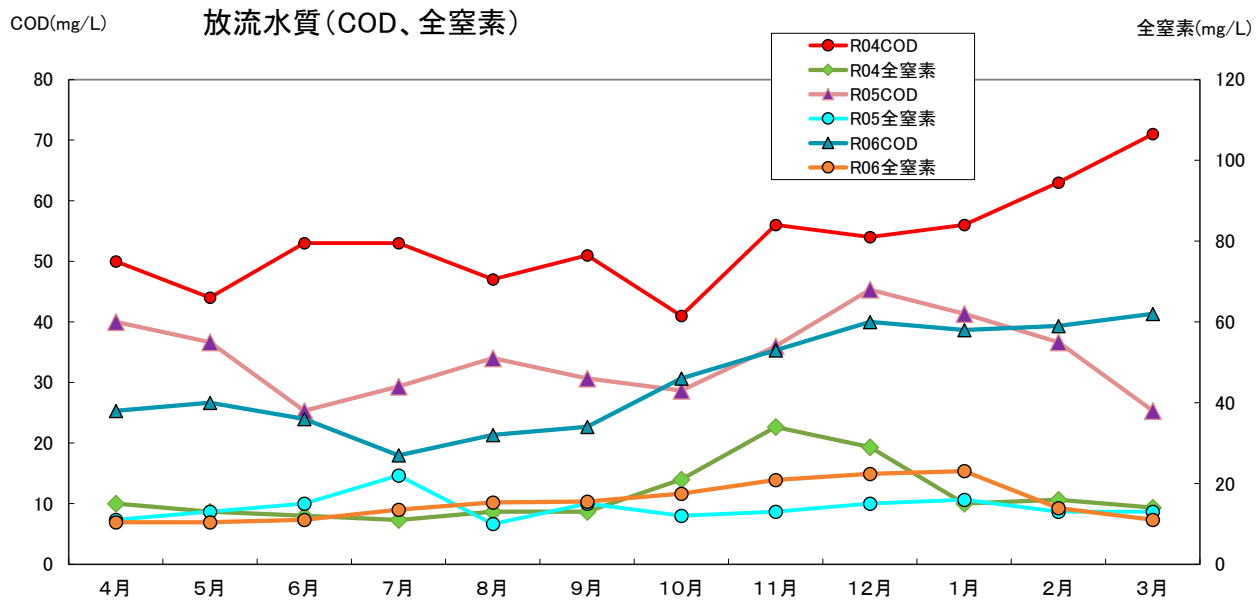
グラフ2 令和4年度～令和6年度処理水の水質（COD、全窒素）
