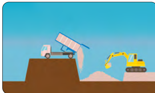
図5 額縁方式
