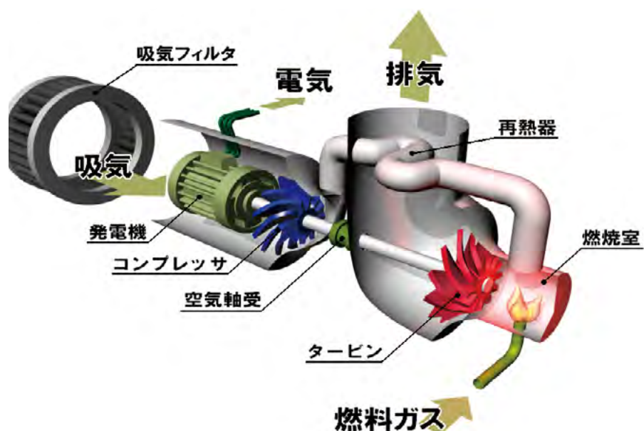
図11 マイクログスタービン発電機の構造
