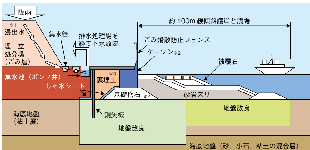
ケーソン式外周護岸（新海面処分場B・Cブロック）
