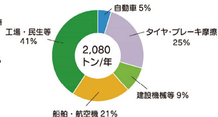
粒子状物質（PM）の排出量
