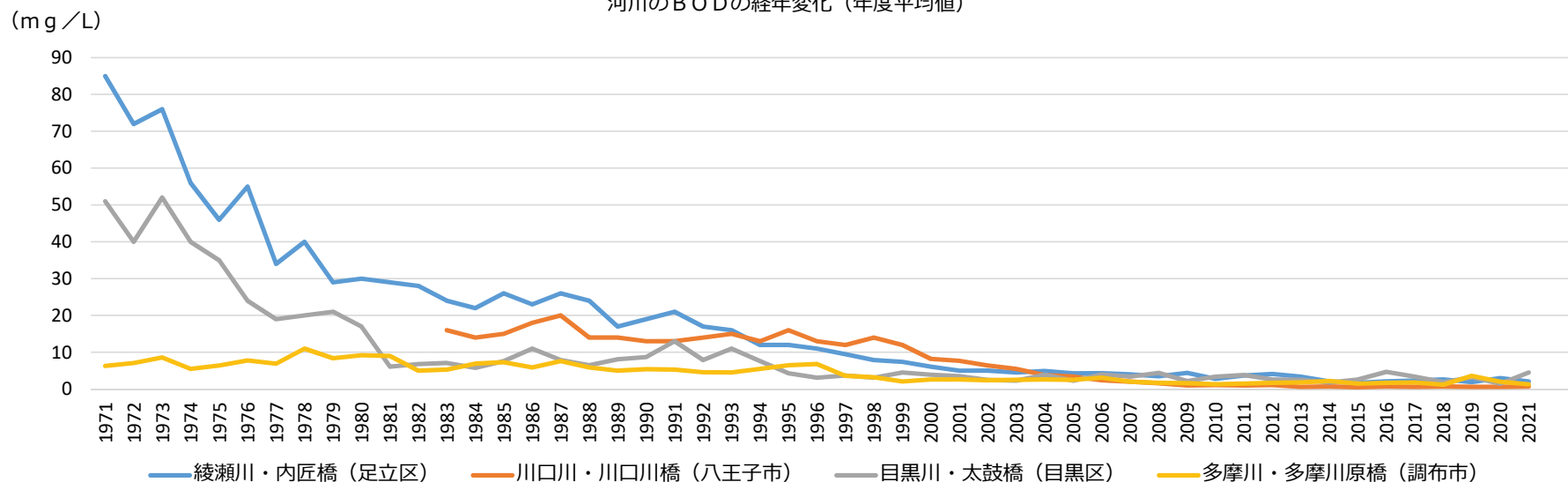
河川のBODの経年変化（年度平均値）
