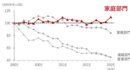
部門別最終エネルギー消費の推移
