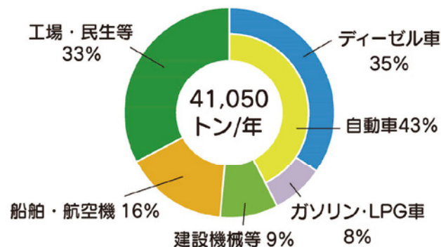
都内の窒素酸化物（NO x ）の排出量
