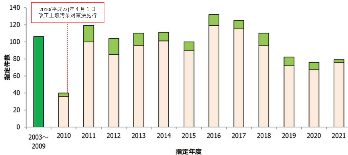
土壌汚染対策法に基づく指定区域又は要措置区域等の指定件数の推移
