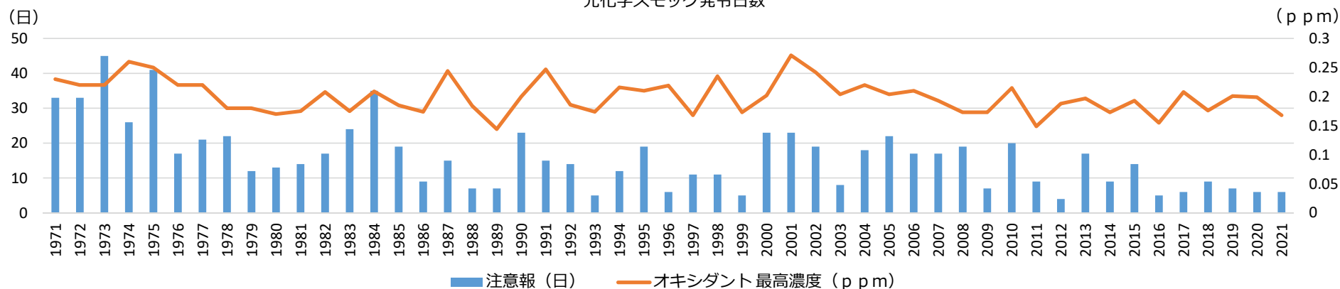
光化学スモッグ発令日数
