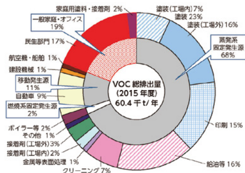
都内のVOC総排出量推計の内訳
