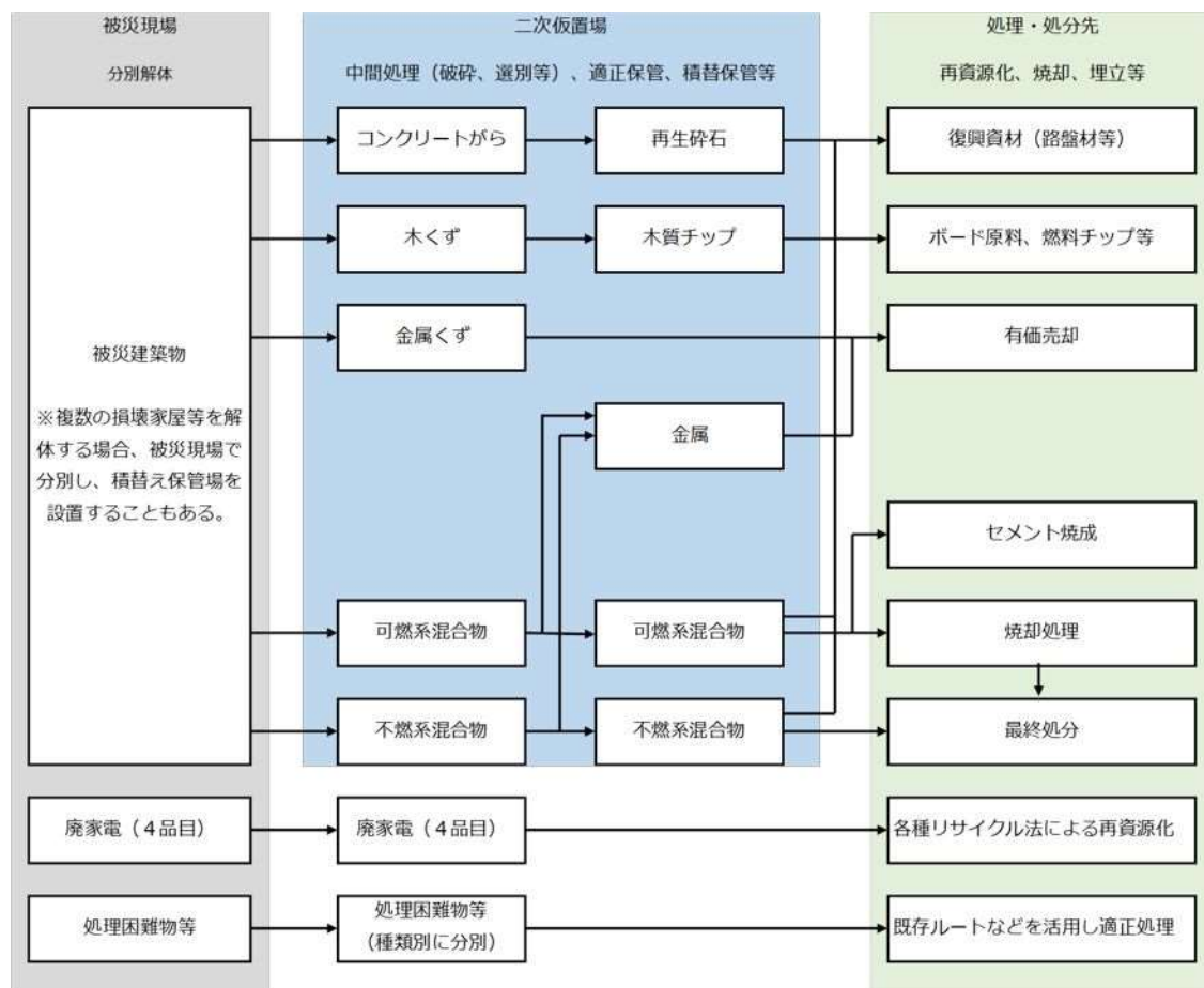
図7 解体廃棄物等（一部片付けごみを含む。）の標準処理フロー
