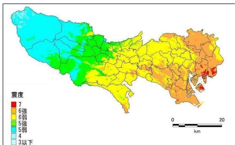
図2 都心南部直下地震における地震動分布
