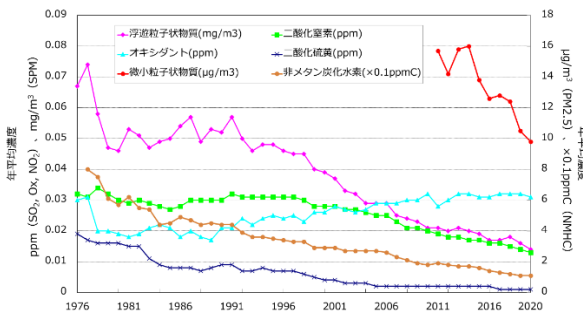
大気環境濃度の推移(一般局平均)
