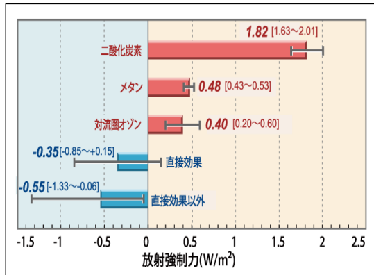
主要温室効果ガスの放射強制力※2
