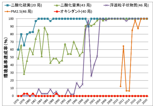
環境基準達成率の推移(一般局)
