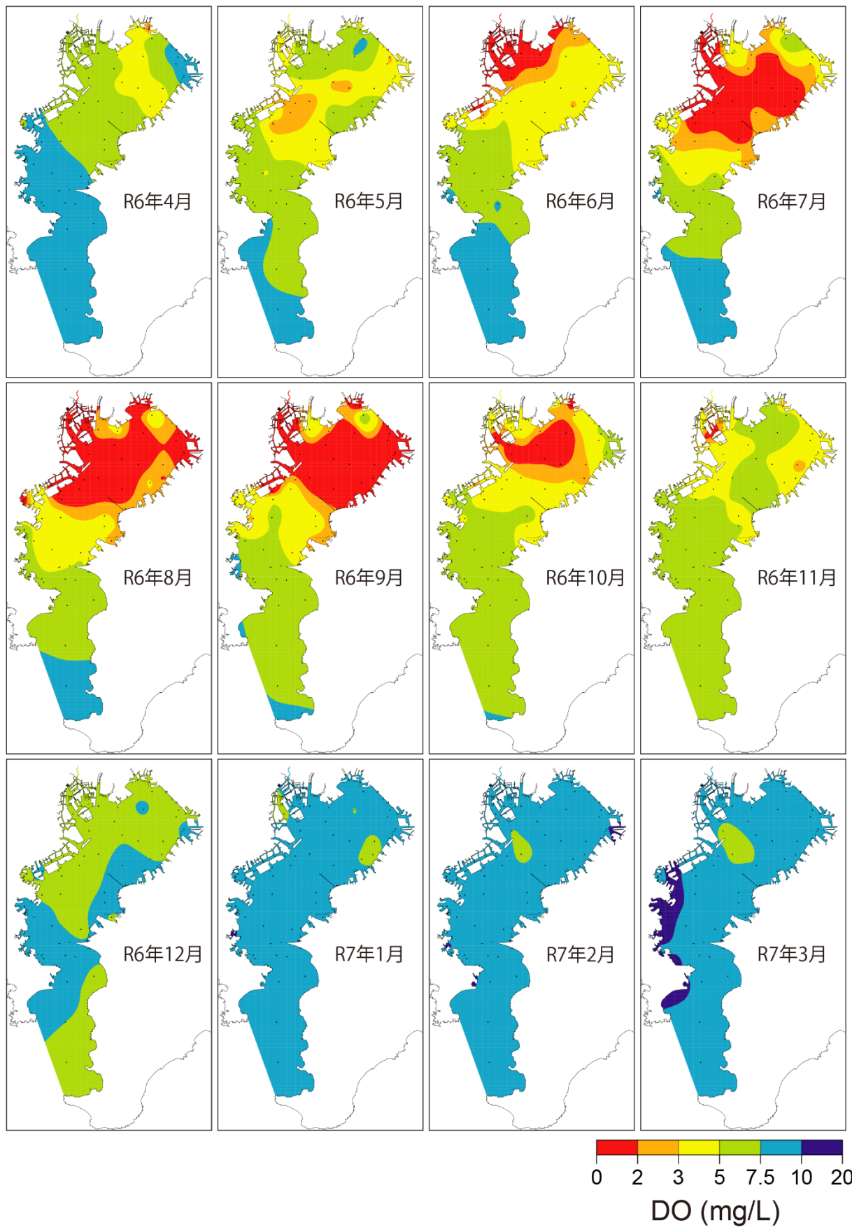
図 22-5 溶存酸素量(DO)(下層)の月別水平分布
