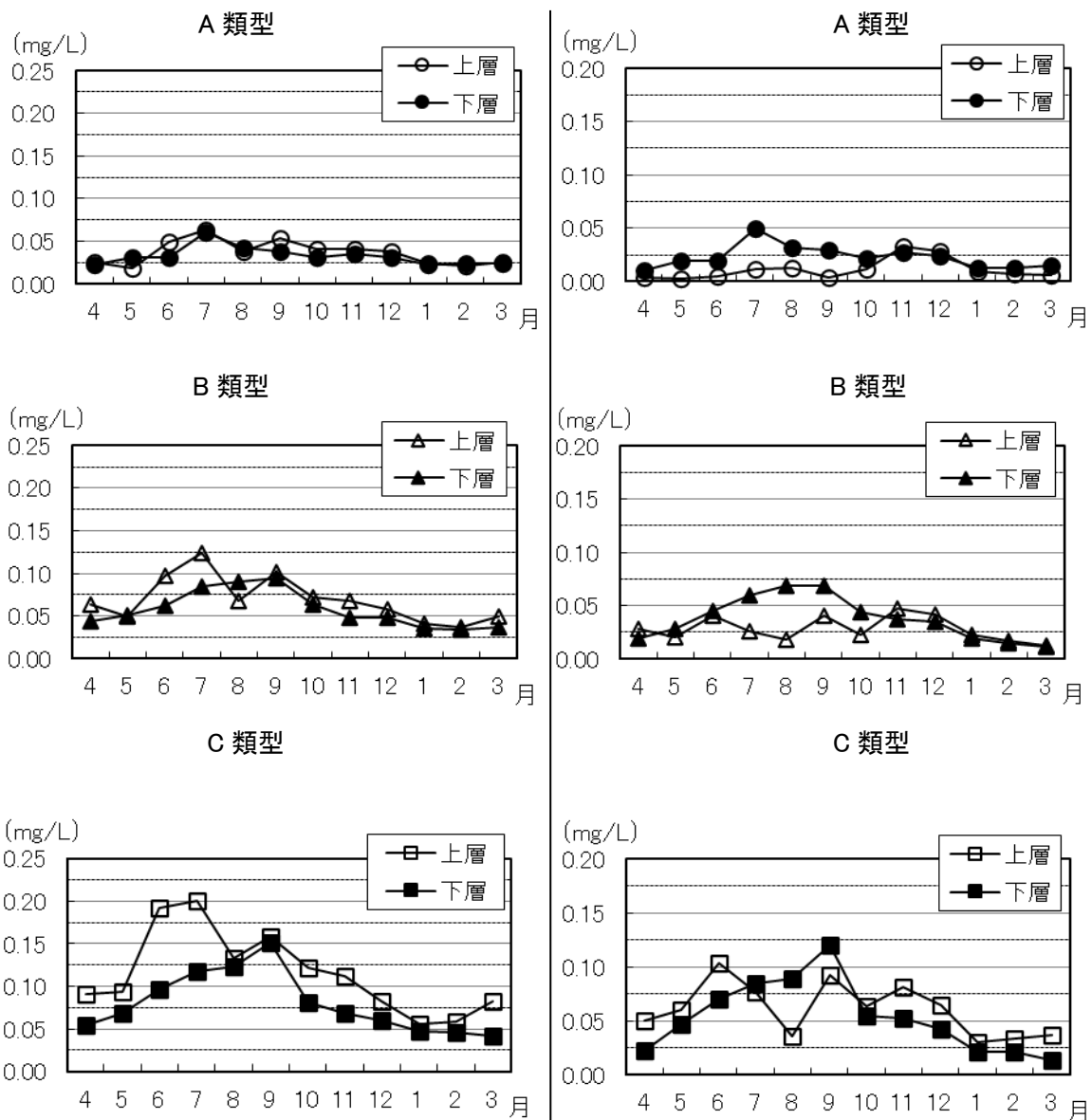
図 18 全りんの变化
