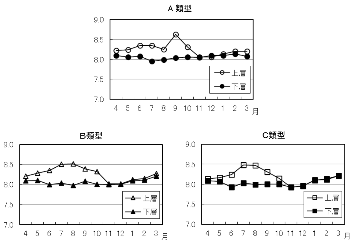
図 15 pH の月変化
