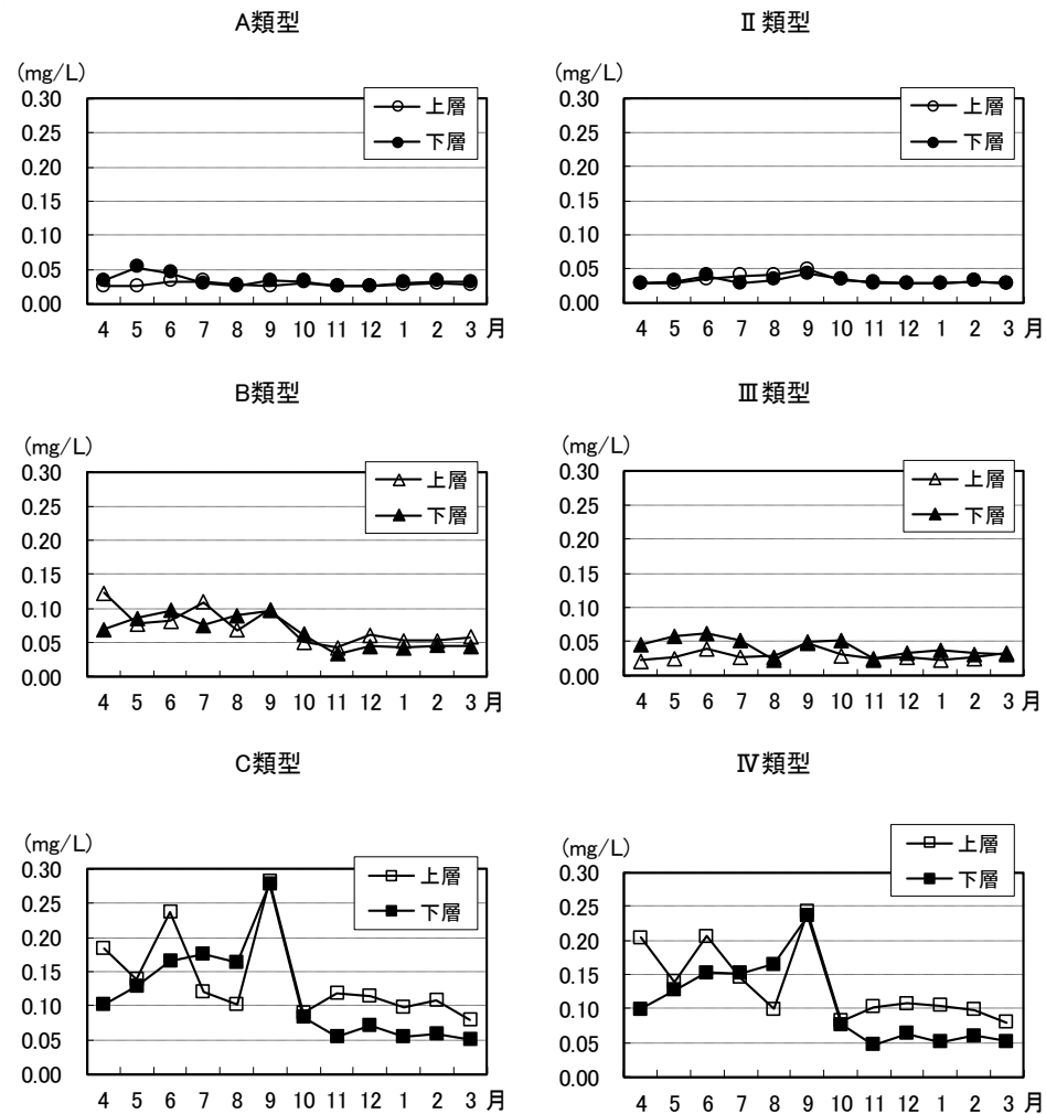
図 35 類型別アンモニア性窒素の月変化
