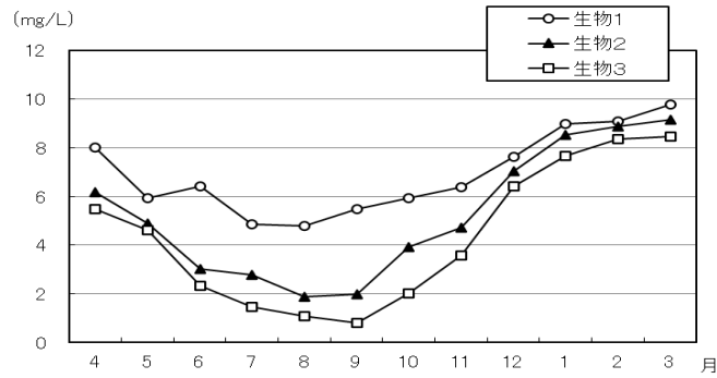
図 14 底層溶存酸素量(下層 DO)の月変化
