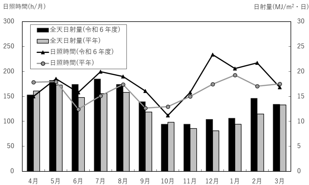
図 26-2 全天日射量及び日照時間の月変化(令和6年度と平年 (※) との比較)
