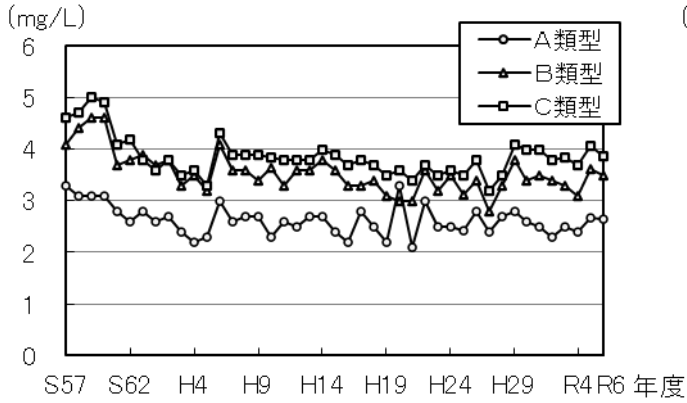
図 3-1 上層 COD の類型別経年変化
