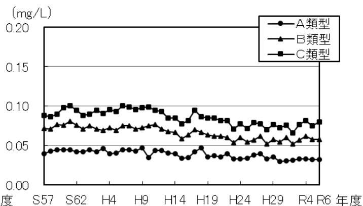
図 5-2 下層全りんの類型別経年変化
