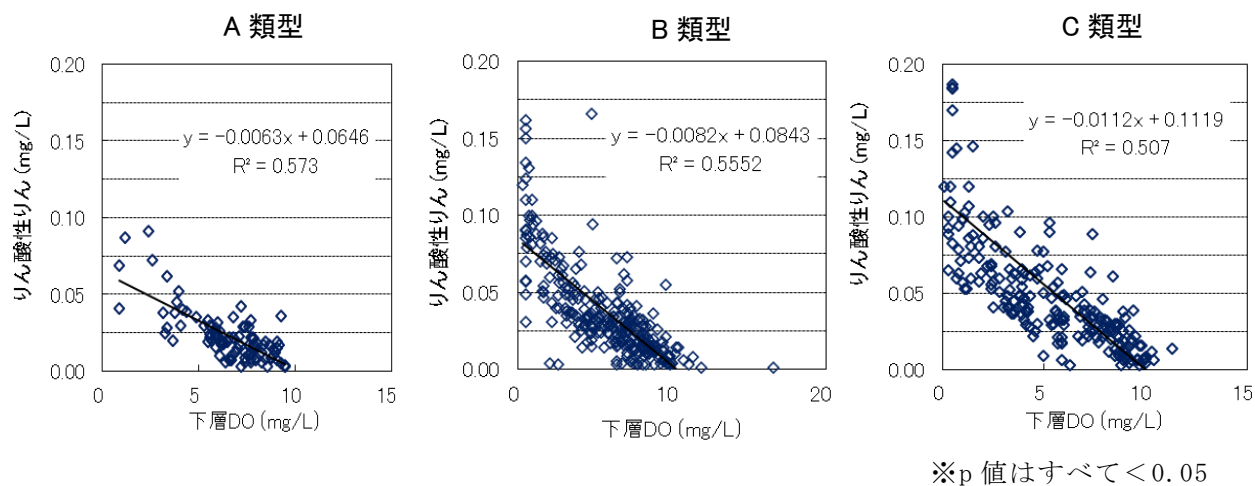
類型別下層 DO と下層りん酸性りんの関係(令和6年度)
