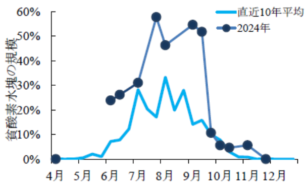
図 29 縦断ラインにおける貧酸素水塊の規模の季節変化
