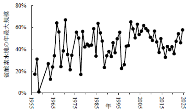
図 30 年最大規模の経年変化
