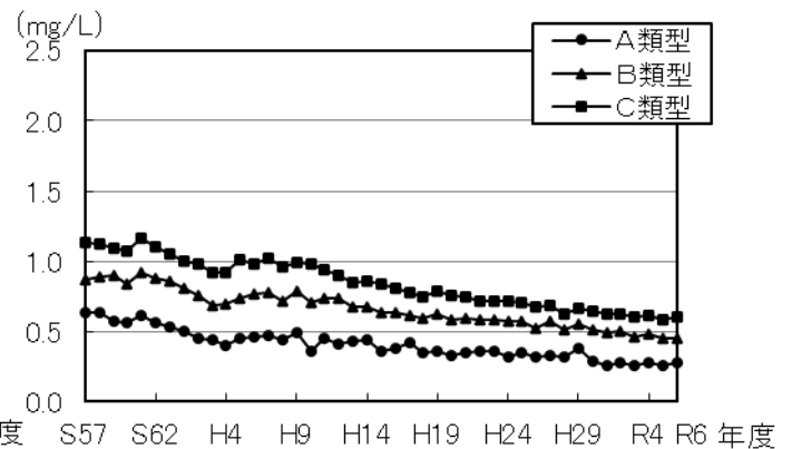
図 4-2 下層全窒素の類型別経年変化
