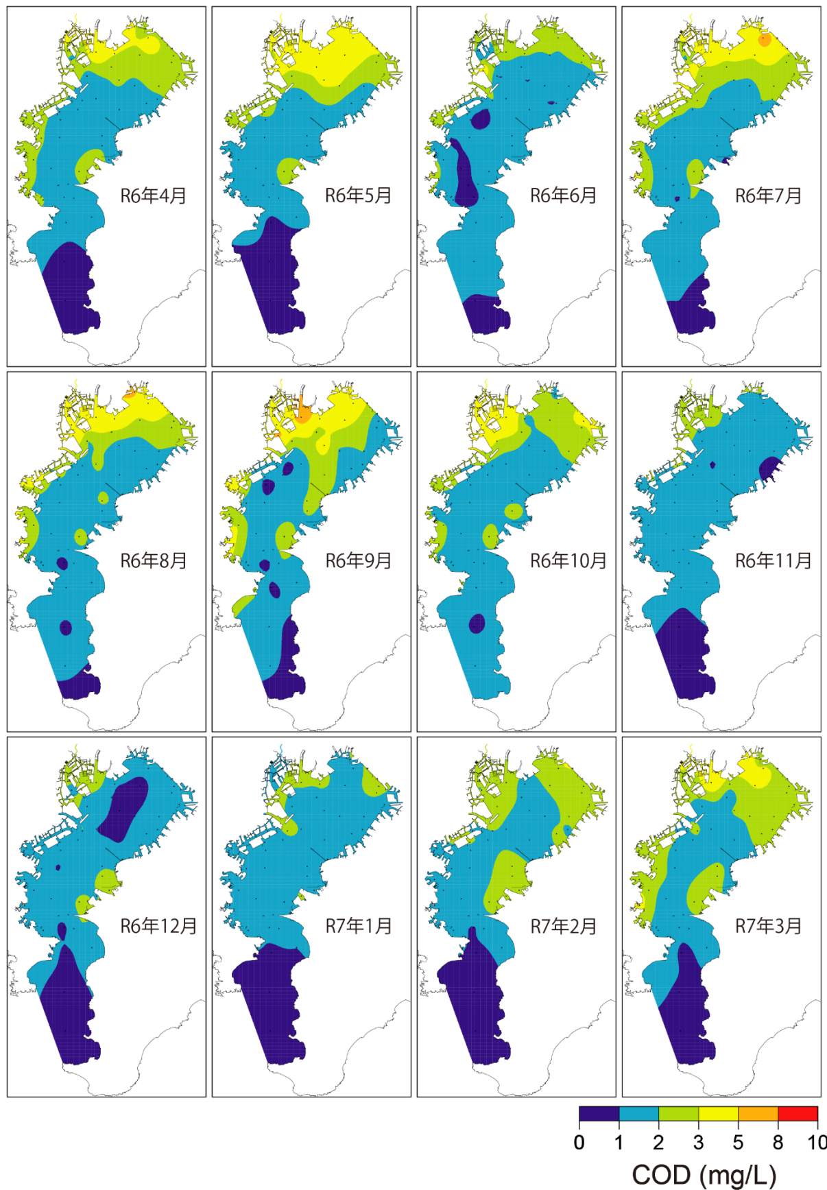
図 22-2 COD(下層)の月別水平分布
