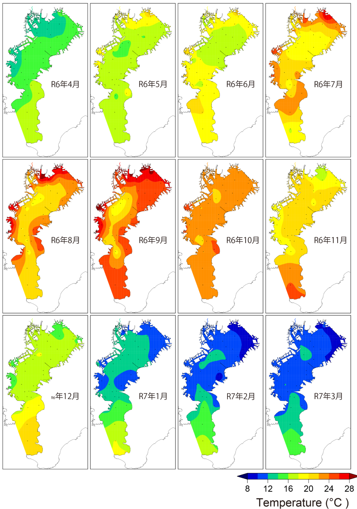
図 22-12 水温(下層)の月別水平分布
