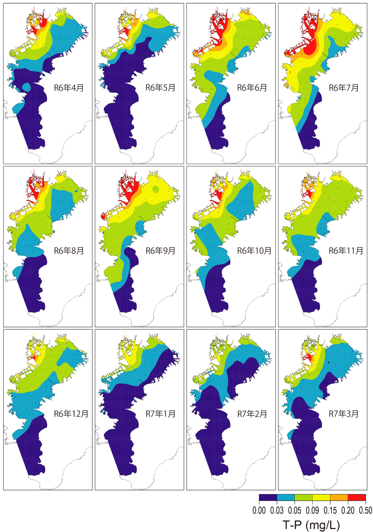
図 22-9 全りん(上層)の月別水平分布
