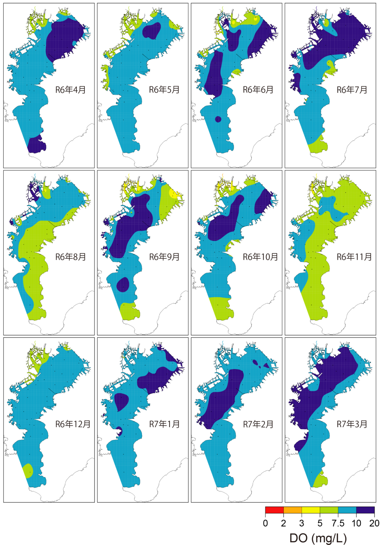
図 22-4 溶存酸素量(DO)(上層)の月別水平分布
