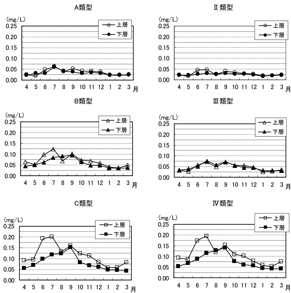
図 36 類型別全りんの月変化
