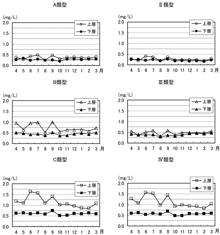
図 34 類型別全窒素の月変化
