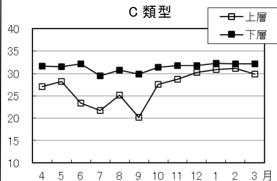
図10 塩分の月変化
