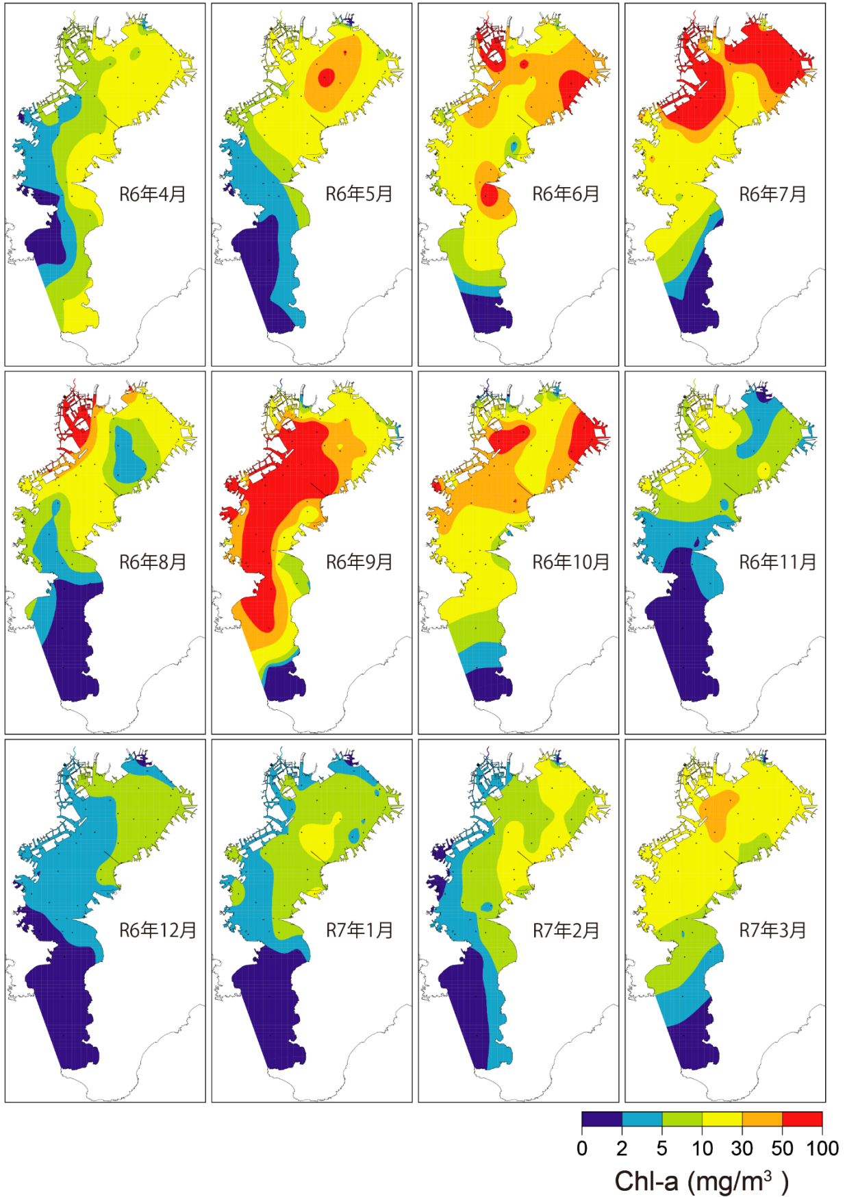
図 22-6 クロロフィル(上層)の月別水平分布
