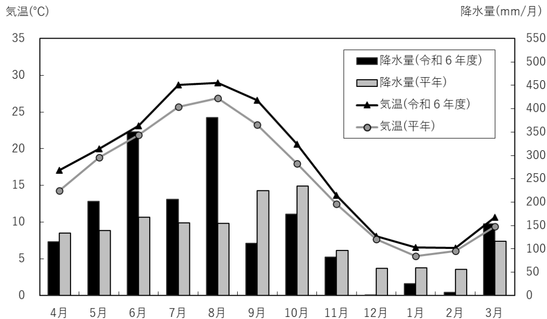
図 26-1 降雨量及び気温の月変化(令和6年度と平年 (※) との比較)
