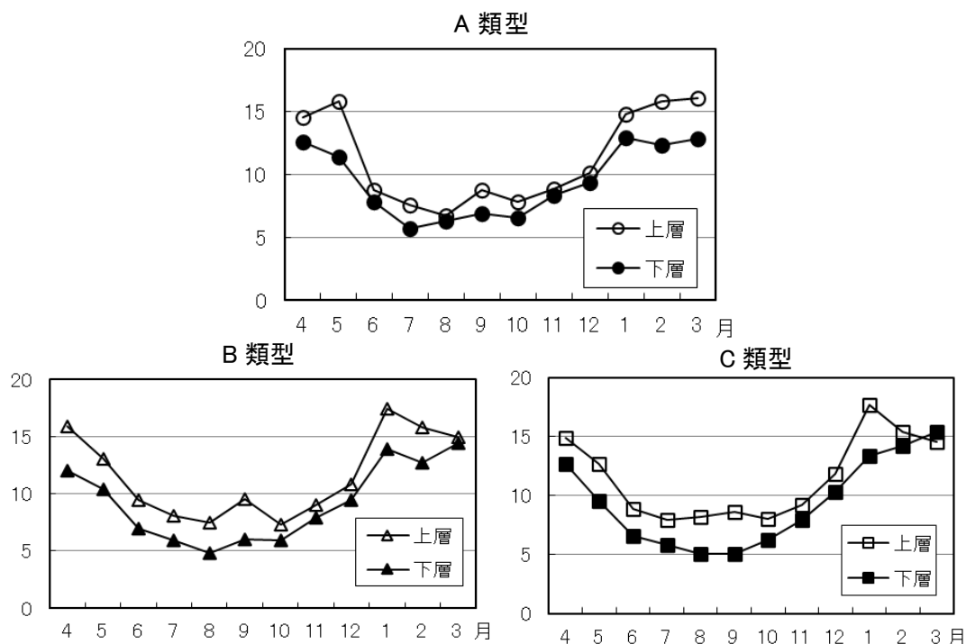
図 20 全窒素／全りん比の月変化
