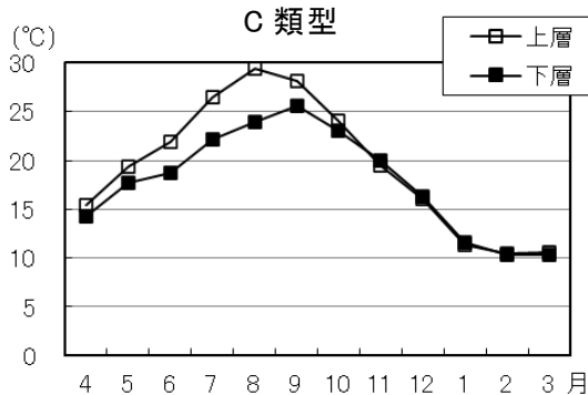
図9 水温の月変化
