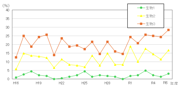
図7 底層の貧酸素割合 類型別経年変化
