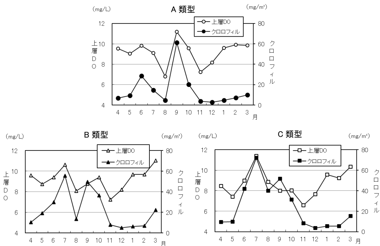
図 13 溶存酸素量(上層 DO)及びクロロフィルの月変化
