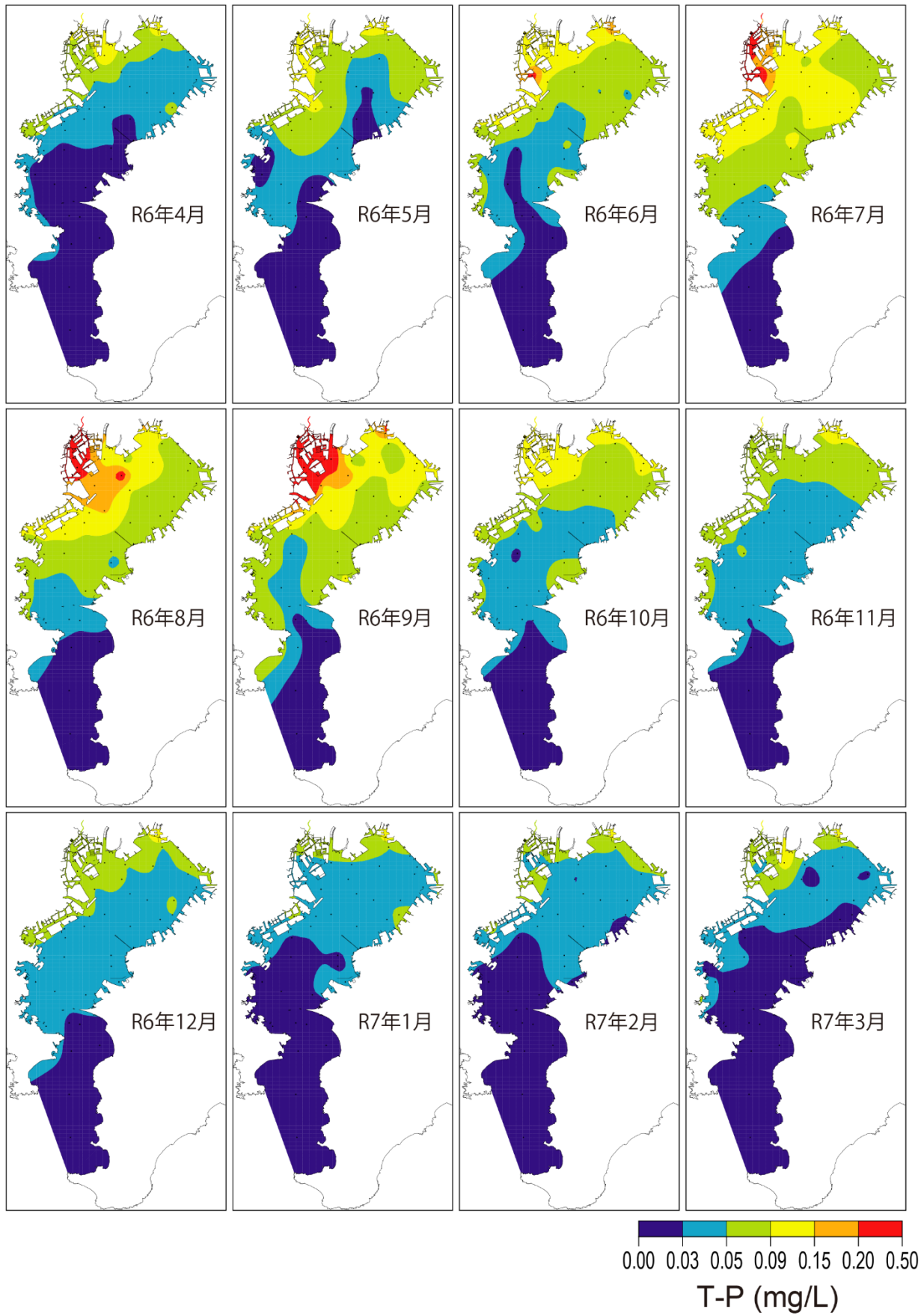
図 22-10 全りん(下層)の月別水平分布
