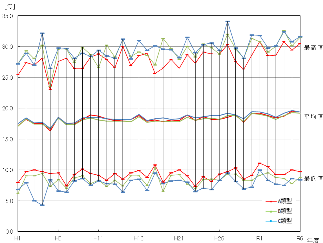
図8 水温（上層）の経年変化
