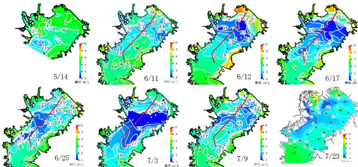
図 28 底層の溶存酸素量分布 (1/2) 等値線の単位は mL/L 赤線は縦断ライン
