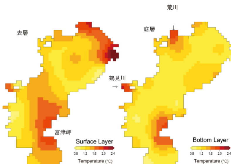
図1 東京湾の表層および底層における水溫の変化 (1985年と2021年の差分)
