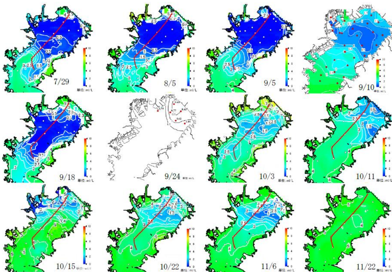
図 28 底層の溶存酸素量分布 (2/2) 等値線の単位は mL/L 赤線は縦断ライン
