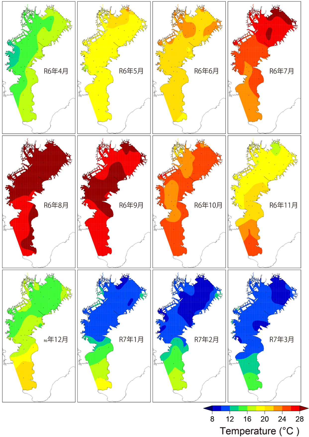
図 22-11 水温(上層)の月別水平分布
