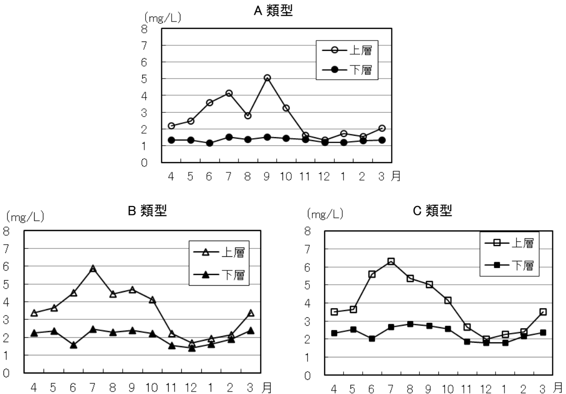
図 11 COD の月変化
