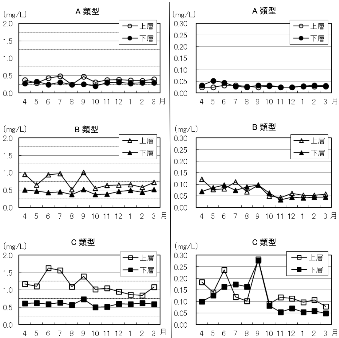
図 16 全窒素の変化
