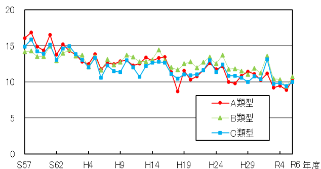
図 21 全窒素／全りん比の経年変化
