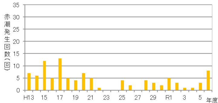
神奈川県地先海域(発生回数)
