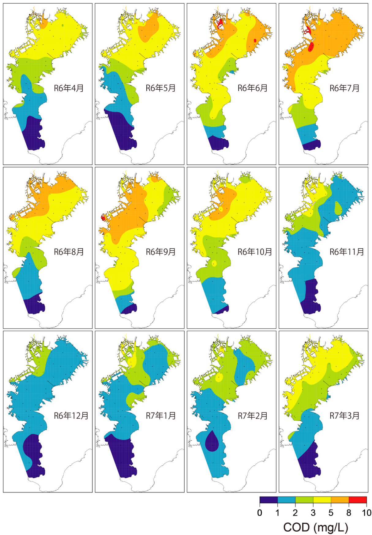
図 22-1 COD(上層)の月別水平分布
