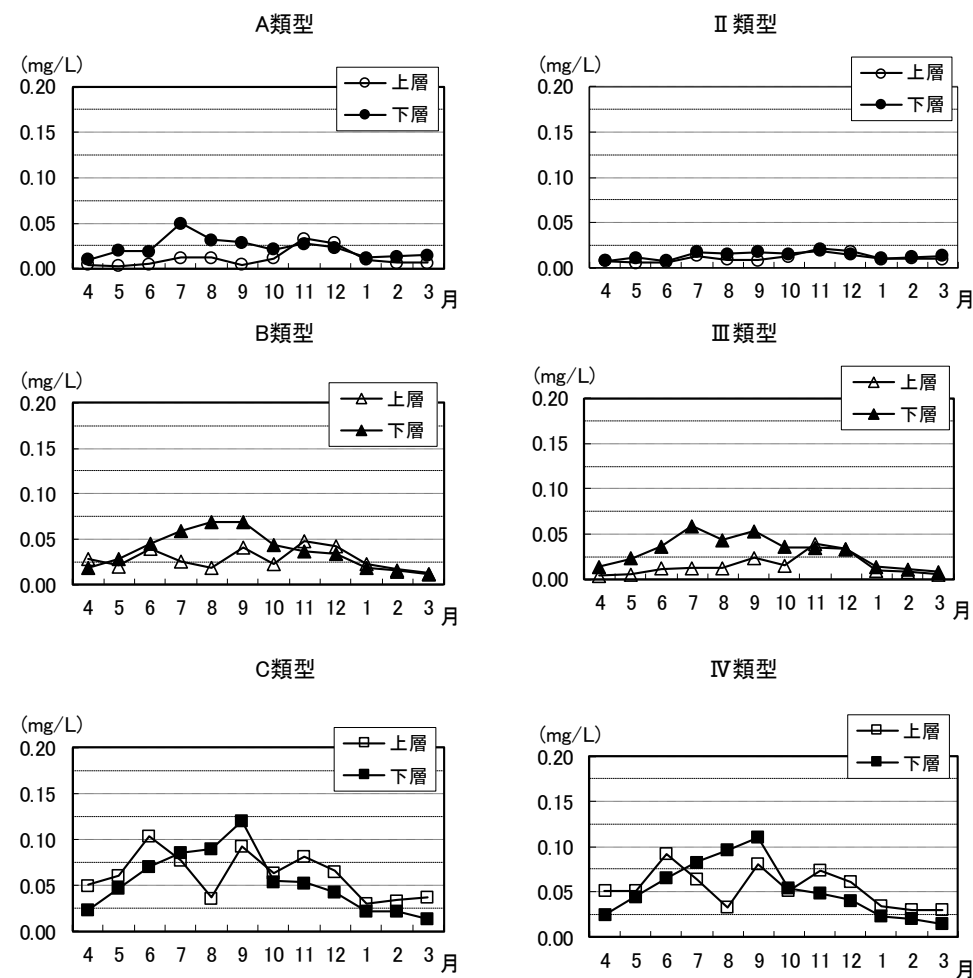
図 37 類型別りん酸性りんの月変化
