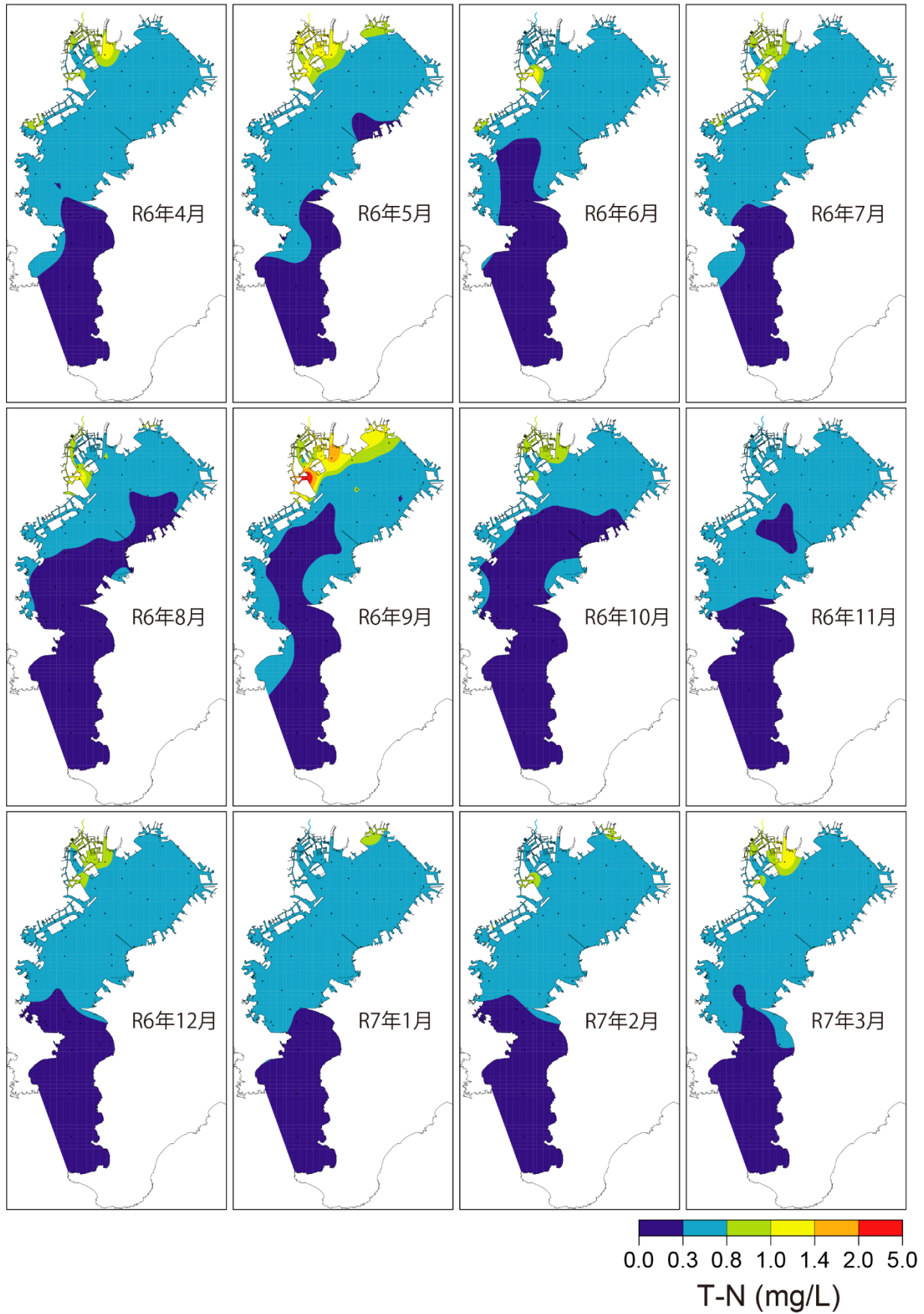
図 22-8 全窒素(下層)の月別水平分布
