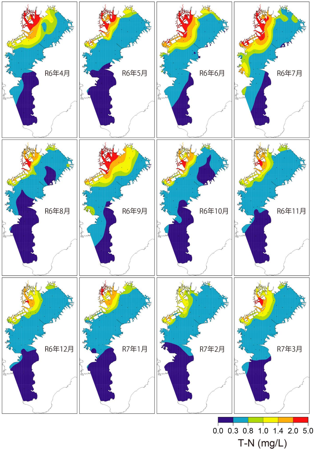
図 22-7 全窒素(上層)の月別水平分布
