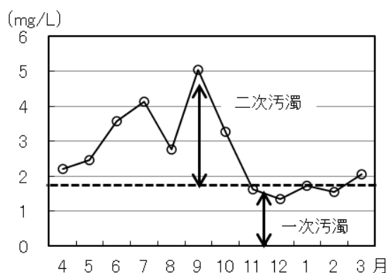
令和6年度 COD上層(A類型)の月変化
