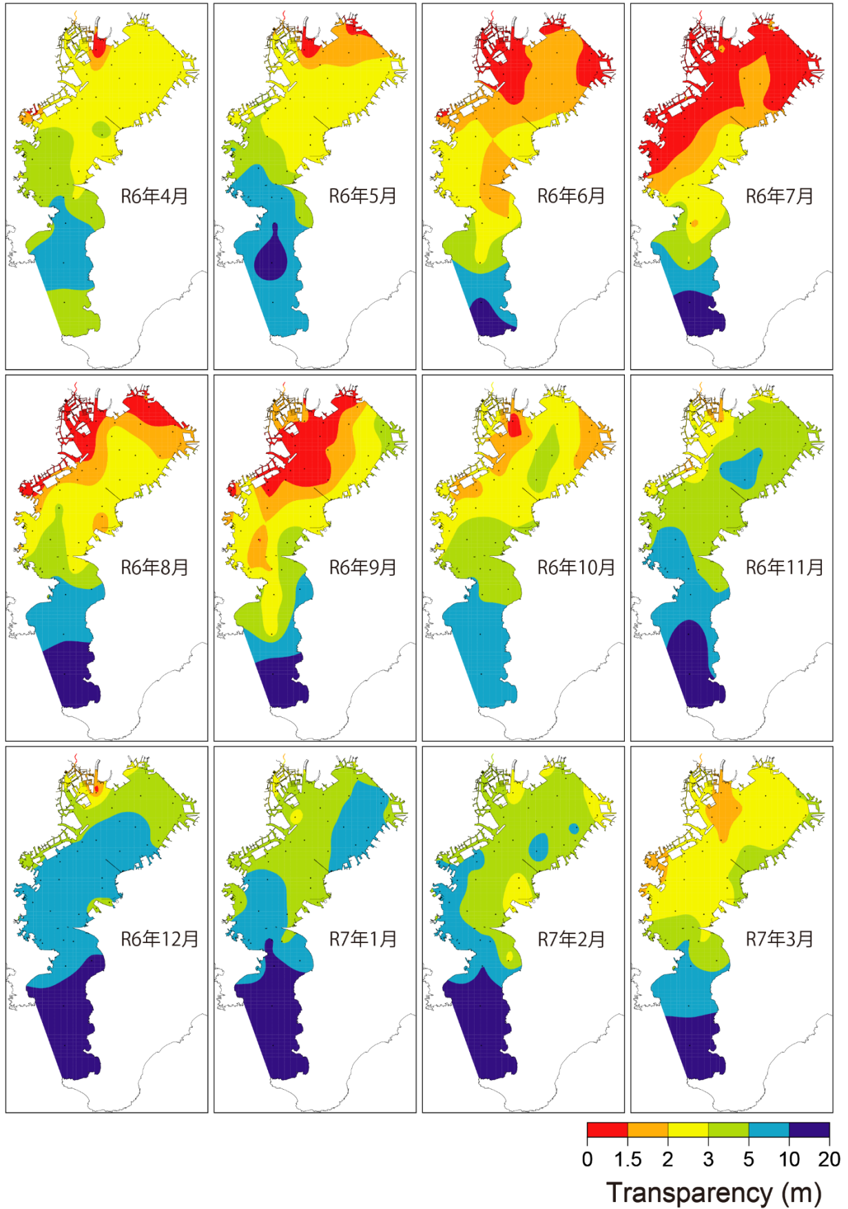
図 22-3 透明度の月別水平分布
