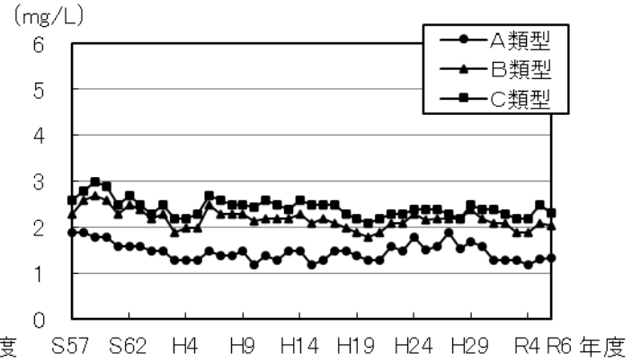
図 3-2 下層 COD の類型別経年変化
