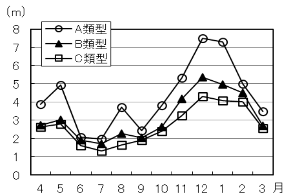
図 12 透明度の月変化
