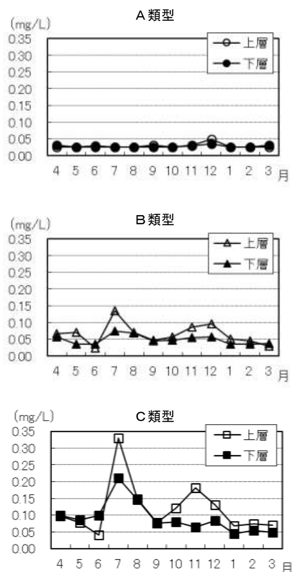
図 16 アンモニア性窒素の変化
