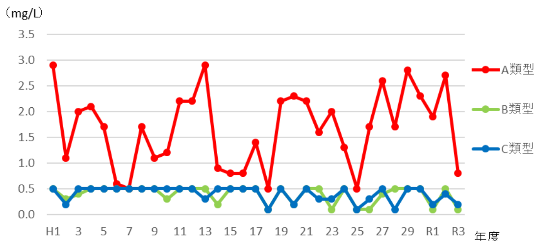
図6 下層 DO 最小値の推移
