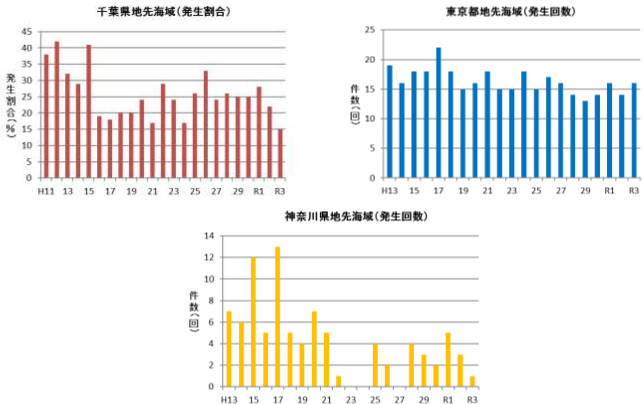
図 22-2 過去の赤潮発生状況
