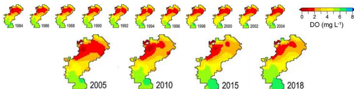
9月底層の DO 濃度分布の長期的推移
