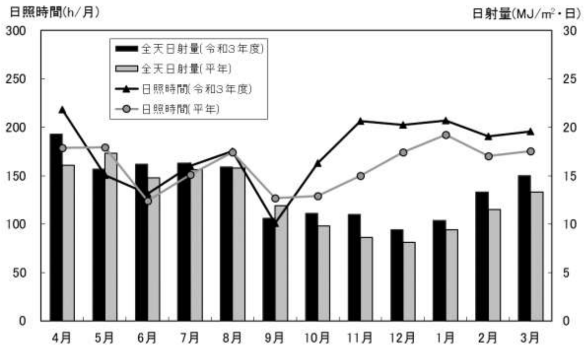
25-2 全天日射量及び日照時間の月変化(令和3年度と平年 (※) との比較)
