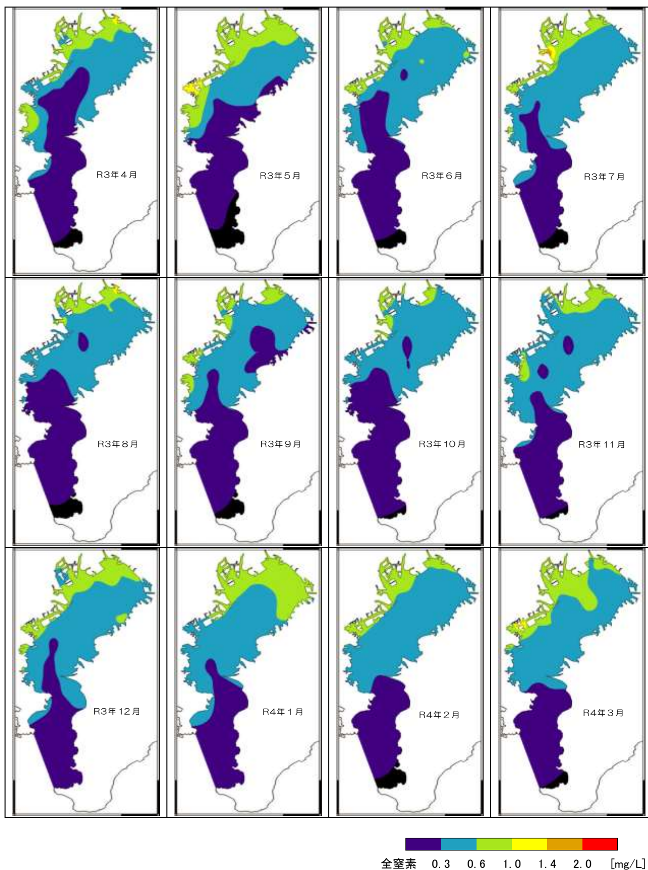
図 21－8 全窒素(下層)の月別水平分布
