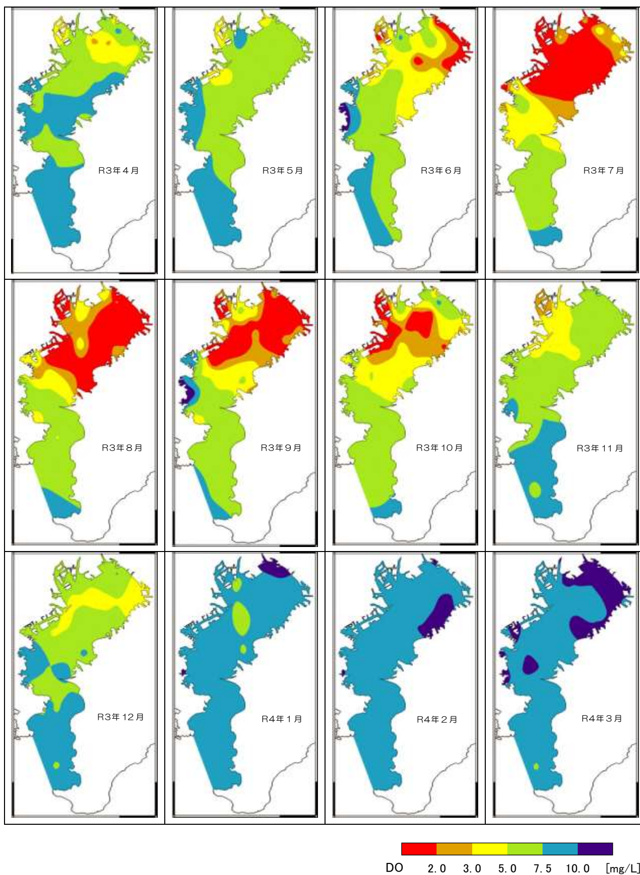
図 21-5 溶存酸素量(DO)(下層)の月別水平分布
