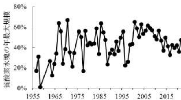
図3 貧酸素水塊の年最大規模の経年変化
