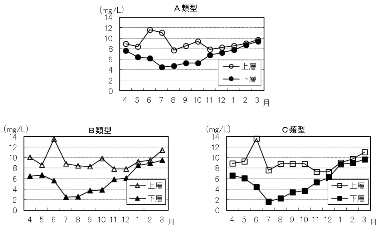
図 12 溶存酸素量(DO)の月変化
