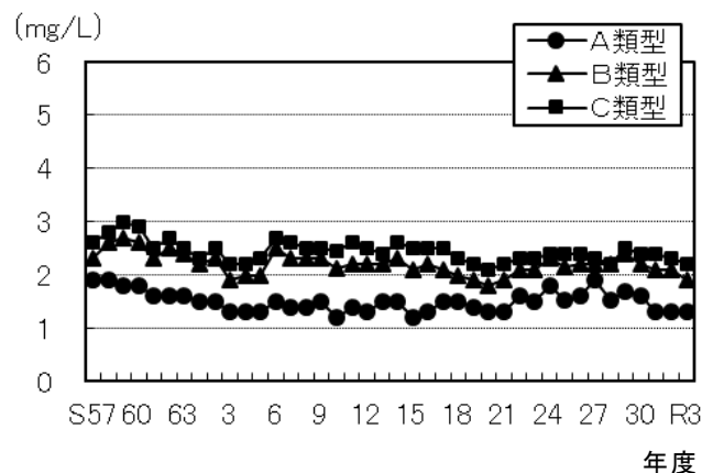
図 3-2 下層 COD の類型別経年変化
