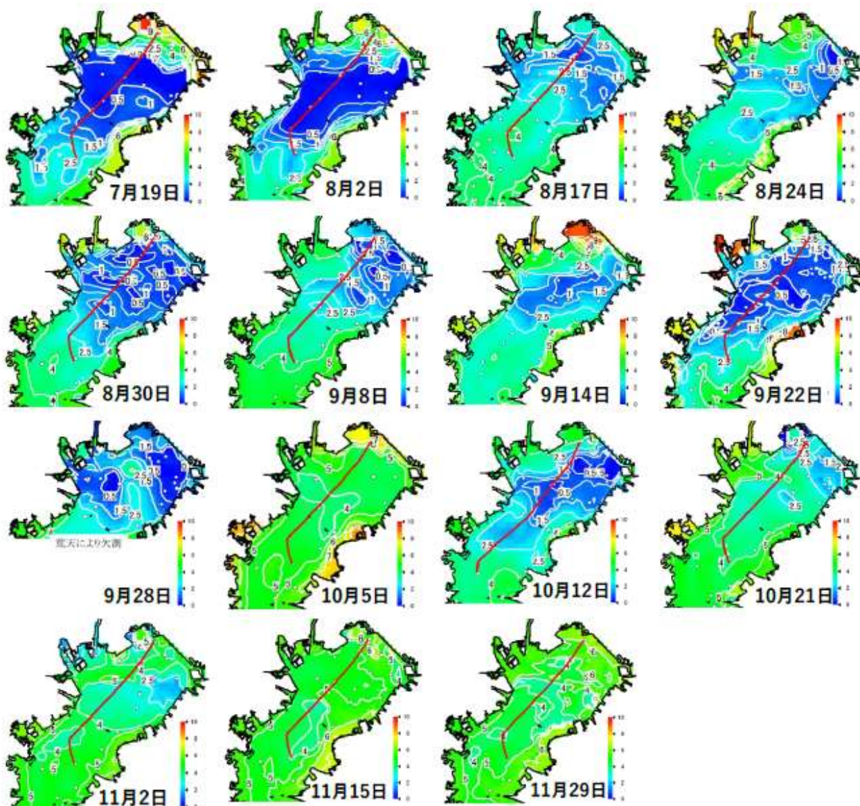
図1 底層の溶存酸素量分布（続き）
