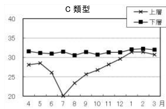
図9 塩分の月変化
