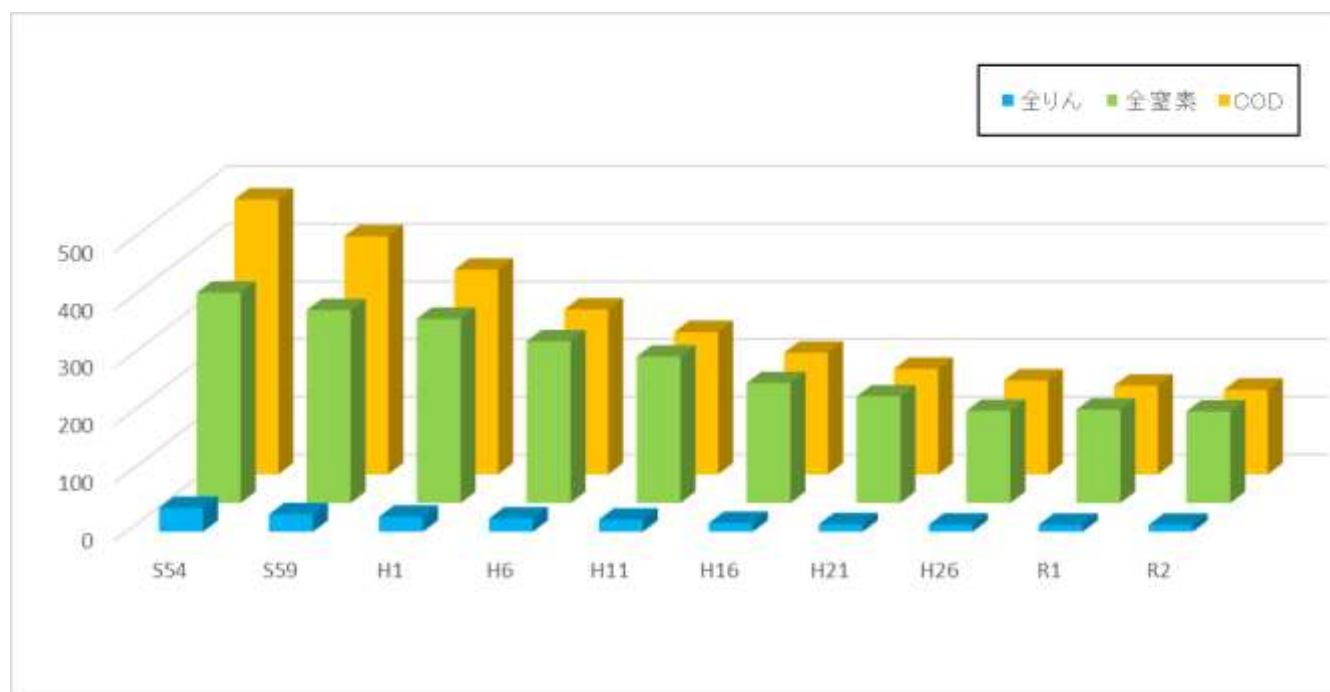
図 24-1 東京湾への汚濁負荷量の経年変化
