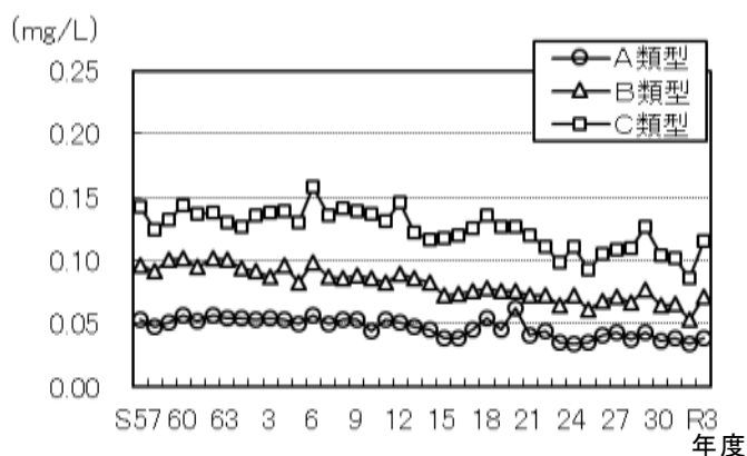
図 5-1 上層全りんの類型別経年変化
