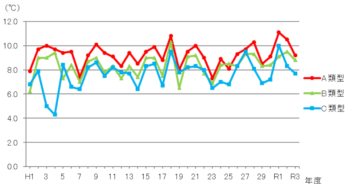
図7 水温（上層）最小値の経年変化
