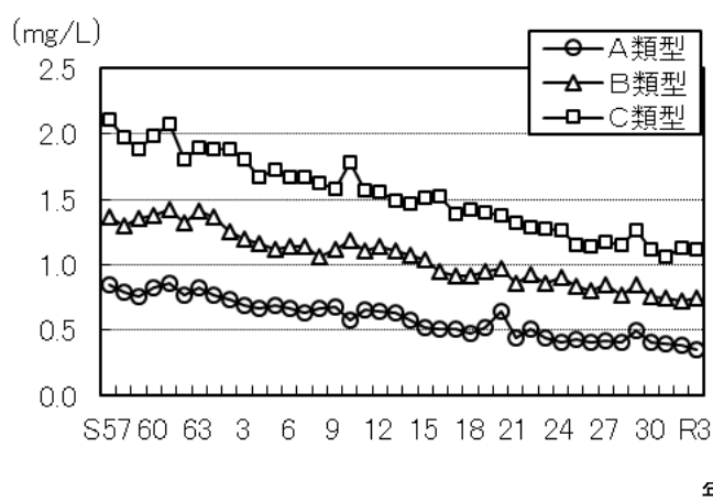
図 4-1 上層全窒素の類型別経年変化
