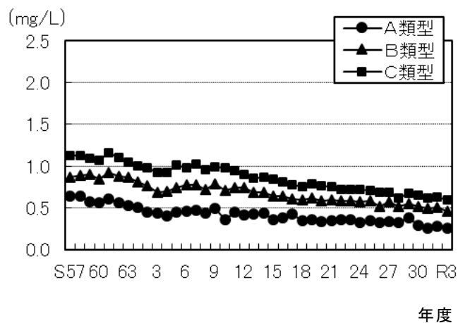
図 4-2 下層全窒素の類型別経年変化
