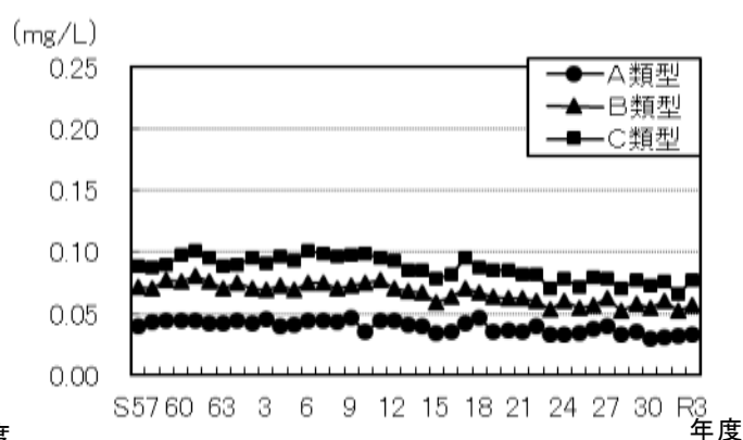
図 5-2 下層全りんの類型別経年変化
