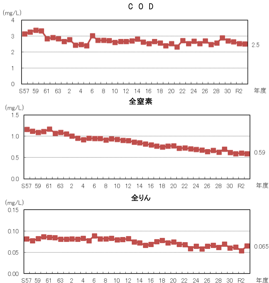
図 2 湾代表値（全層）の経年変化
