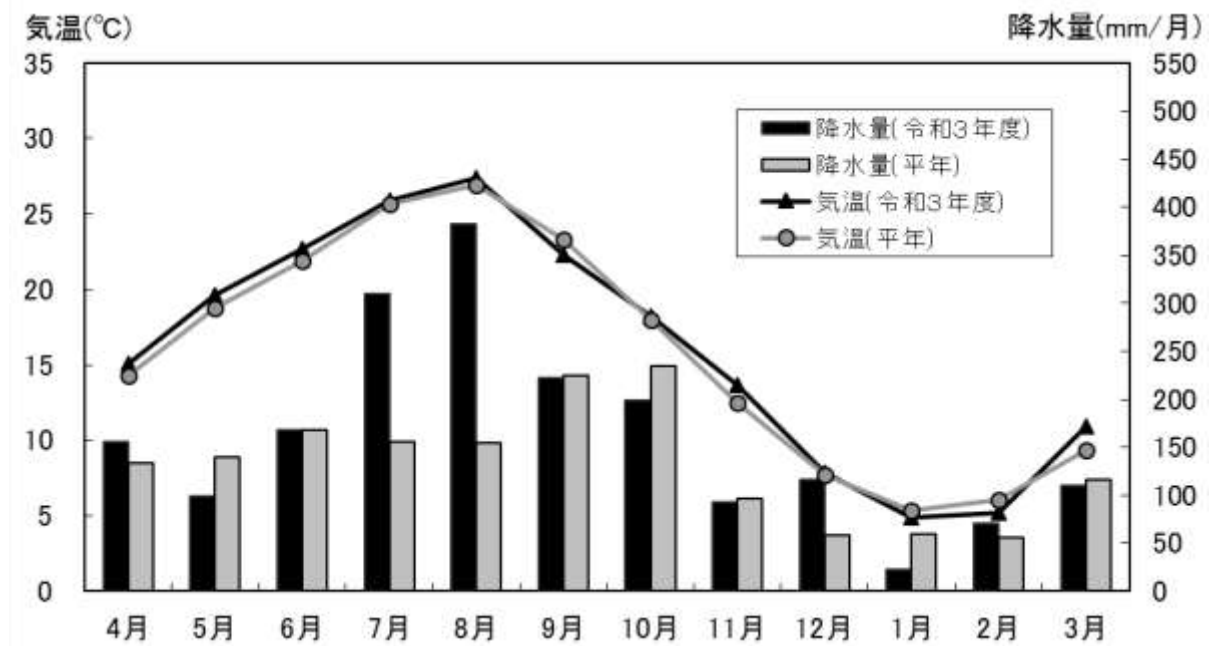
図 25-1 降雨量及び気温の月変化(令和3年度と平年 (※) との比較)
