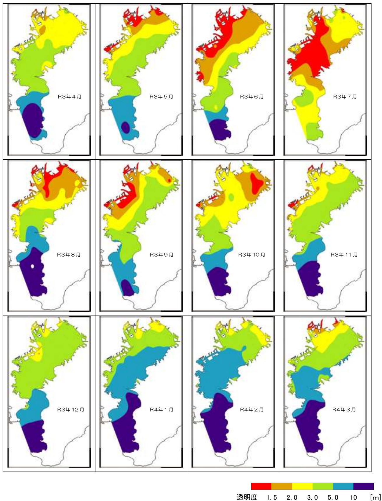
図 21-3 透明度の月別水平分布
