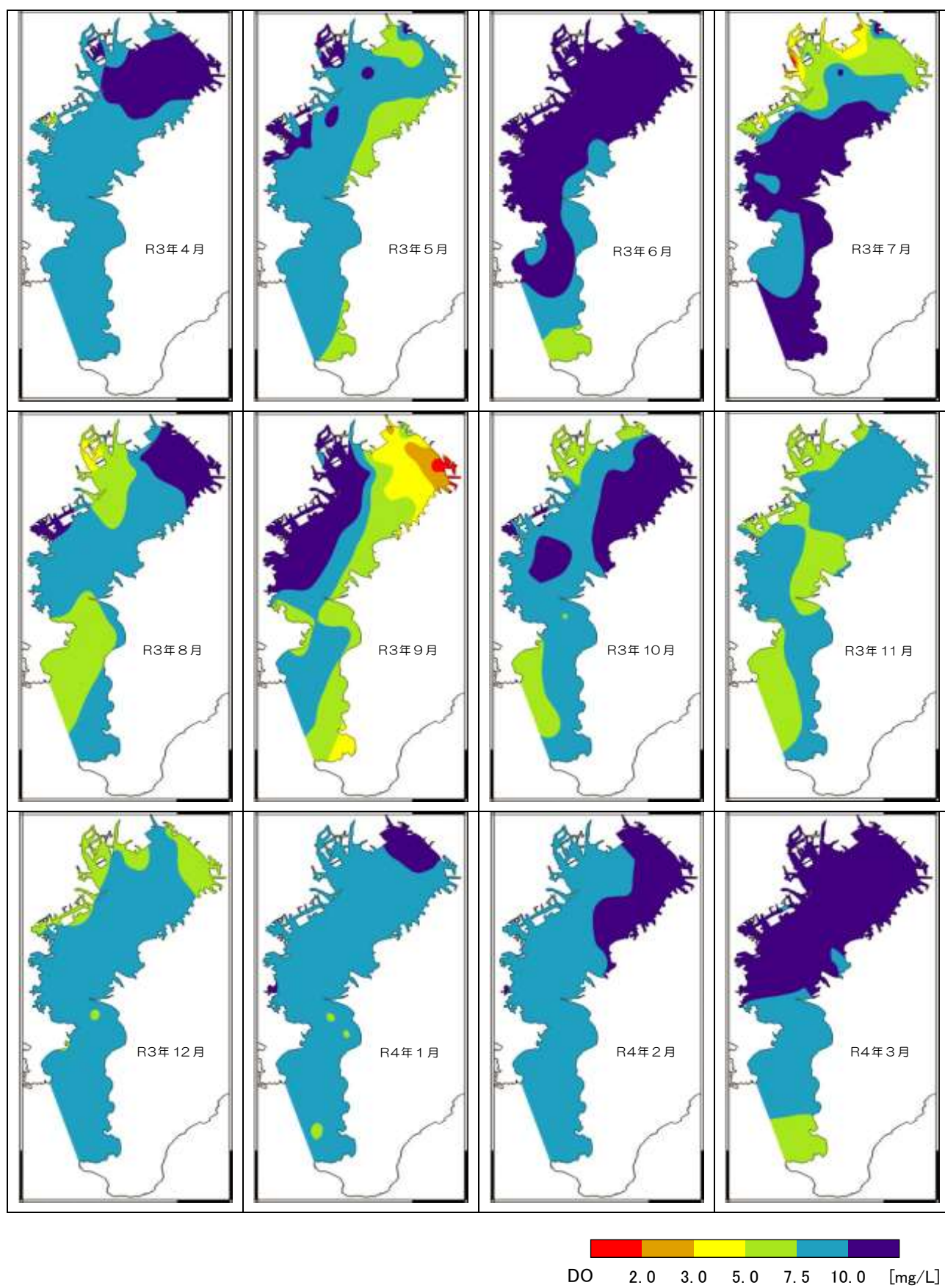
図 21-4 溶存酸素量(DO)(上層)の月別水平分布
