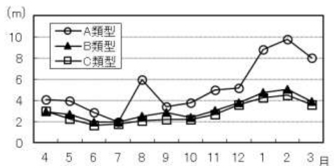
図 11 透明度の月変化
