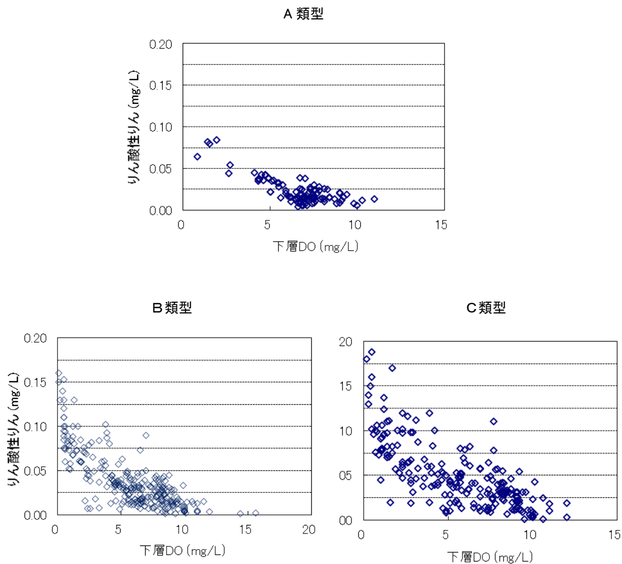
類型別下層 DO と下層りん酸性りんの関係(令和3年度)
