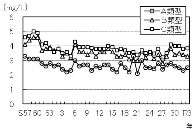
図 3-1 上層 COD の類型別経年変化
