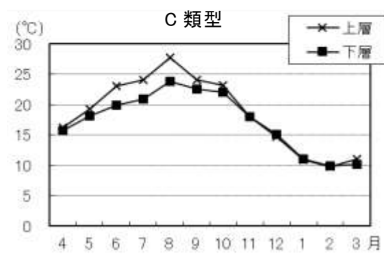
図8 水温の月変化
