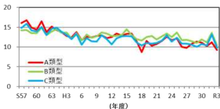
図 20 全窒素／全りん比の経年変化
