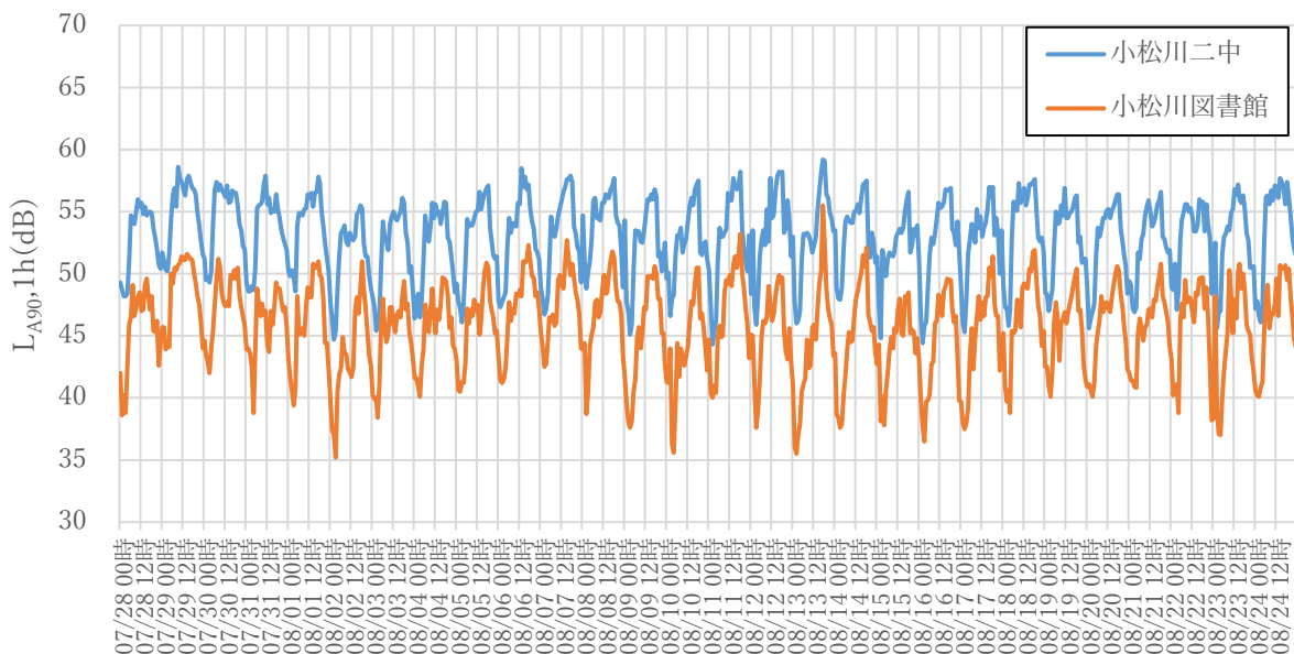
図2 環境騒音 ( L_{A90, 1時間} ) 比較
