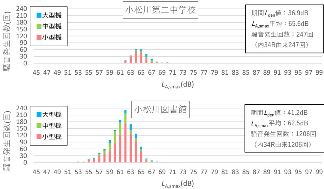
図1 最大騒音レベル別・機種(大中小)別騒音発生回数比較
