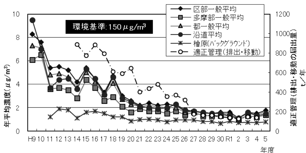
図5-5 ジクロロメタンの経年変化
