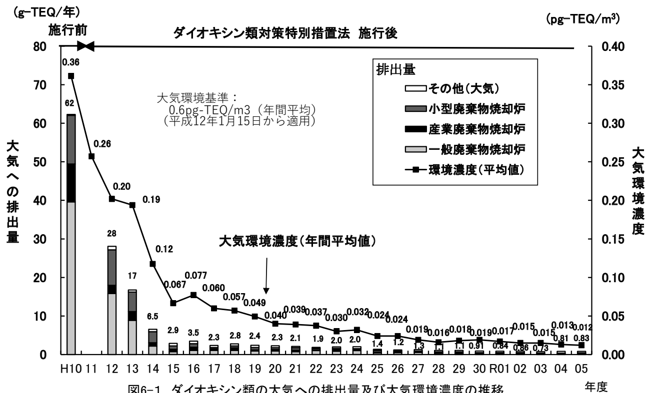
図6-1 ダイオキシン類の大気への排出量及び大気環境濃度の推移
