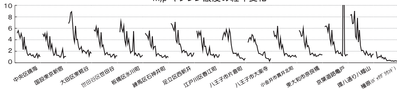
m,p-キシレン濃度の経年変化
