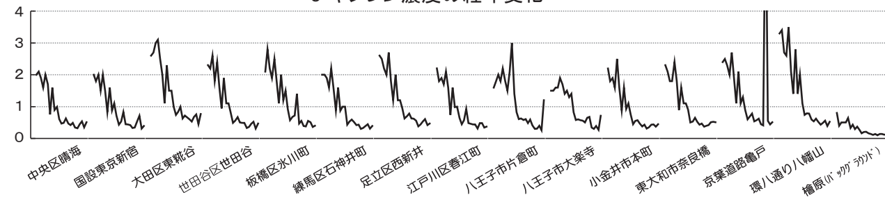
o-キシレン濃度の経年変化
