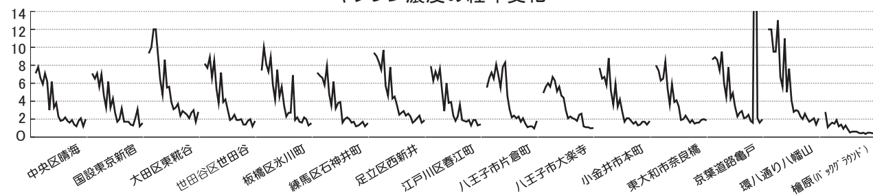
キシレン濃度の経年変化
