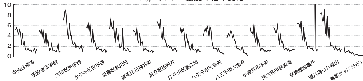
m,p-キシレン濃度の経年変化
