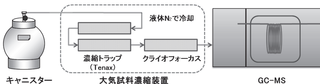
図 2 大気試料濃縮-GC/MS 装置
