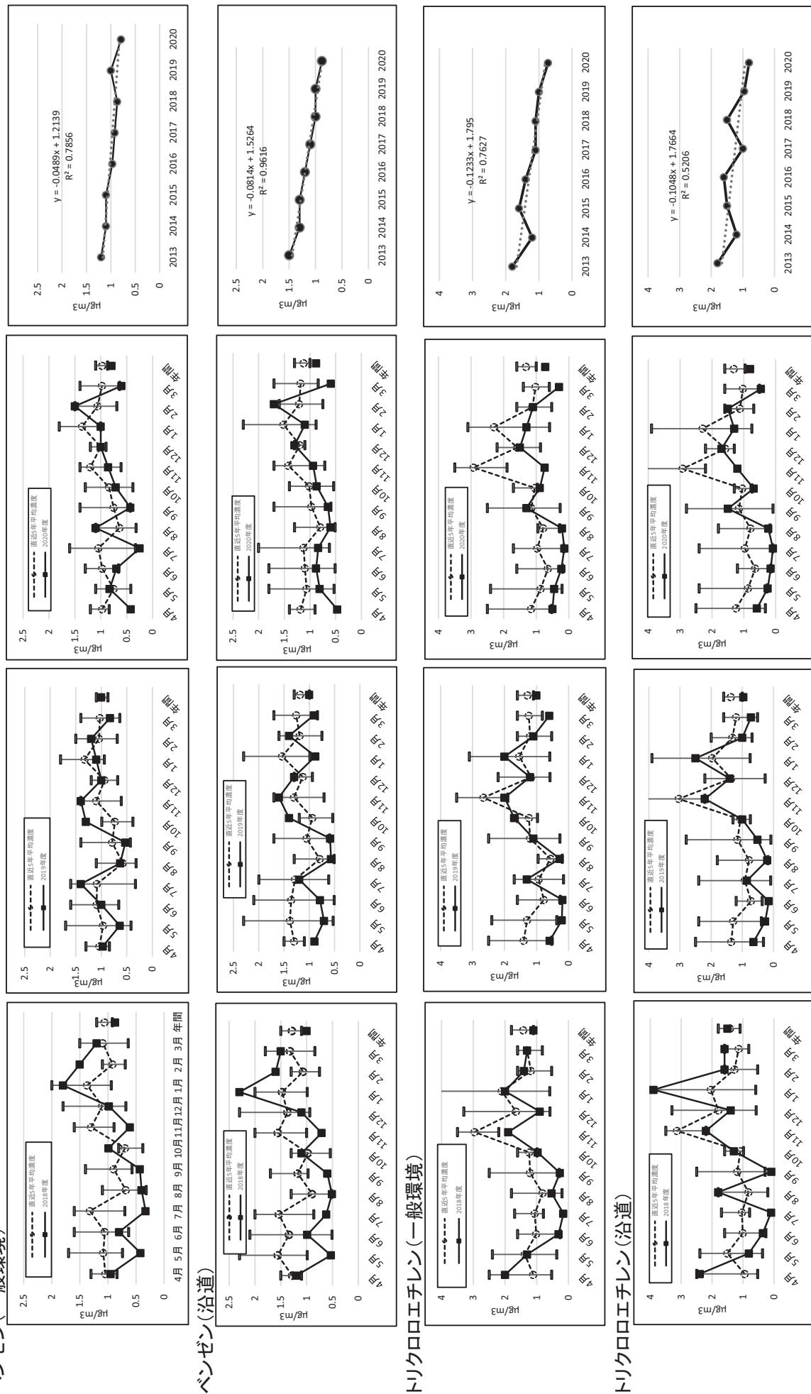
図5-7 各年度の経月変化及び経年変化 ベンゼン(一般環境)
