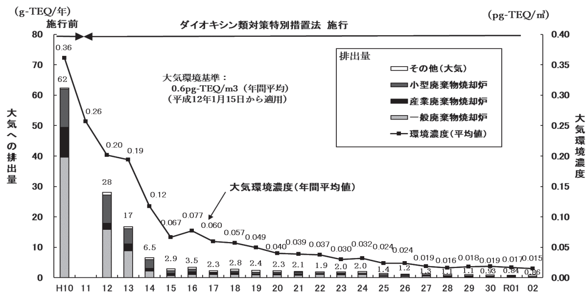
図 6-1 ダイオキシン類の大気への排出量及び大気環境濃度の推移
