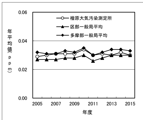
図9-9 光化学オキシダント年平均値の経年変化
