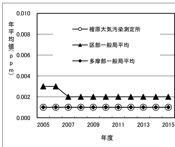
図9-10 二酸化硫黄年平均値の経年変化
