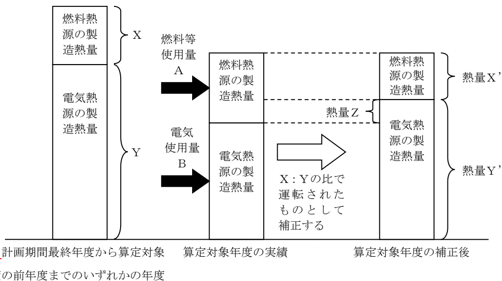
図2：算定対象年度に電気熱源の使用がある場合の排出量等の補正方法
