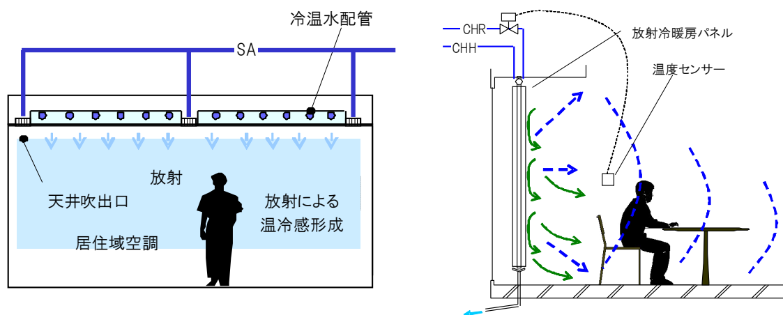
天井放射冷暖房空調システムの例
