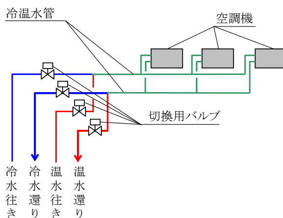
冷水・温水配管と切換用バルブ
