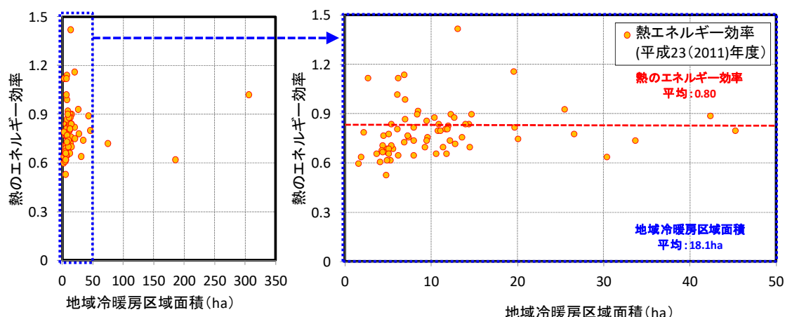
平成 23 年度までの対象事業所における熱エネルギー効率の分布
