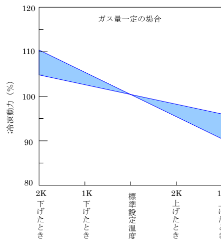
冷却水入口温度を変化させた場合の冷凍能力の変化（ガス焚冷温水発生機）
