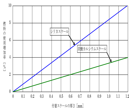
スケール付着と燃料増加率
