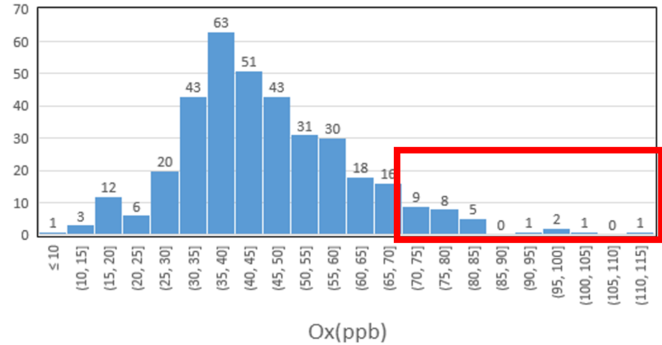
武蔵野市関前の日最高8時間値のヒストグラム（2023年度）
