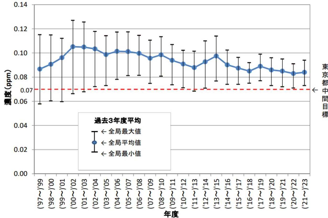
年間4番目に高い日最高8時間値の3年平均の経年変化（再掲）
