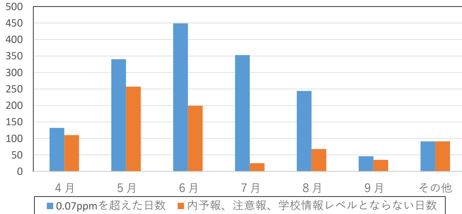
日最高8時間値が0.07ppmを超えた延べ日数（2021年度-2023年度、月別）
