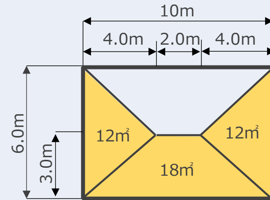
屋根伏図
