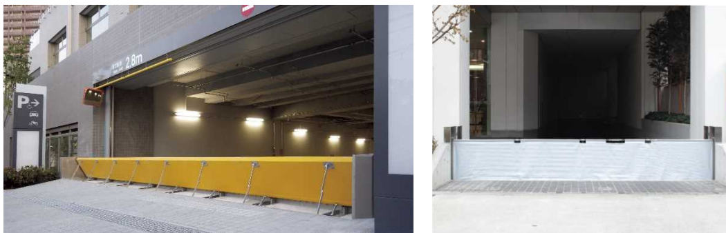
起伏式止水板、シート式止水板の例
