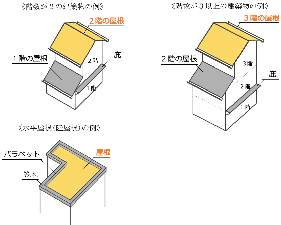
【図10 対象となる屋根のイメージ】
