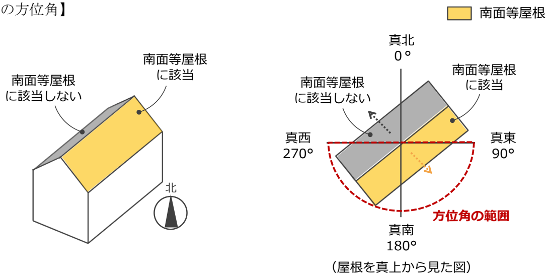
【図11 屋根の方位角】
