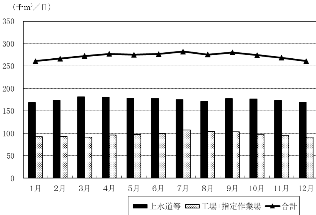
図2 月別地下水揚水量
