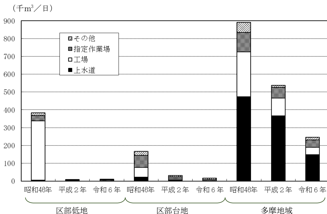
図 4 昭和 46 年、平成 2 年、令和 6 年における地下水揚水量
