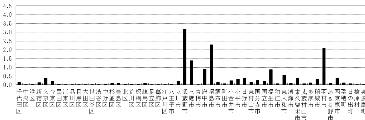
図3 区市町村別単位面積当たりの揚水量
