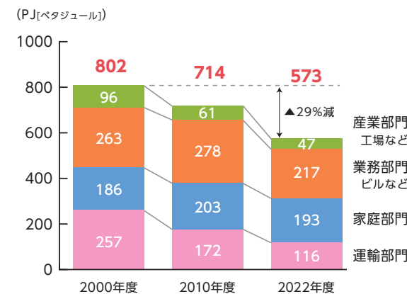
都のエネルギー消費状況
