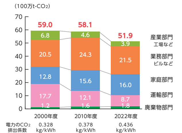
都の二酸化炭素排出状況
