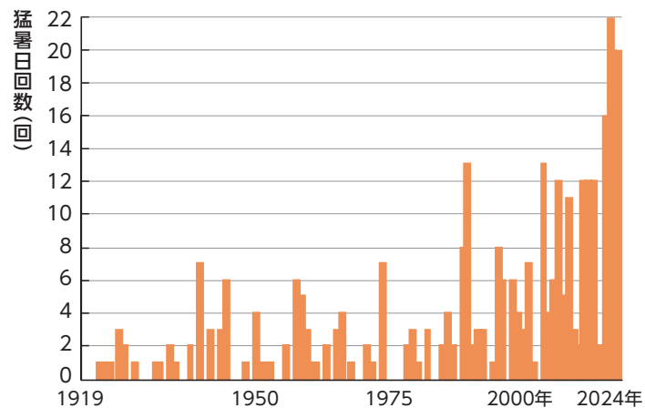
東京管区气象台での猛暑日回数
