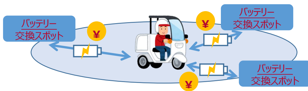
BaaS の一例
