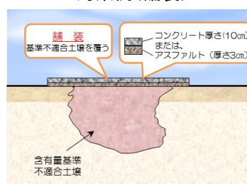
対策例(舗装)
