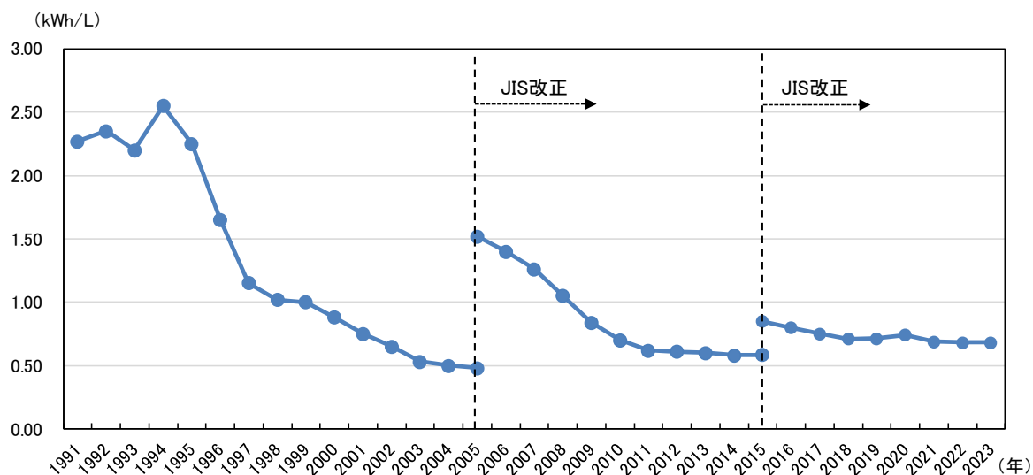
図 2-28 電気冷蔵庫の省エネルギーの進展状況
