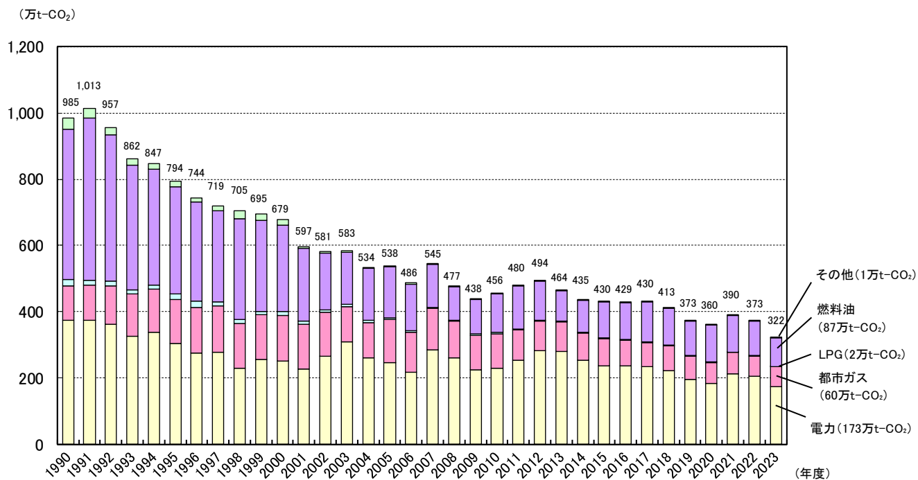
図 3-13 産業部門の二酸化炭素排出量の推移
