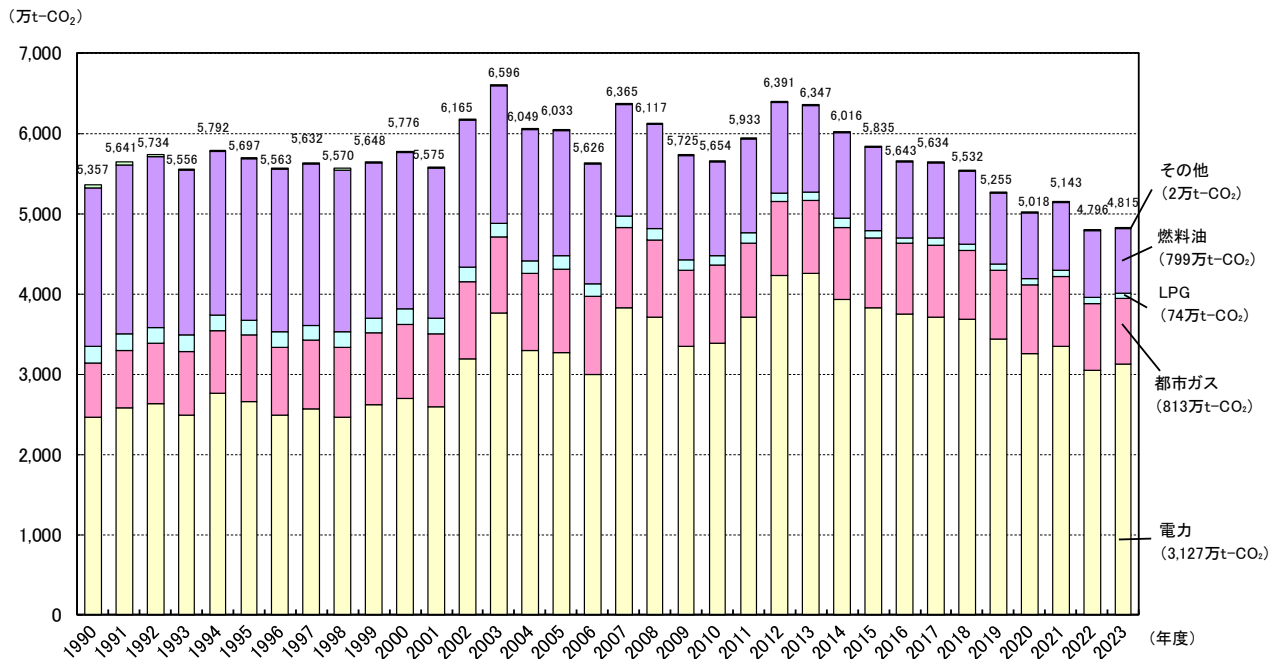
図 3-11 東京都におけるエネルギー起源 CO 2 排出量（燃料種別）の推移
