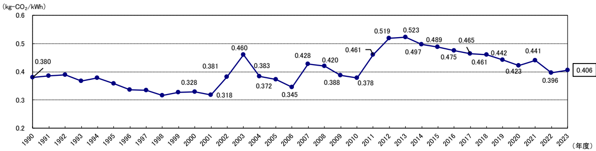
図 3-1 電力の二酸化炭素排出係数の推移
