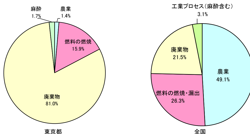
図 3-20 東京都と全国の一酸化二窒素排出構成比（2023 年度）
