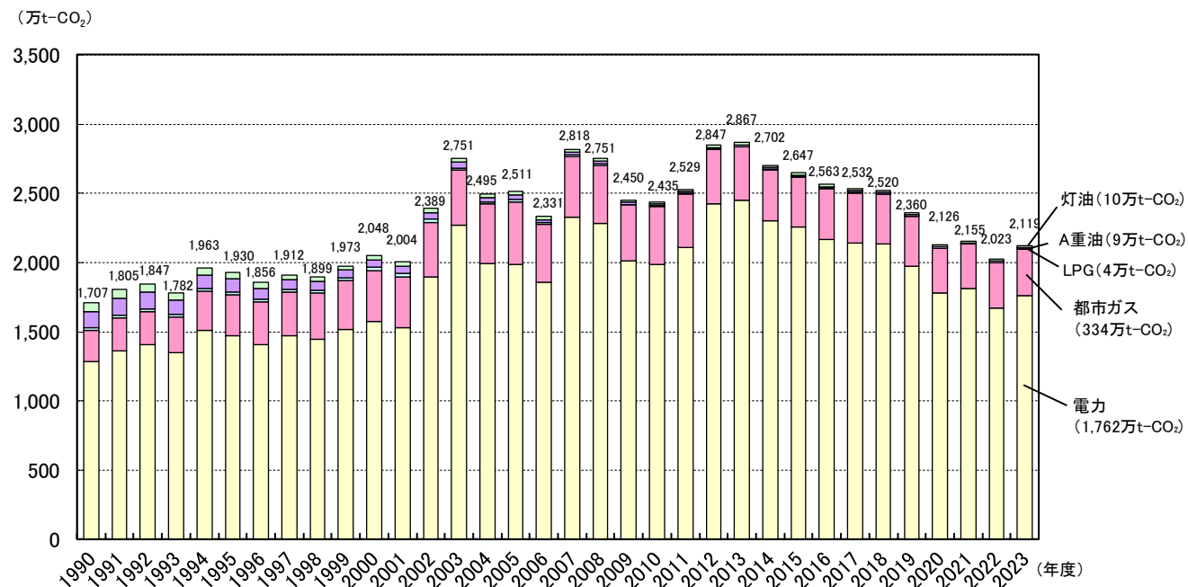
図 3-14 業務部門の二酸化炭素排出量の推移
