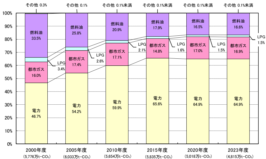
図 3-12 東京都におけるエネルギー起源 CO 2 排出量（燃料種別）の構成比
