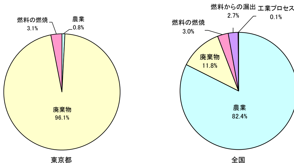
図 3-19 東京都と全国のメタン排出構成比（2023 年度）
