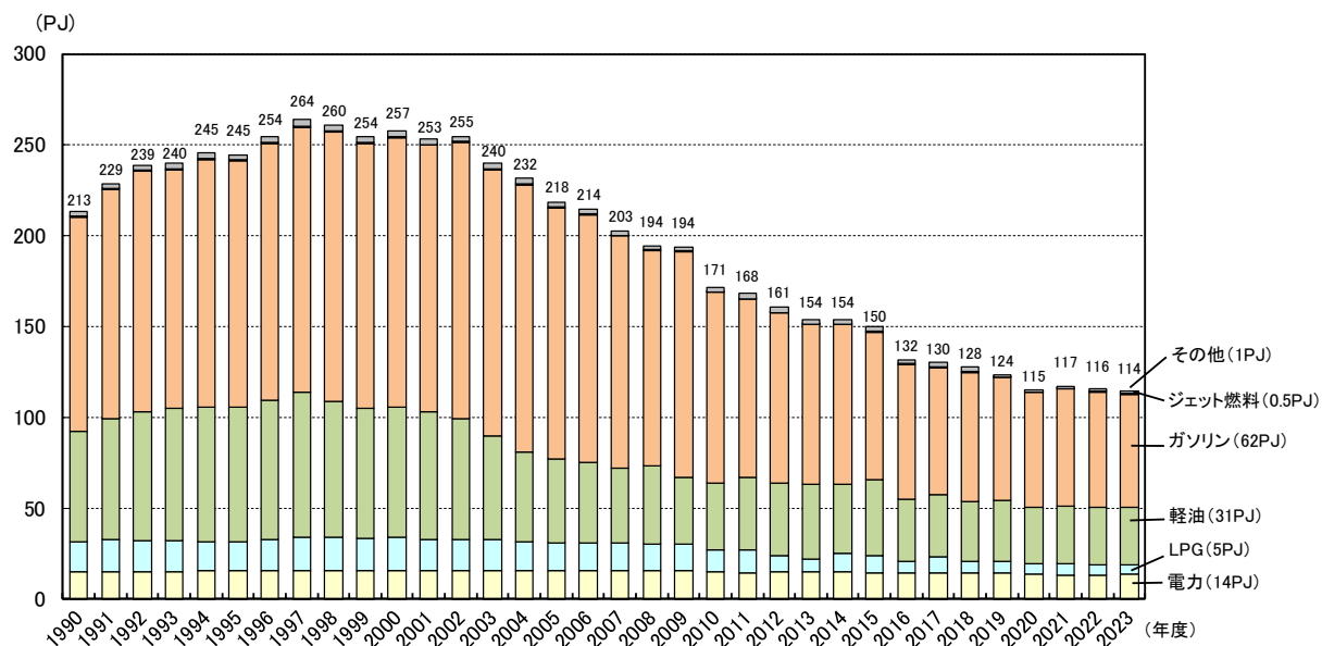
図 2-31 運輸部門の最終エネルギー消費（燃料種別）の推移
