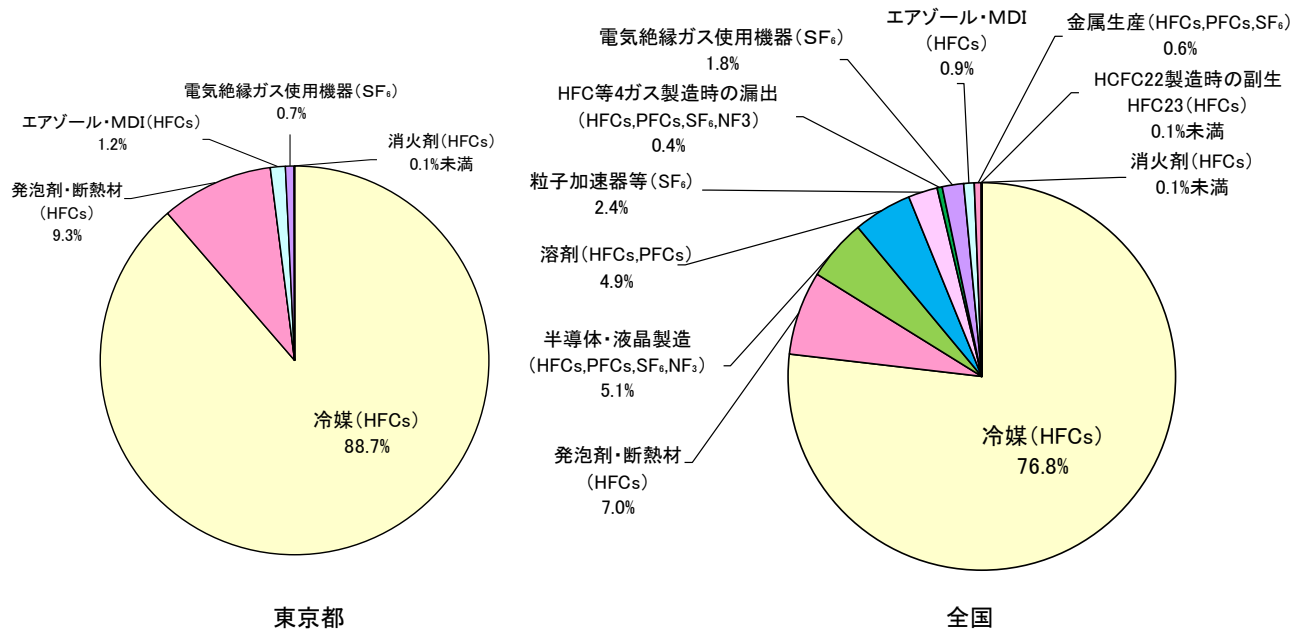
図 3-21 東京都と全国の HFC 等 4 ガス排出構成比 (2023 年度)
