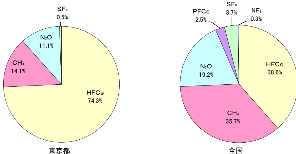
図 3-18 東京都と全国のその他の温室効果ガス排出構成比 (2023 年度)
