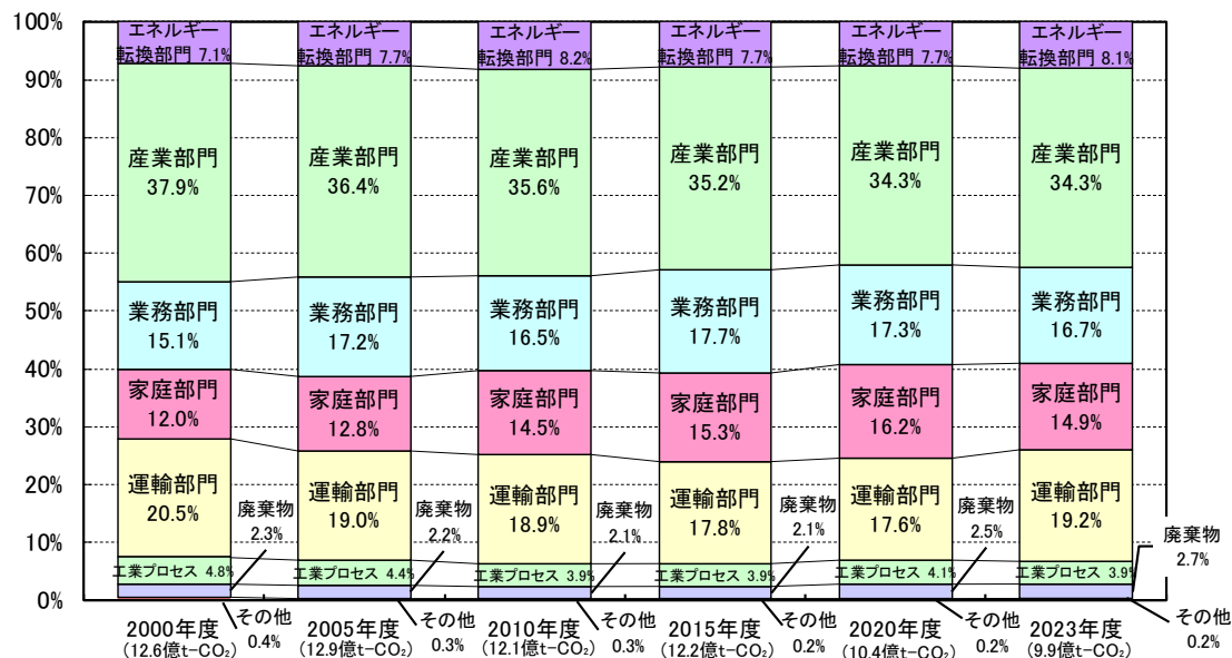
図 3-10 全国における二酸化炭素排出量の構成比
