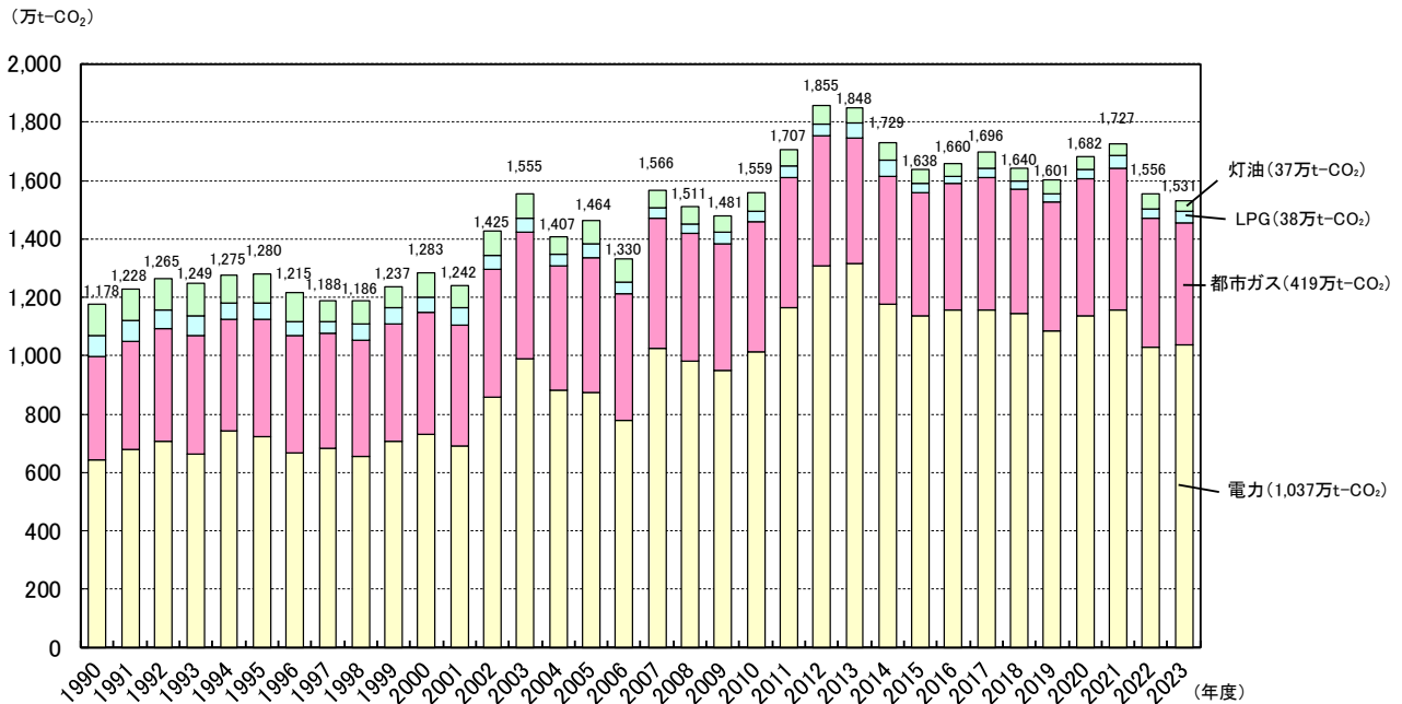
図 3-15 家庭部門の二酸化炭素排出量の推移
