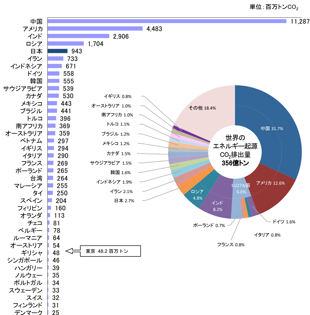
図 1-1 国別エネルギー起源 CO 2 排出量 (2023 年)
