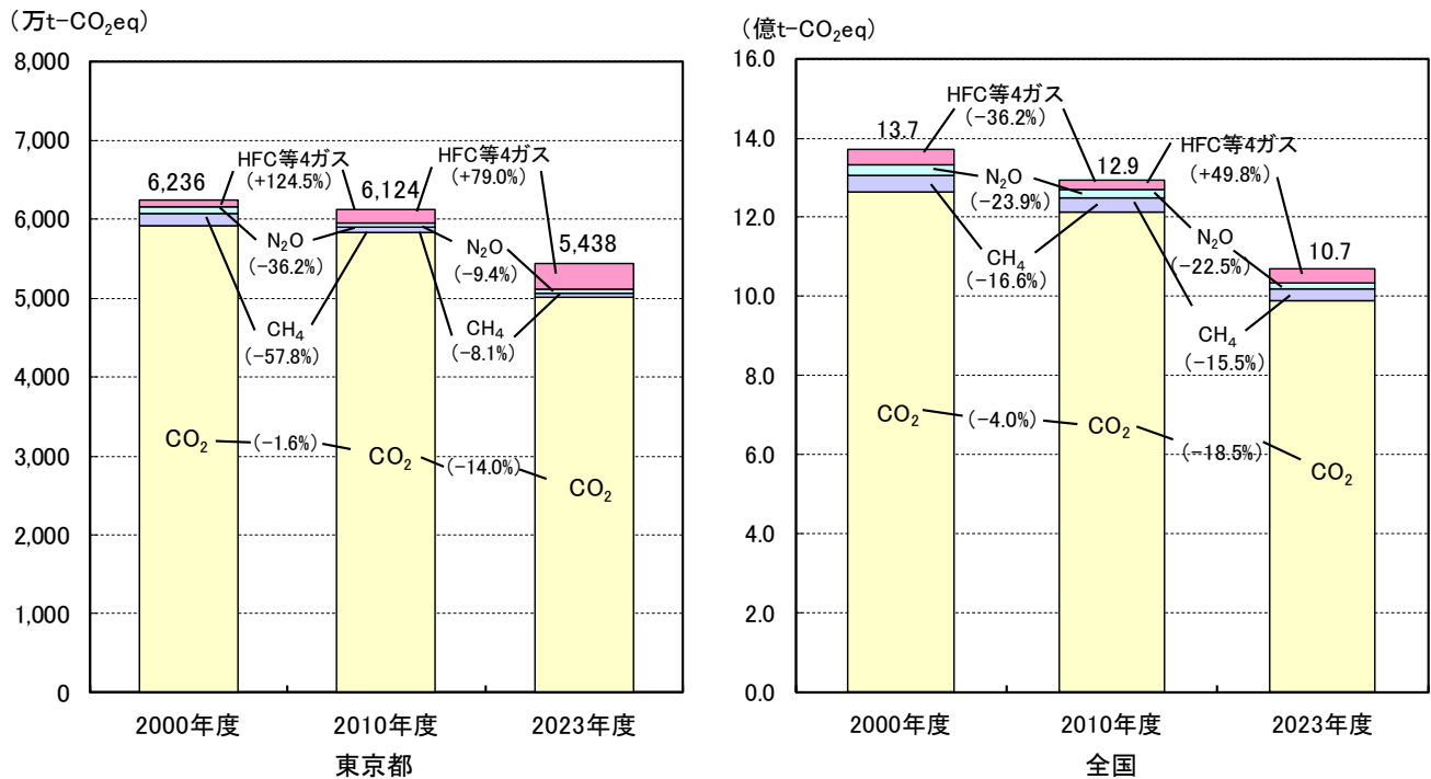
図 3-5 東京都と全国の温室効果ガス別排出量の推移
