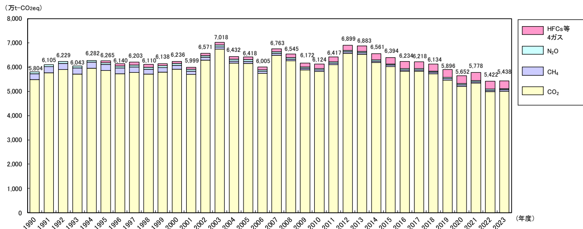
図 3-3 東京都における温室効果ガス総排出量の推移
