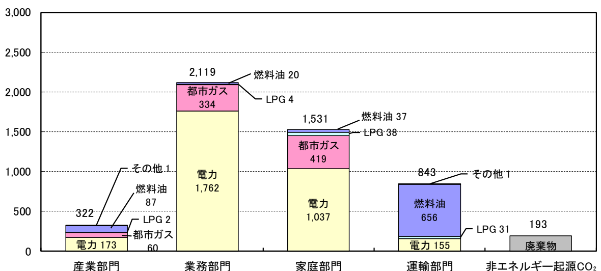
図 3-6 東京都における二酸化炭素排出量の部門別状況（2023 年度）
