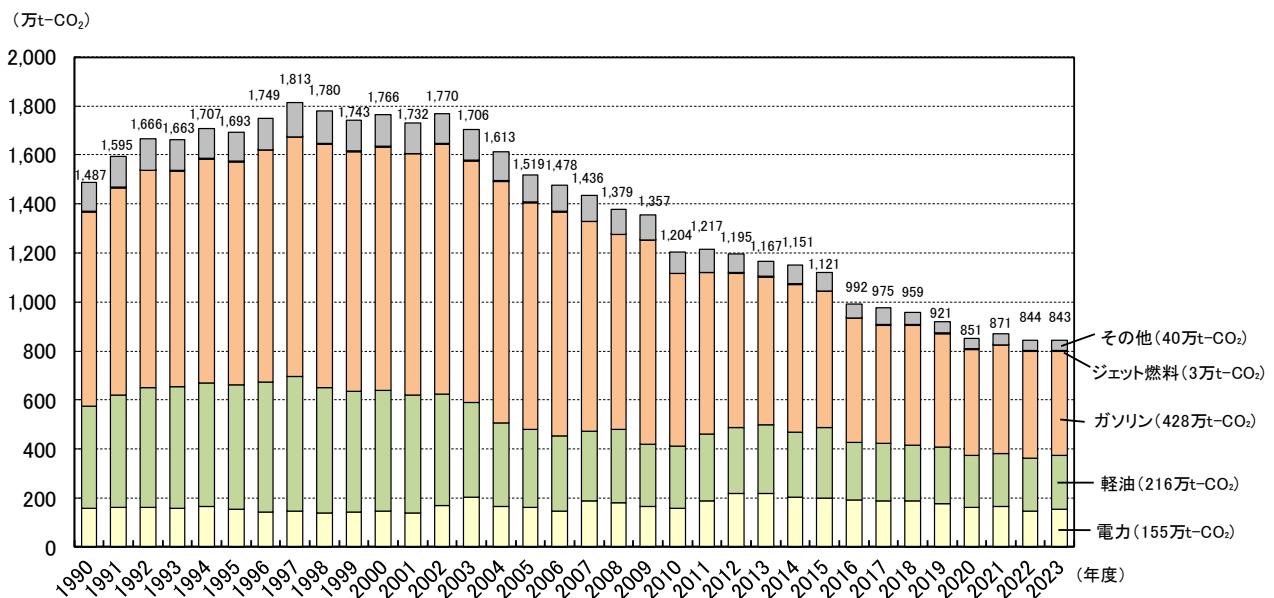
図 3-16 運輸部門の二酸化炭素排出量の推移
