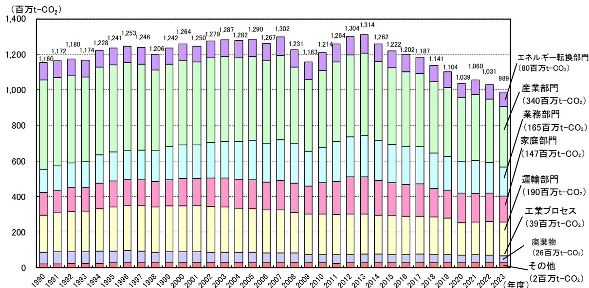
図 3-9 全国における二酸化炭素排出量の推移
