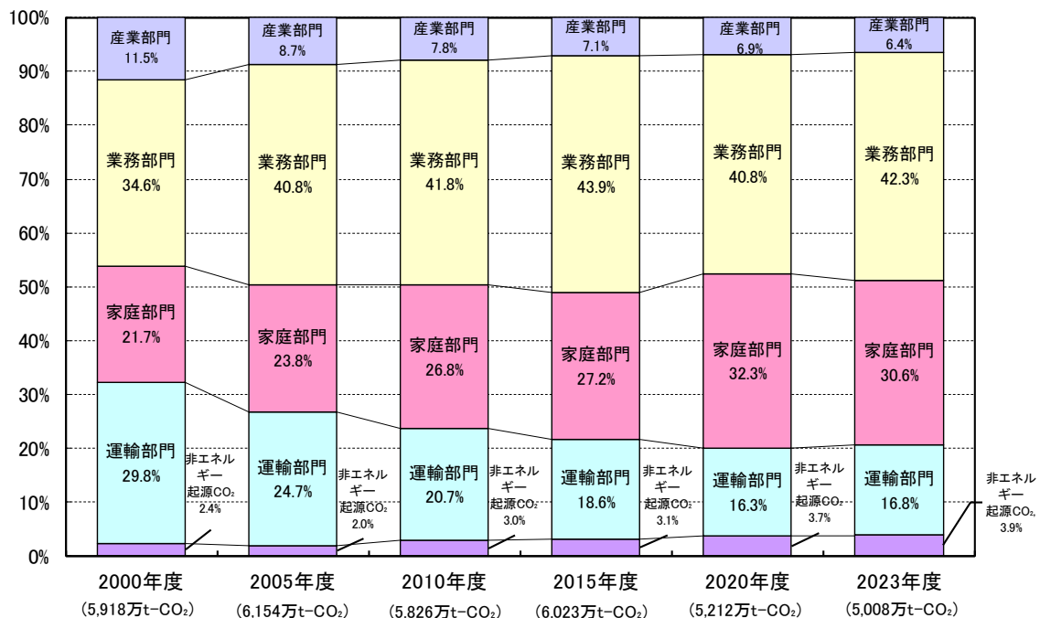
図 3-8 東京都における総 CO 2 排出量（部門別）の構成比
