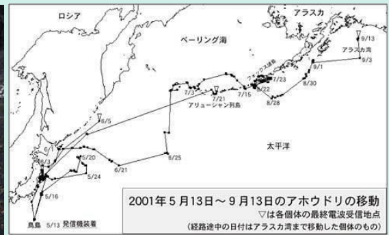
アホウドリの移動経路
