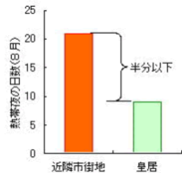
図-3 熱帯夜日数の違い(8月)
