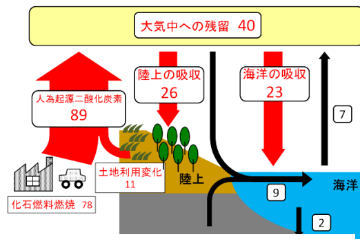
陸上と海洋の二酸化炭素の吸収模式図 49
