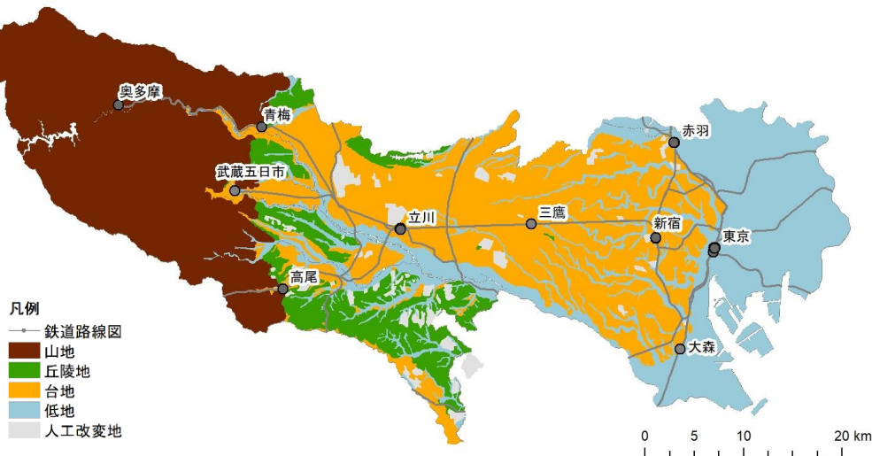
東京(本土部)の地形区分
