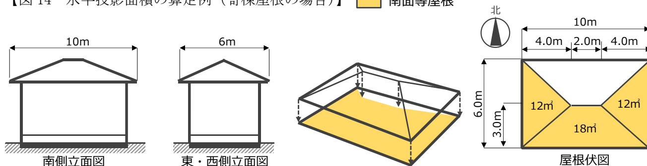
【図14 水平投影面積の算定例（寄棟屋根の場合）】 ■ 南面等屋根
