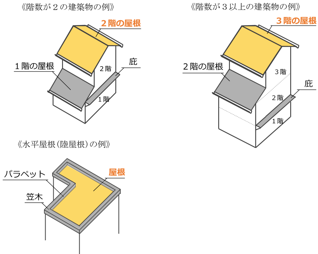
【図10 対象となる屋根のイメージ】 ■ 「屋根」に含むもの ■ 「屋根」に含まないもの
