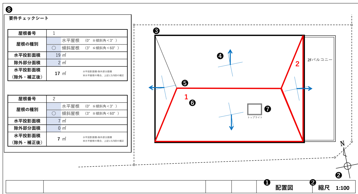
【図8 算定除外可能建築物への該当が確認できる図面（記載例）】
