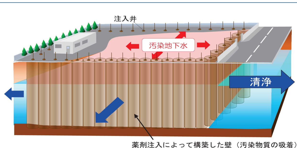
透過性地下水浄化壁の概要
