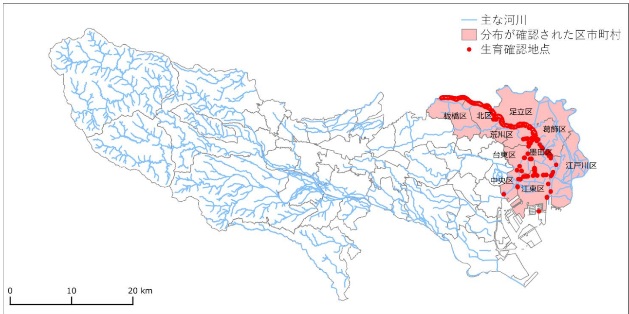
東京都内の分布状況 (2026年2月現在)
