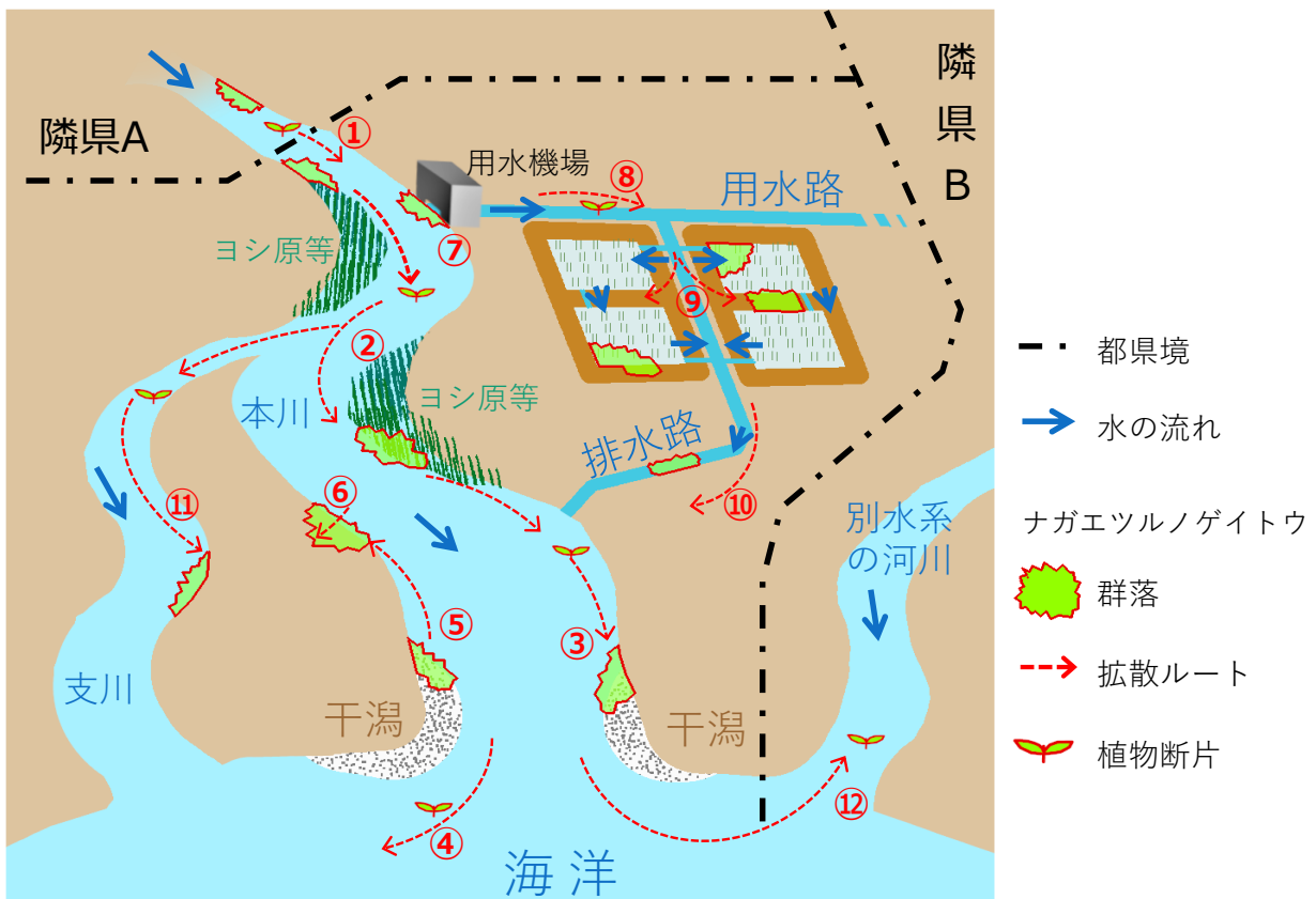
水の流れを通じた河川・水路・水田等での拡散経路の概念図
