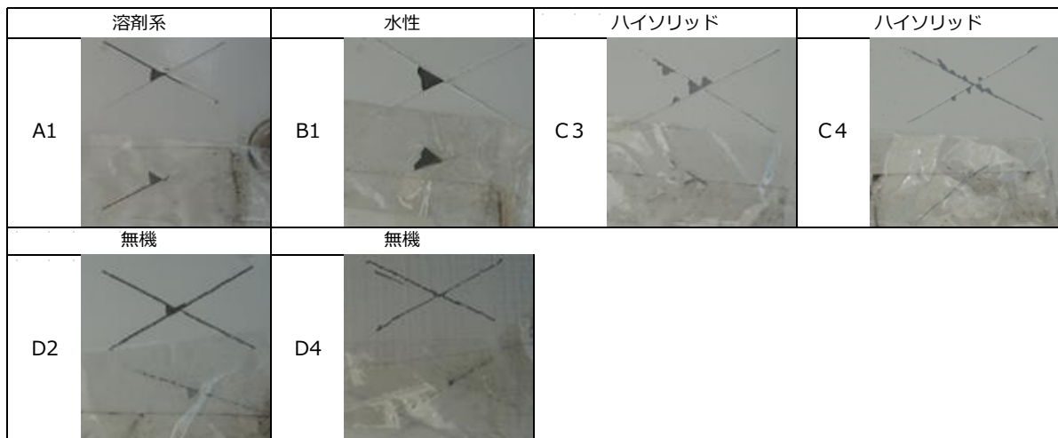
図3 付着性試験結果
