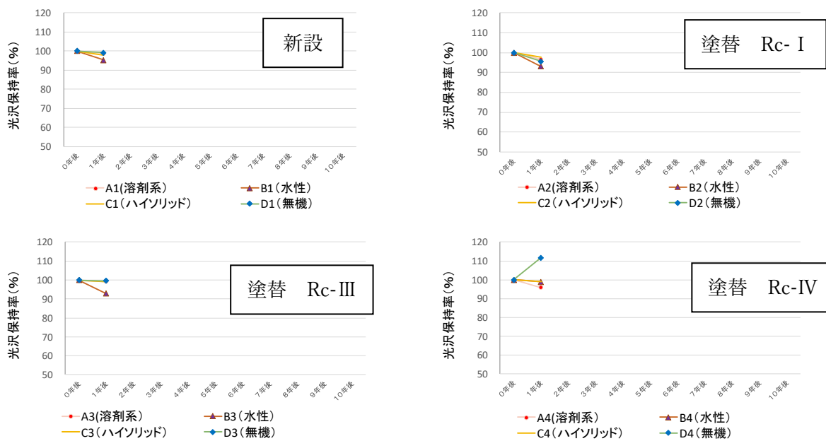
図4 光沢保持率
