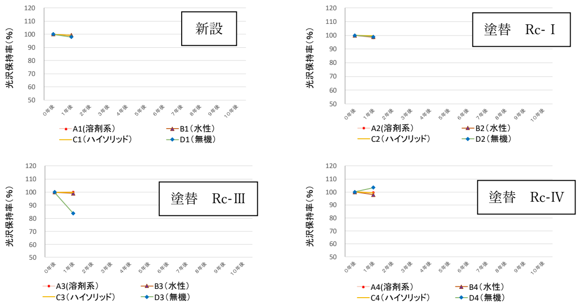
図2 光沢保持率
